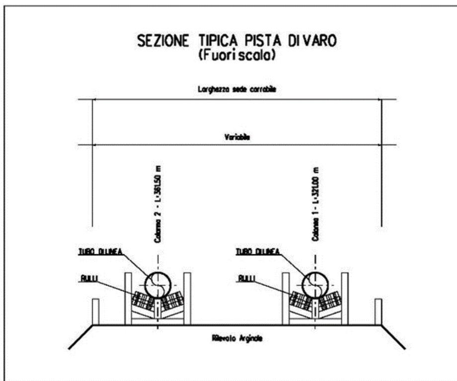
Fig. 7.1/H: Sezione della pista di varo (area in corrispondenza del sedime carrabile)
