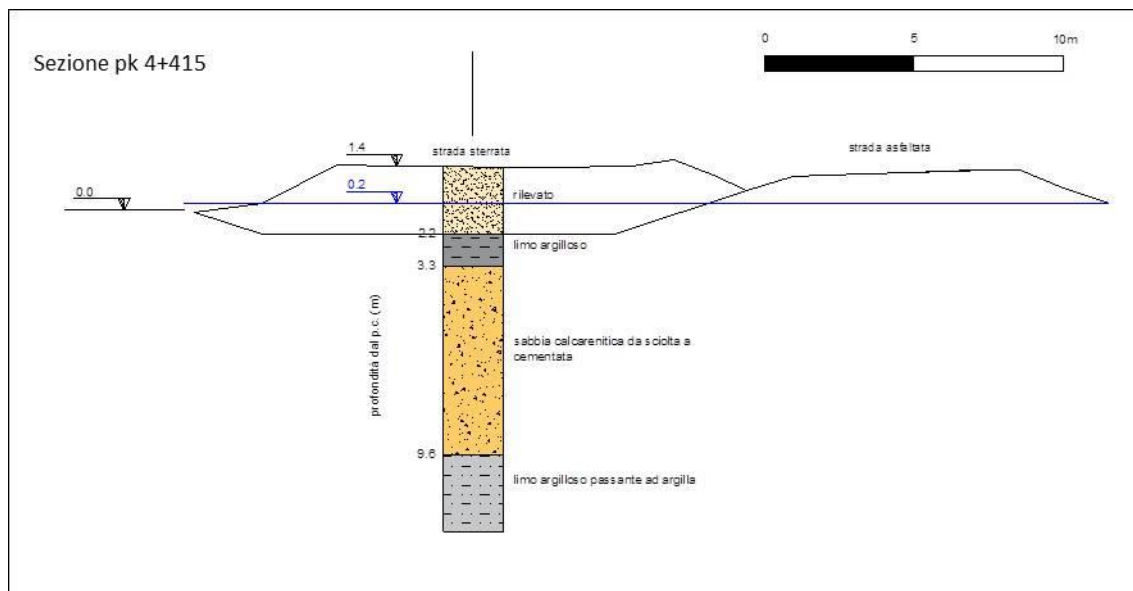
Fig. 7.1/C: Sezione trasversale km 4+415
