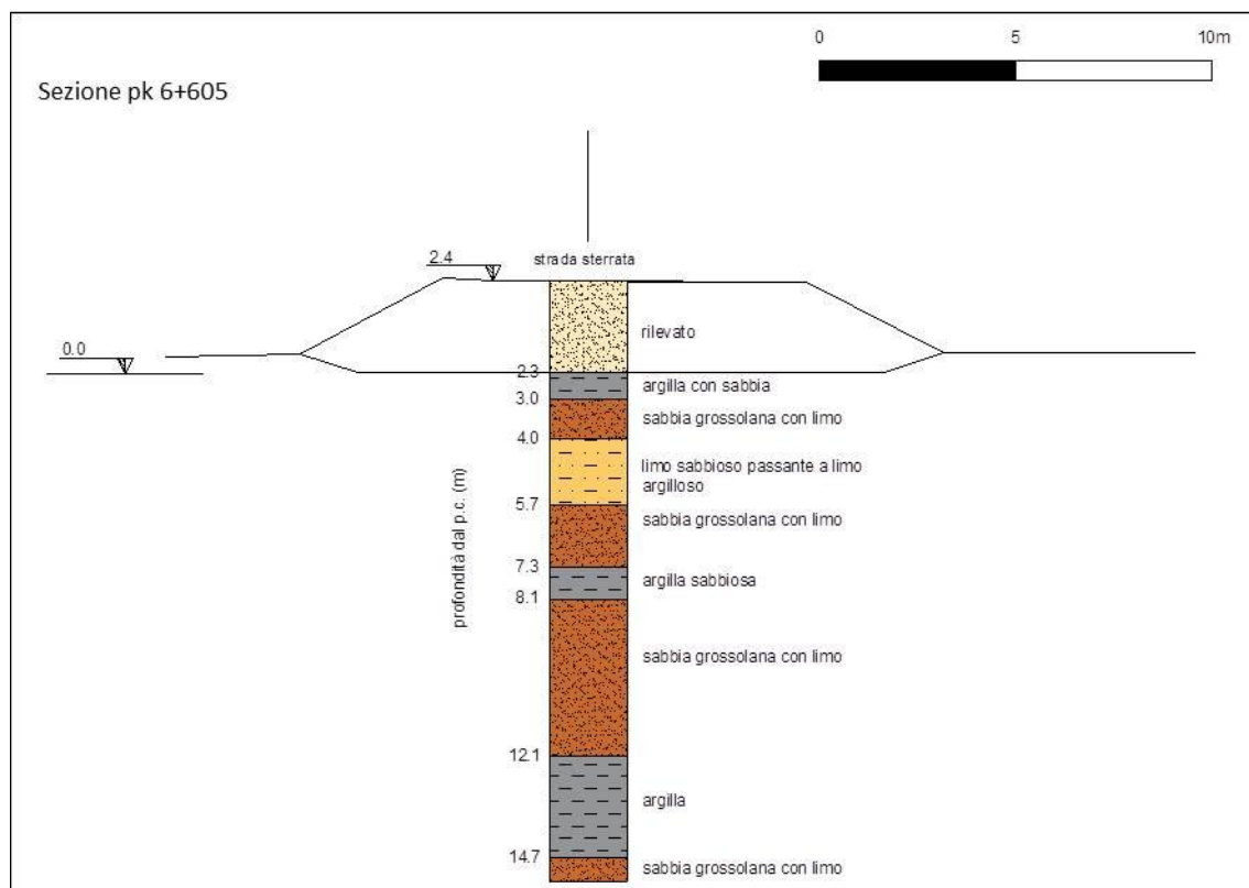
Fig. 7.1/G: Sezione trasversale km 6+605
