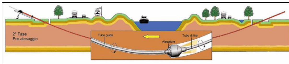
Fig. 7.1/J: Alesaggio del foro
