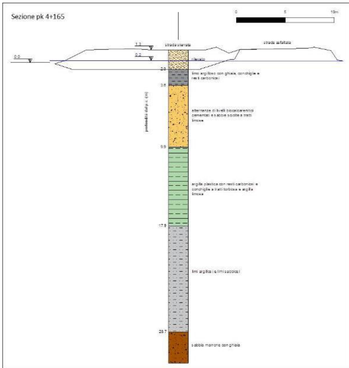
Fig. 7.1/B: Sezione trasversale km 4+165
