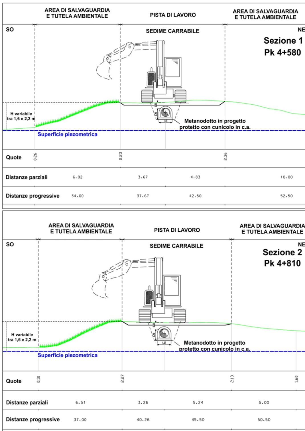
Fig. 7.1/F: Sezioni trasversali del tratto in percorrenza stradale - Stagno di Cagliari (dati altimetrici da DTM 1x1 m)
