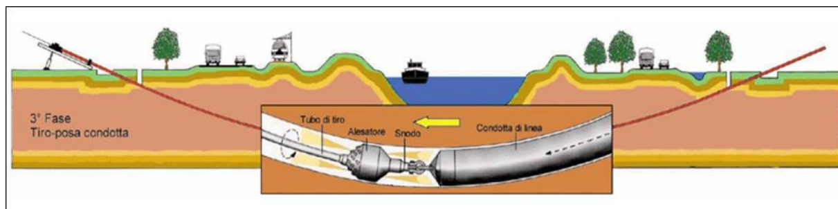
Fig. 7.1/K: Varo della condotta
