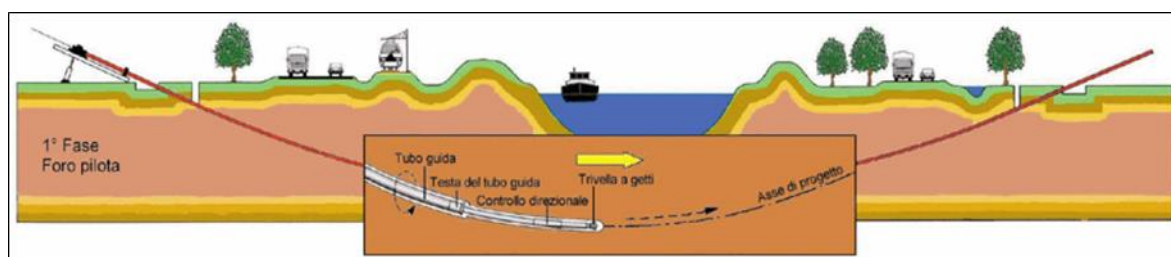
Fig. 7.1/I: Esecuzione del foro pilota
