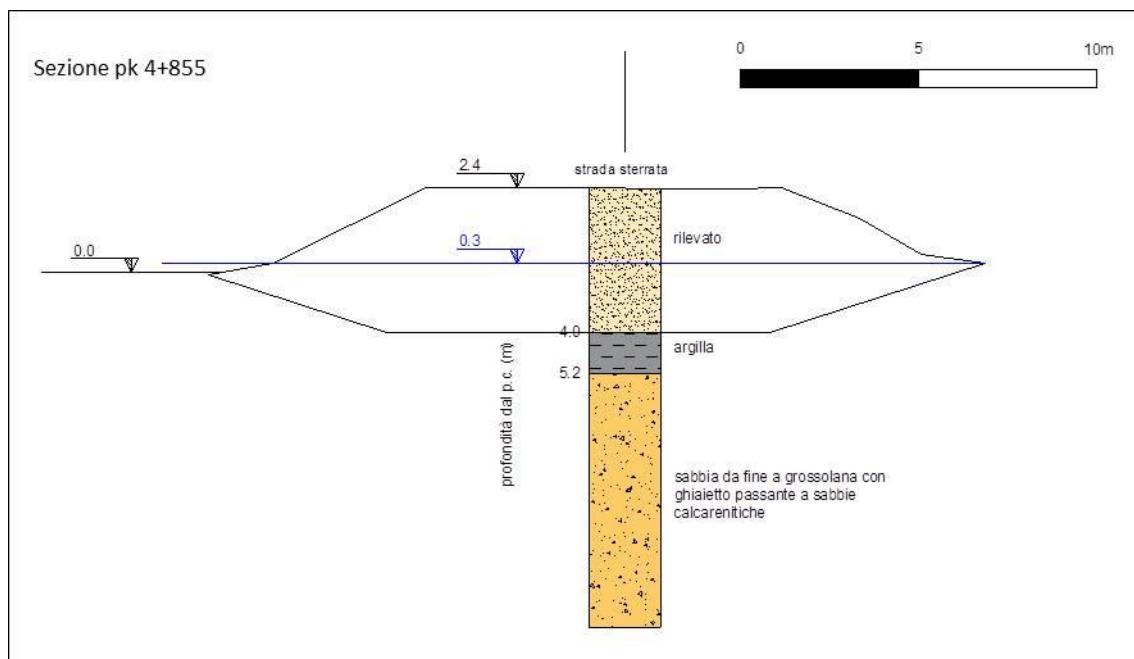
Fig. 7.1/D: Sezione trasversale km 4+855
