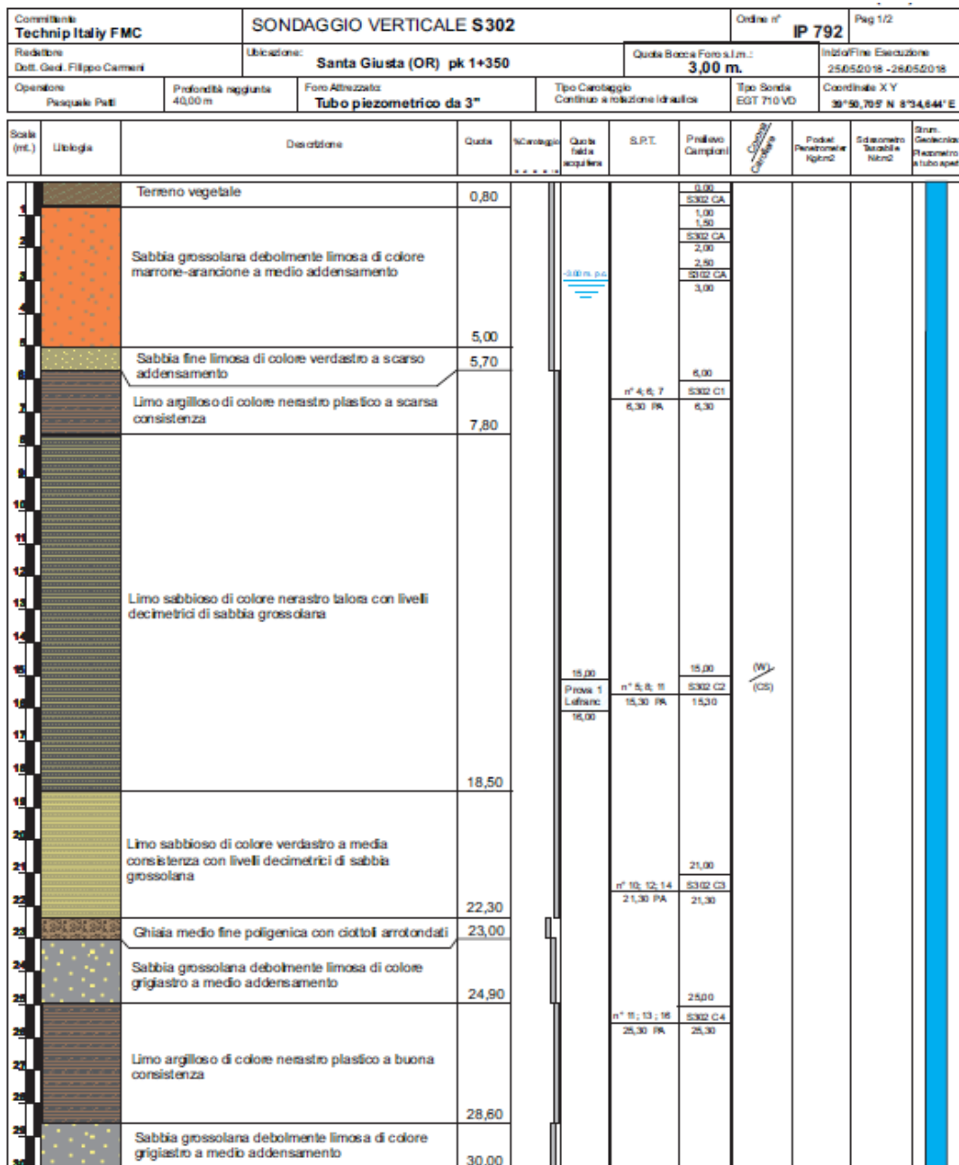
Fig. 7.2/A: Stratigrafia risultante da sondaggio geognostico eseguito in prossimità dello Stagno di S. Giusta.
