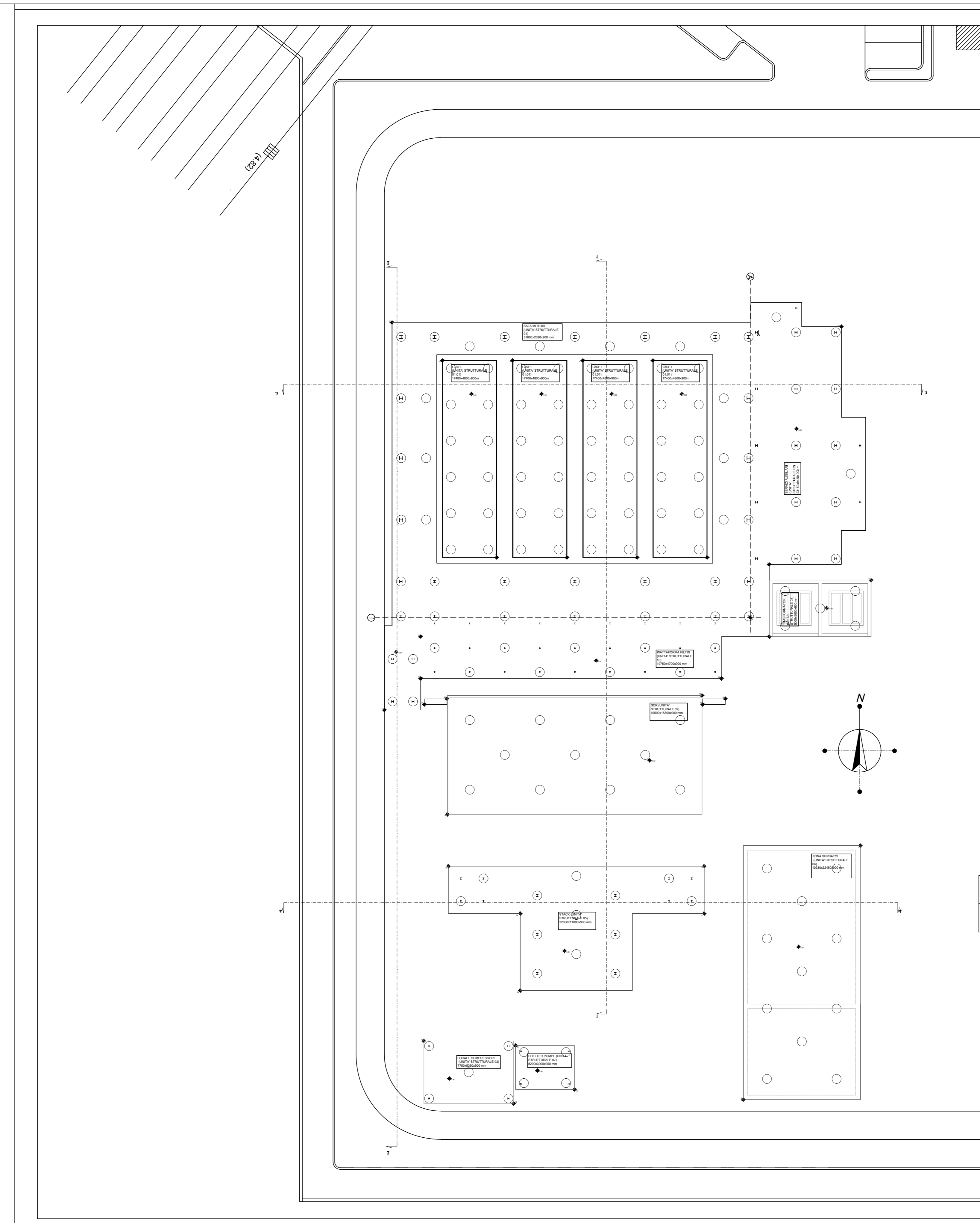
PIANTA DELLE FONDAZIONI
