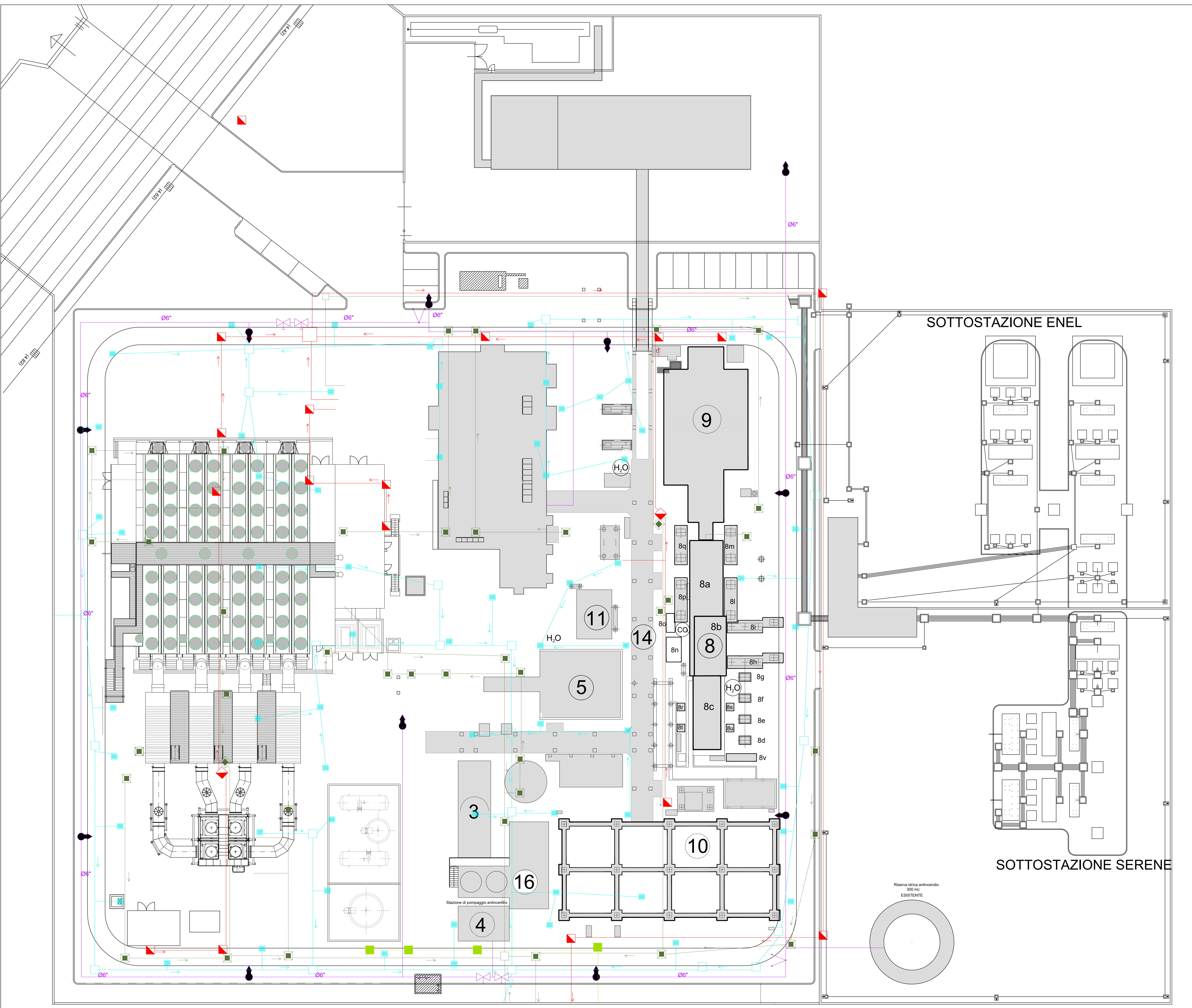
PLANIMETRIA DEI SOTTOSERVIZI
