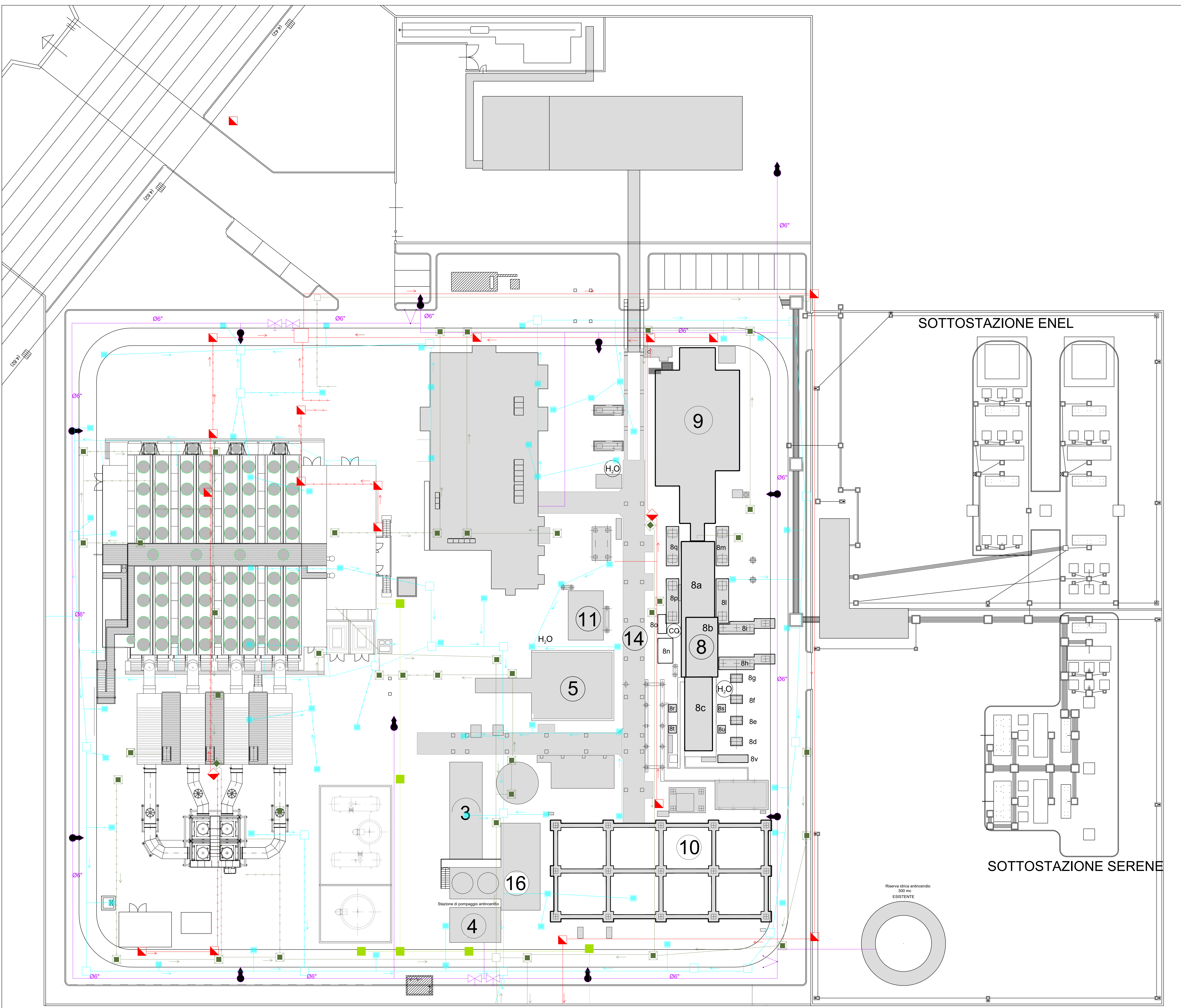
PLANIMETRIA DEI SOTTOSERVIZI
