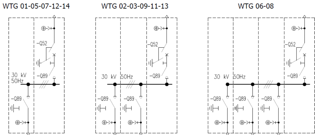
Figura 2- Schemi unifilari quadri MT installati alla base degli aerogeneratori
