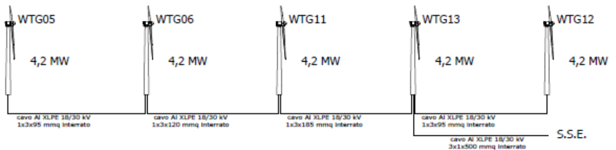
Figura 1 - Schema sottocampi impianto eolico
