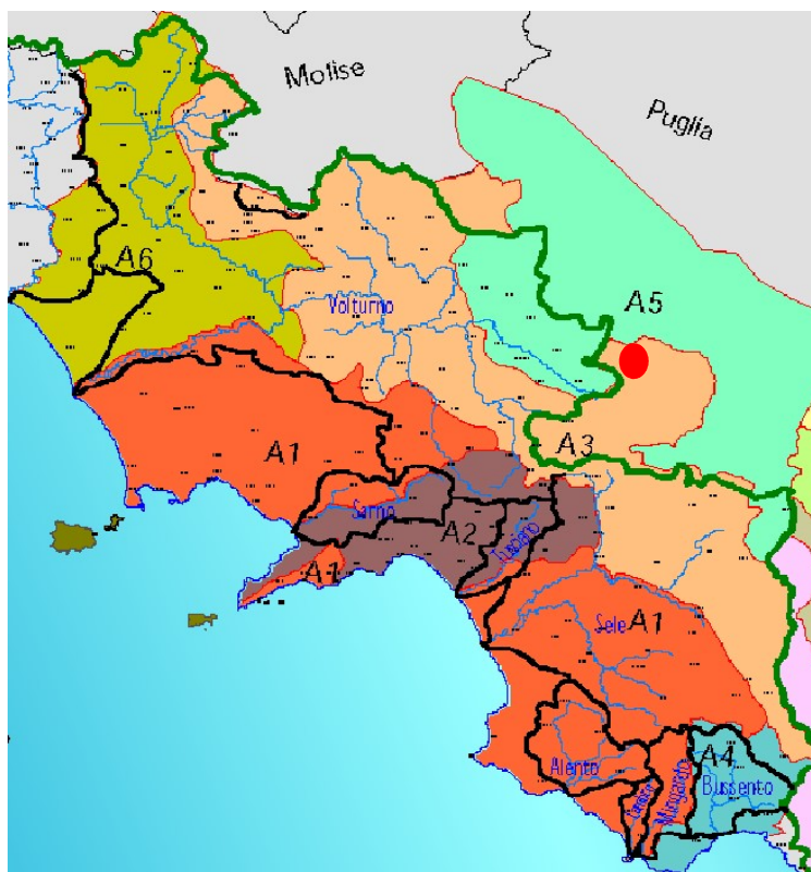
Figura 4: corografia schematica della Regione Campania con indicazione della suddivisione del territorio in 6 aree pluviometriche omogenee per quanto riguarda la regionalizzazione delle medie dei massimi annuali delle altezze di pioggia giornaliera. In rosso l'individuazione dell'area d'intervento.
