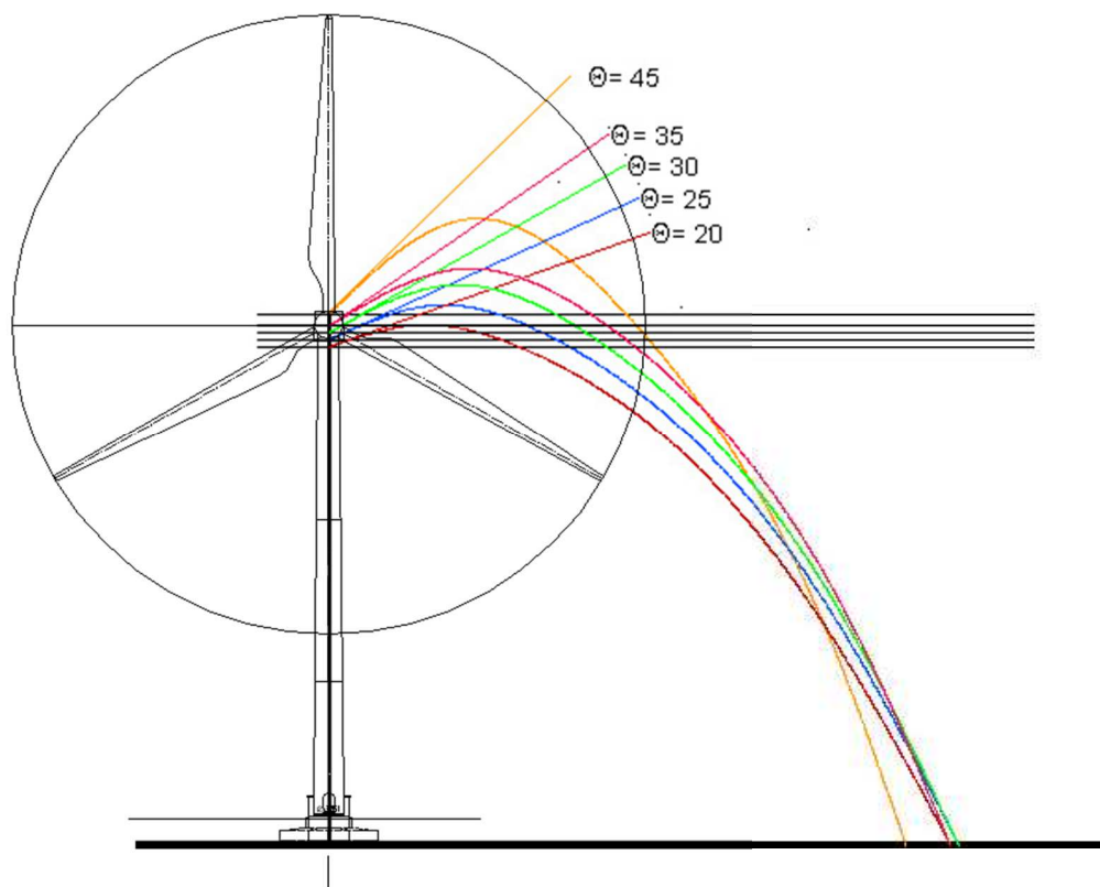
Figura 2 - Traiettoria di caduta in relazione all'angolo \theta
