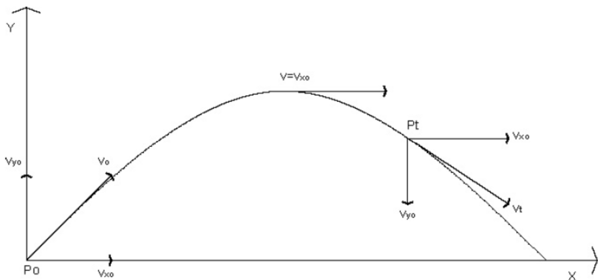
Figura 1 - Traiettoria di un grave in caduta
