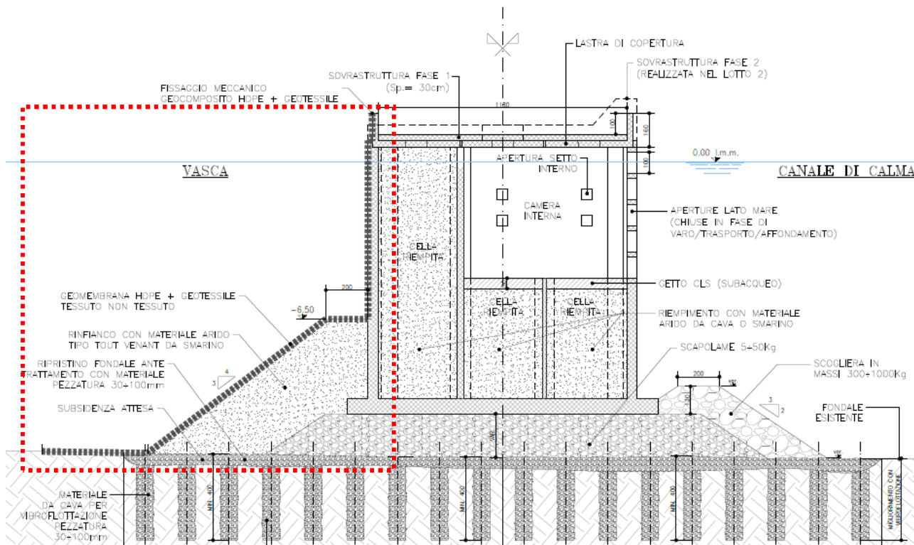
Figura 4-14. Sezione tipologica cassone con rinfianco e posa geomembrana Progetto Esecutivo
