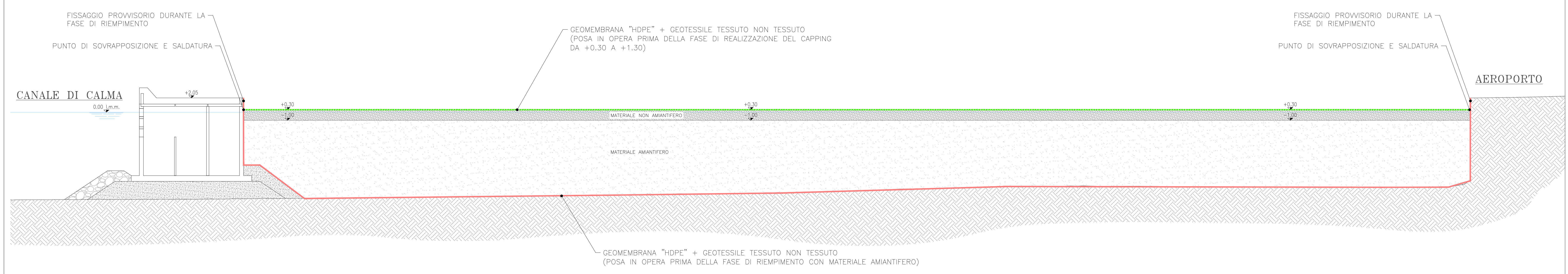
SEZIONE TRASVERSALE TIPO
