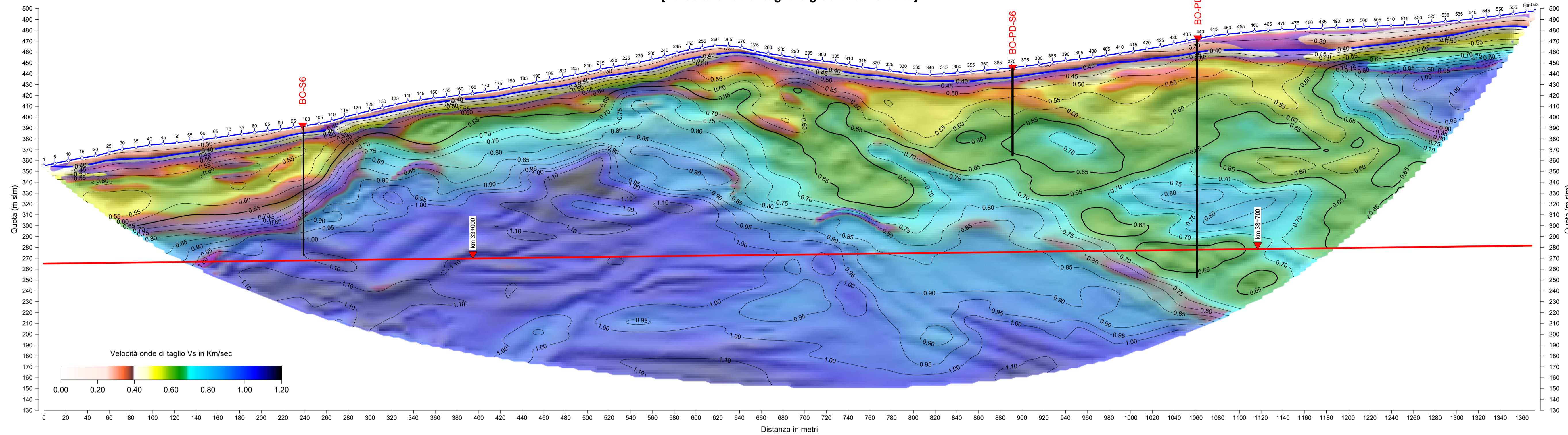
Log galleria - Velocità onde di compressione (km/sec)
