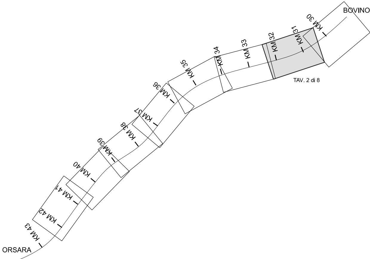
KEY-PLAN
