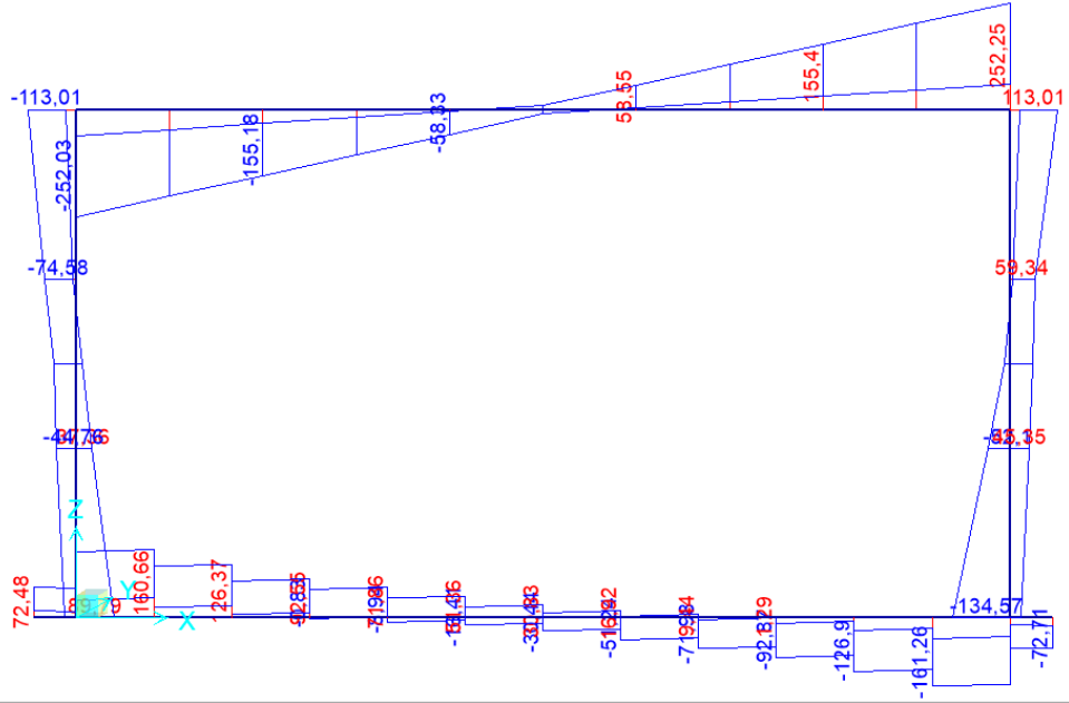
Figura 9-4 – Sforzi assiali ENVE_SISMA
