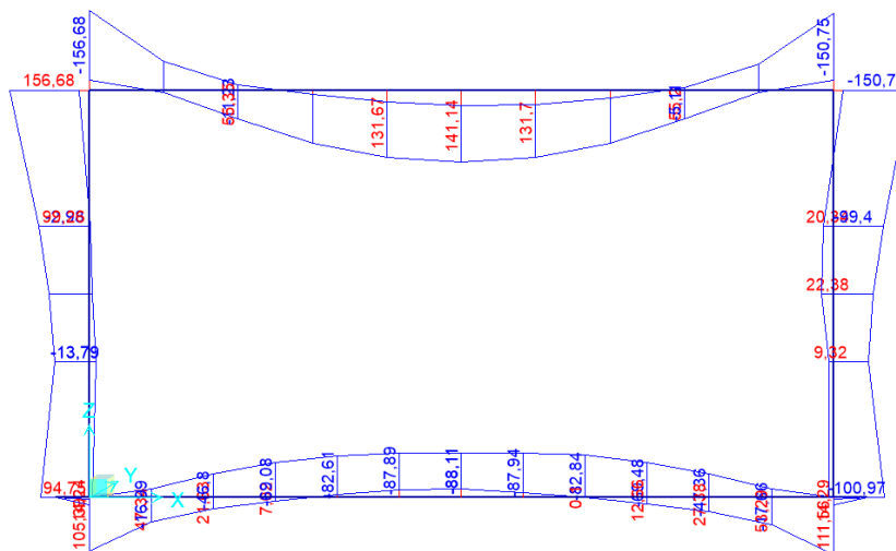
Figura 9-2 – Momenti flettenti ENVE_SLU
