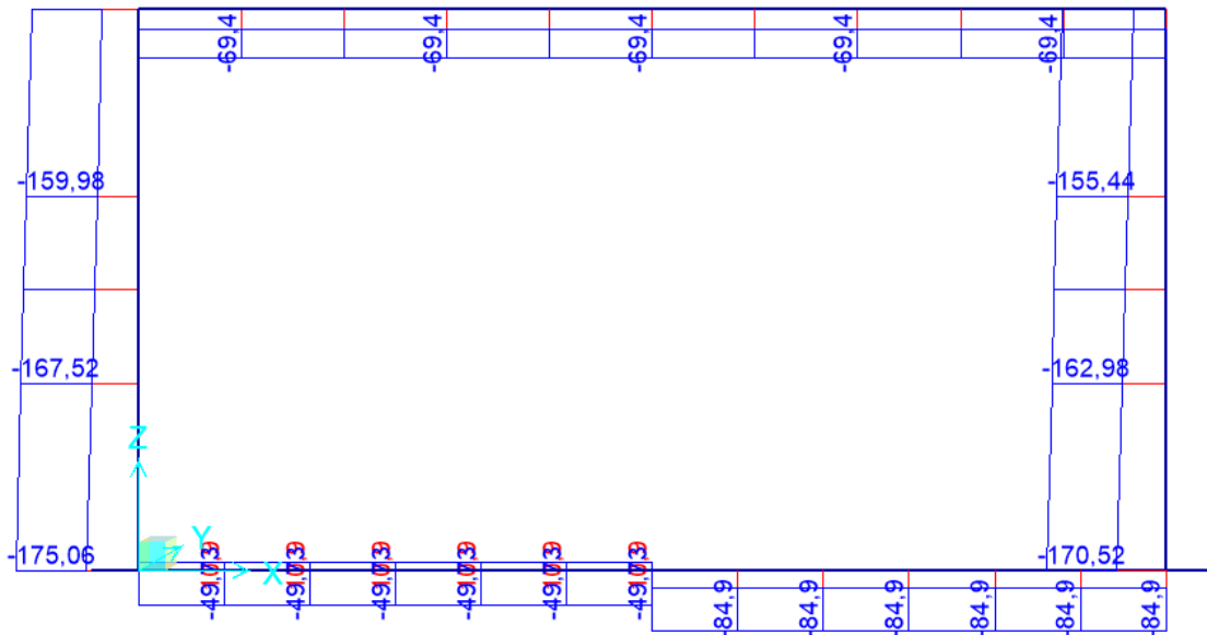
Figura 9-7 – Sforzi assiali ENVE_SLE
