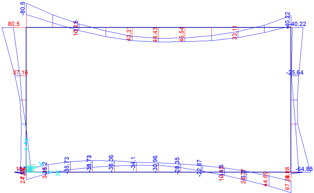
Figura 9-5 – Momenti flettenti ENVE_SISMA
