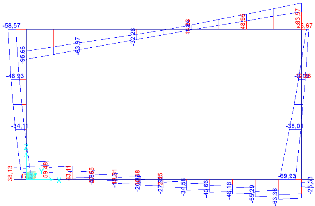
Figura 9-6 – Sforzi di taglio ENVE_SISMA
