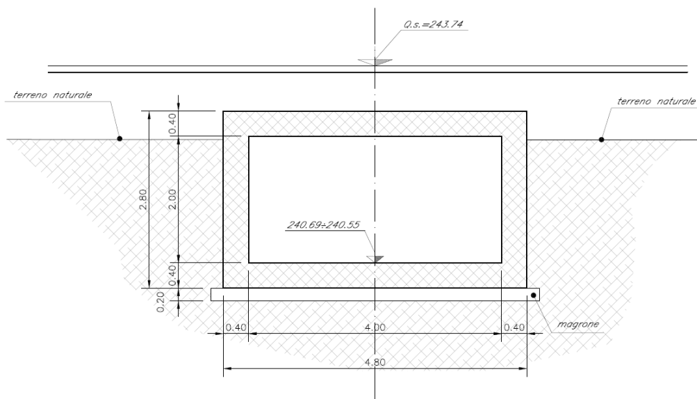
Figura 1-1 – Sezione tombino scatolare stradale IN01_E
