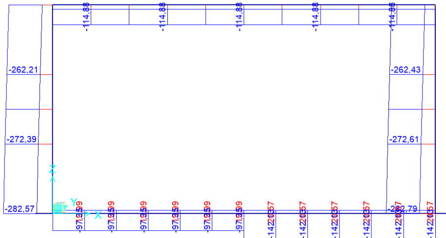
Figura 9-2 – Momenti flettenti ENVE_SLU
