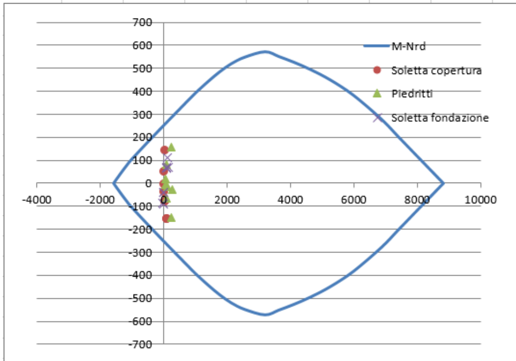
Figura 10-1 Verifica a pressoflessione
