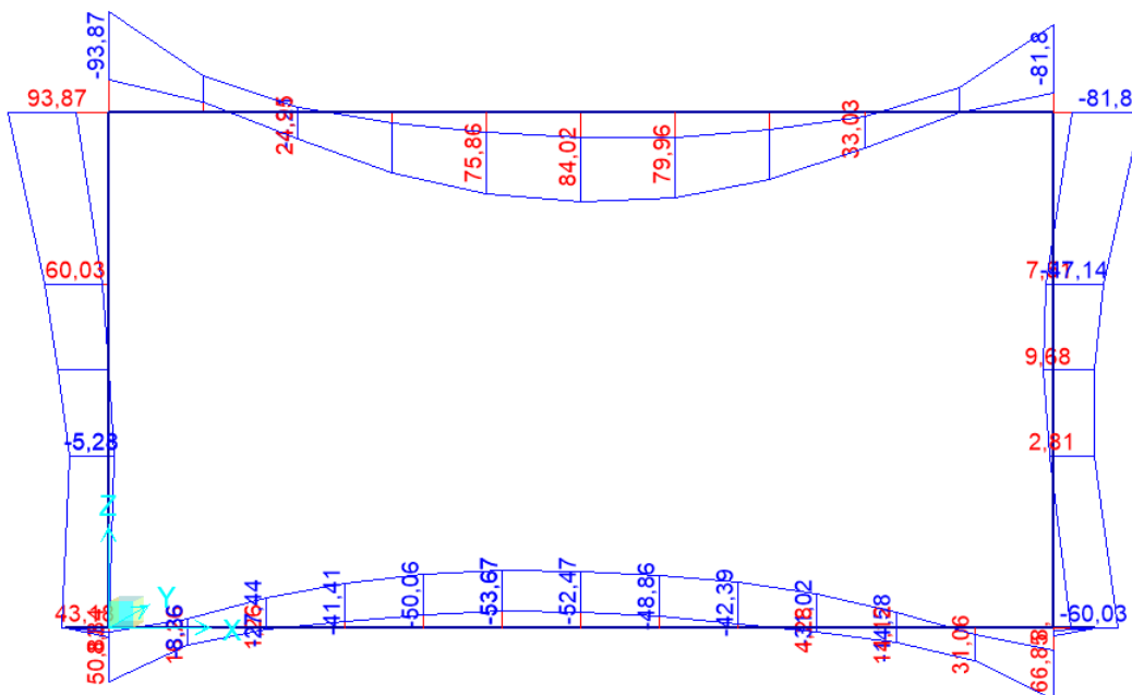
Figura 9-8 – Momenti flettenti ENVE_SLE
