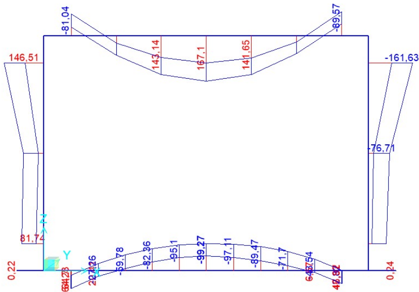
Figura 9-2 – Momenti flettenti ENVE_SLU
