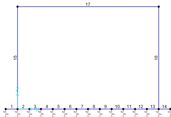
Figura 8-1 – Modello di calcolo
