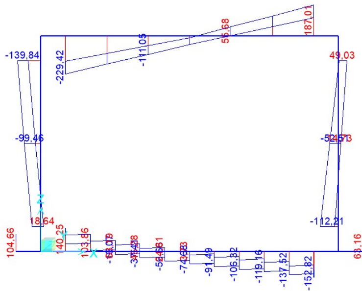
Figura 9-6 – Sforzi di taglio ENVE_SISMA
