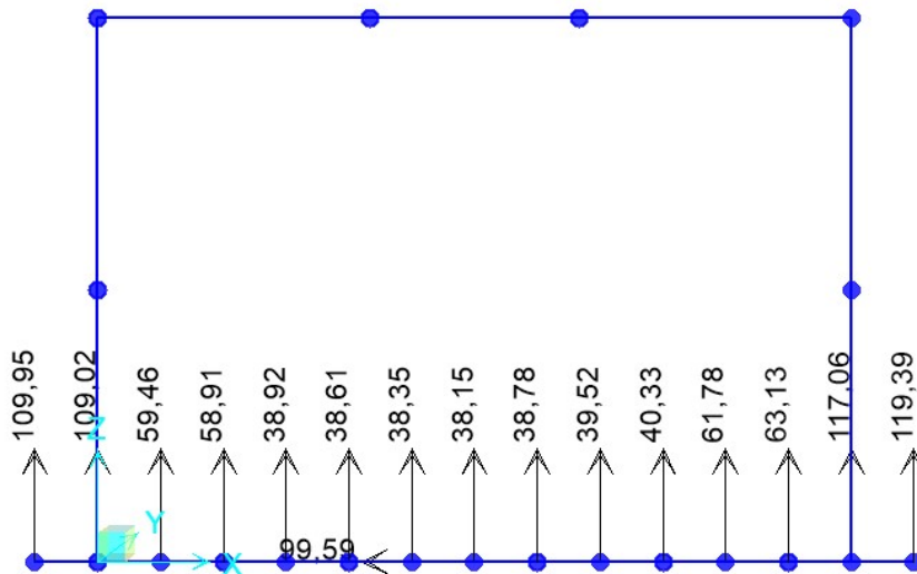
Figura 11-1 – Reazioni molle in fondazione
