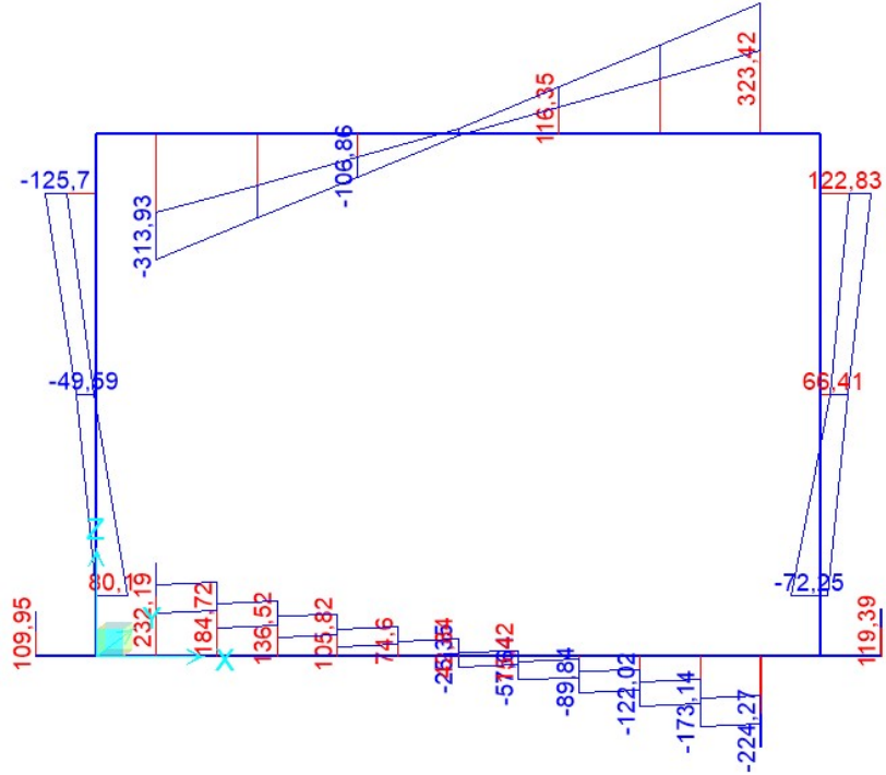
Figura 9-3 – Sforzi di taglio ENVE_SLU
