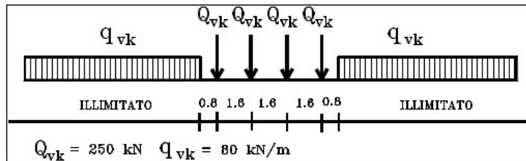
Figura 6-1 – Treno di carico LM71
