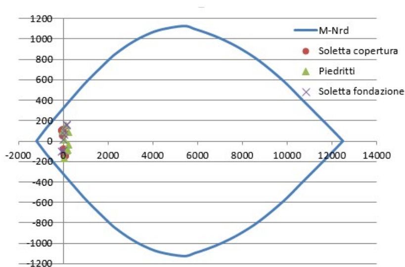
Figura 10-1 Verifica a pressoflessione
