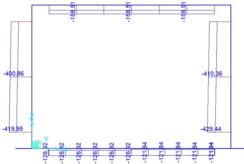
Figura 9-2 – Momenti flettenti ENVE_SLU
