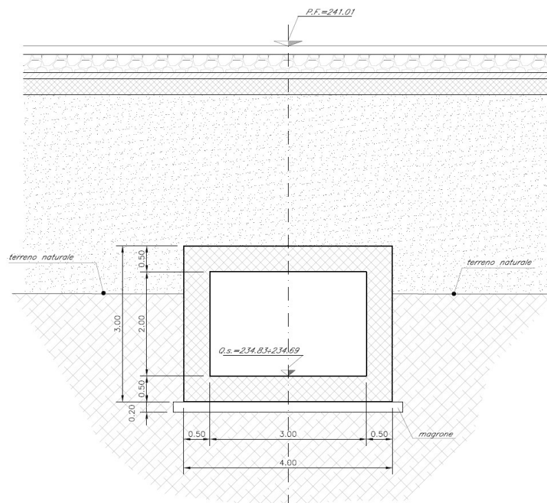
Figura 1-1 – Sezione tombino scatolare ferroviario IN02 A
