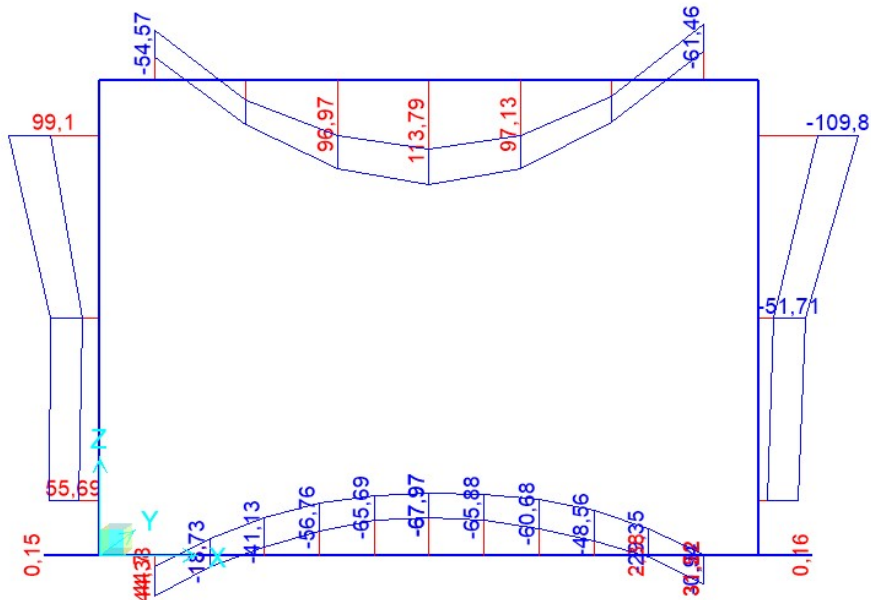
Figura 9-8 – Momenti flettenti ENVE_SLE
