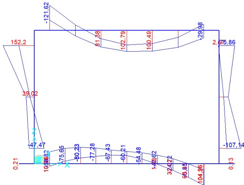
Figura 9-5 – Momenti flettenti ENVE_SISMA
