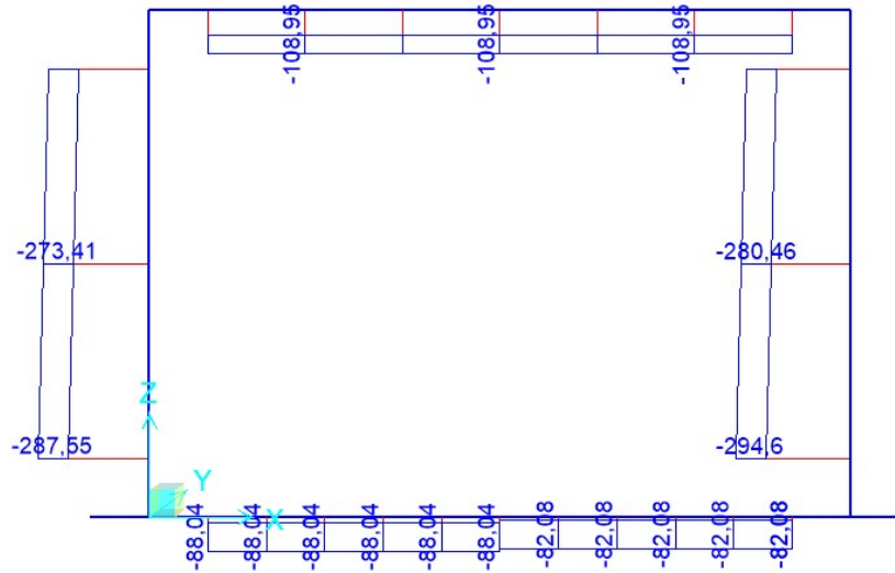
Figura 9-7 – Sforzi assiali ENVE_SLE
