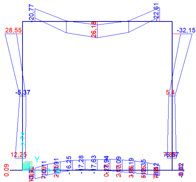
Figura 9-8 – Momenti flettenti ENVE_SLE
