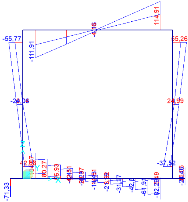
Figura 9-3 – Sforzi di taglio ENVE_SLU
