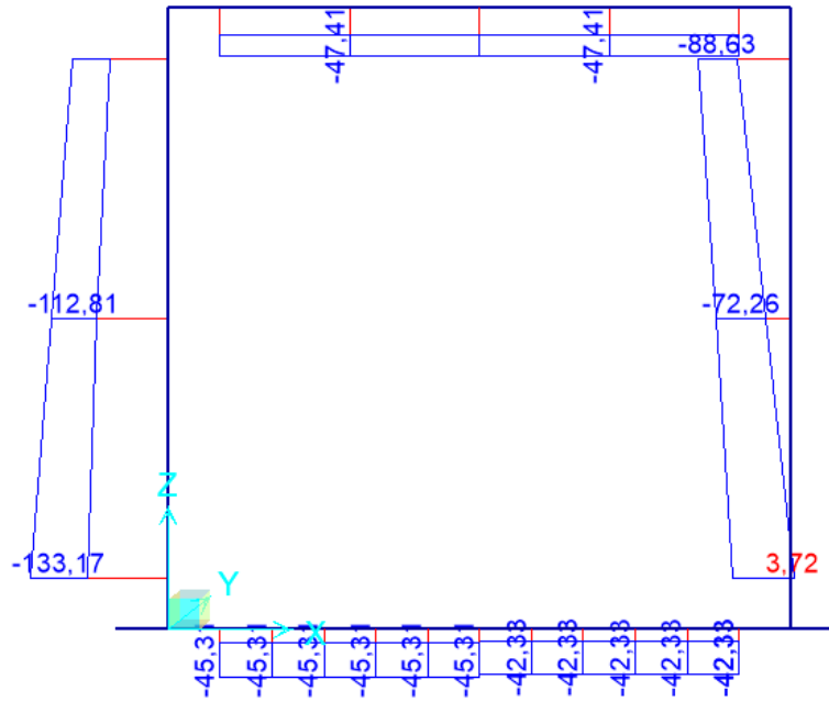
Figura 9-7 – Sforzi assiali ENVE_SLE
