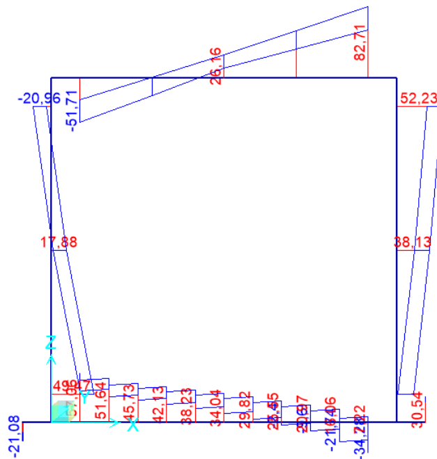
Figura 9-6 – Sforzi di taglio ENVE_SISMA
