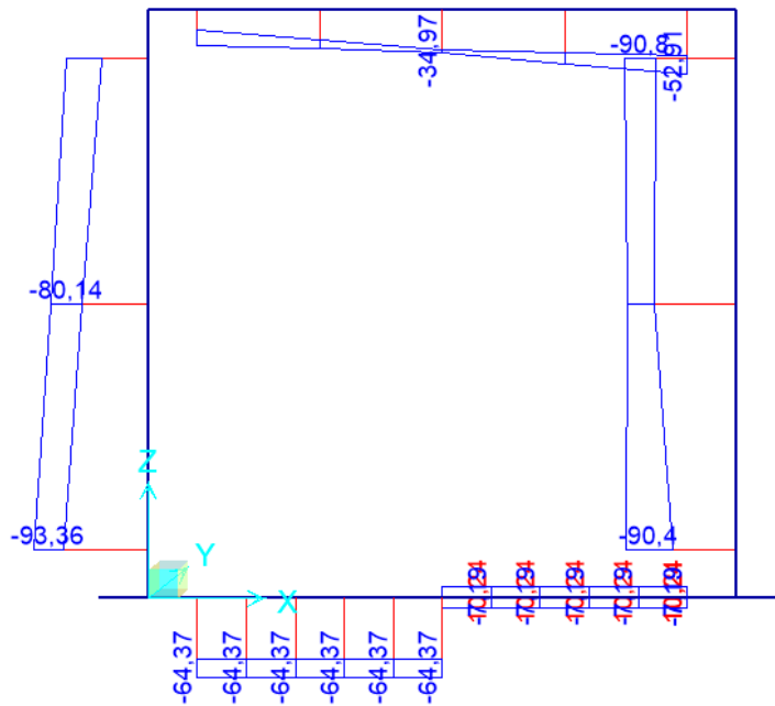
Figura 9-4 – Sforzi assiali ENVE_SISMA
