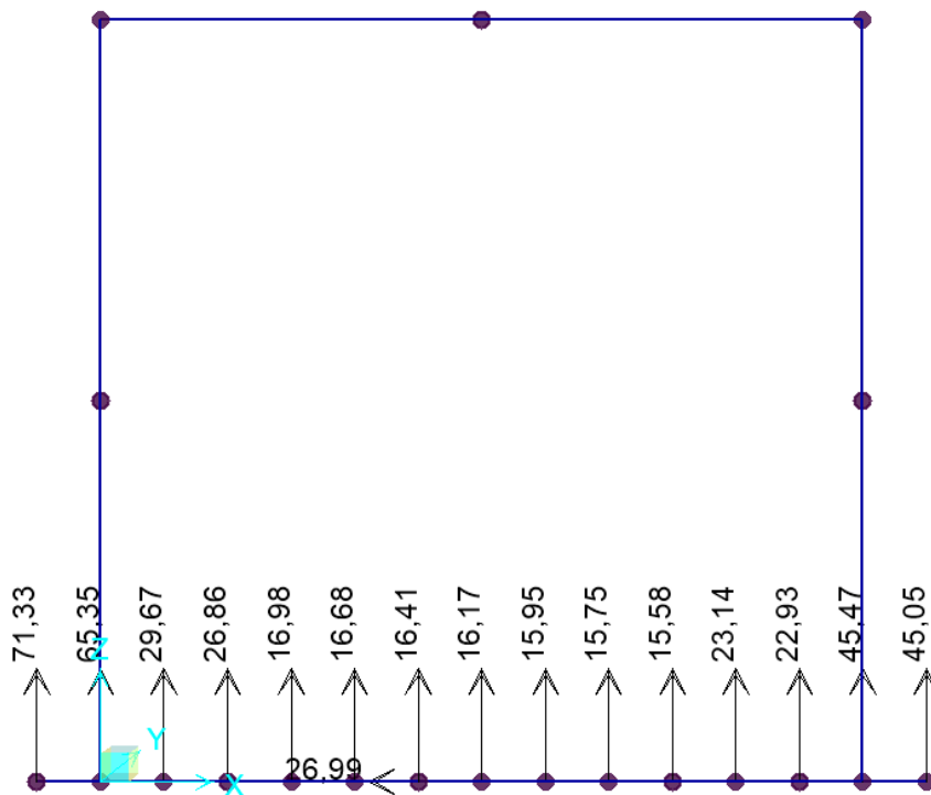
Figura 11-1 – Reazioni molle in fondazione
