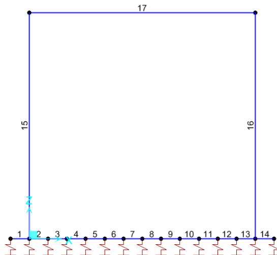
Figura 8-1 – Modello di calcolo
