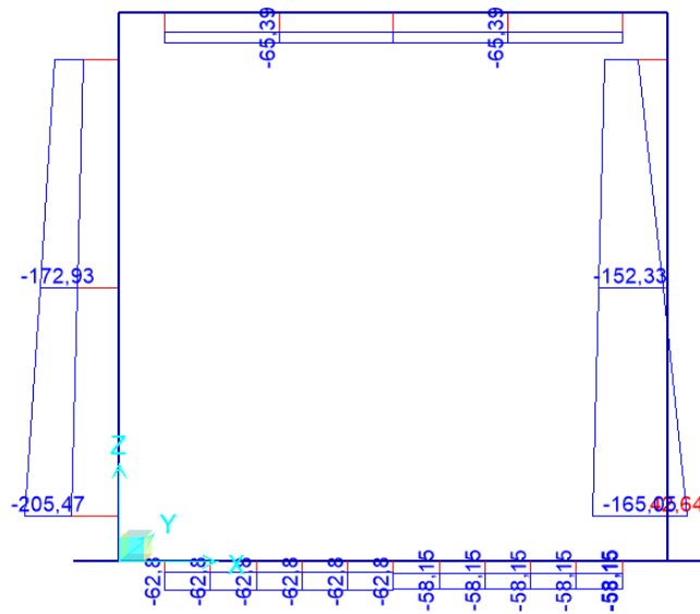
Figura 9-2 – Momenti flettenti ENVE_SLU
