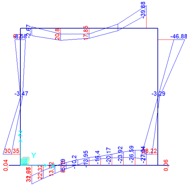
Figura 9-5 – Momenti flettenti ENVE_SISMA
