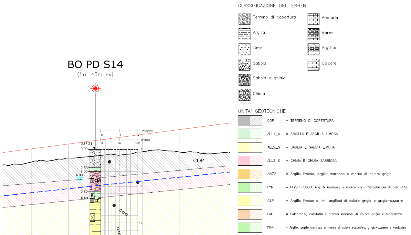
Figura 4-1 – Stralcio profilo geotecnico tratta di riferimento
