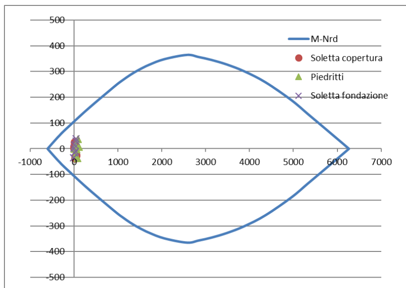
Figura 10-1 Verifica a pressoflessione
