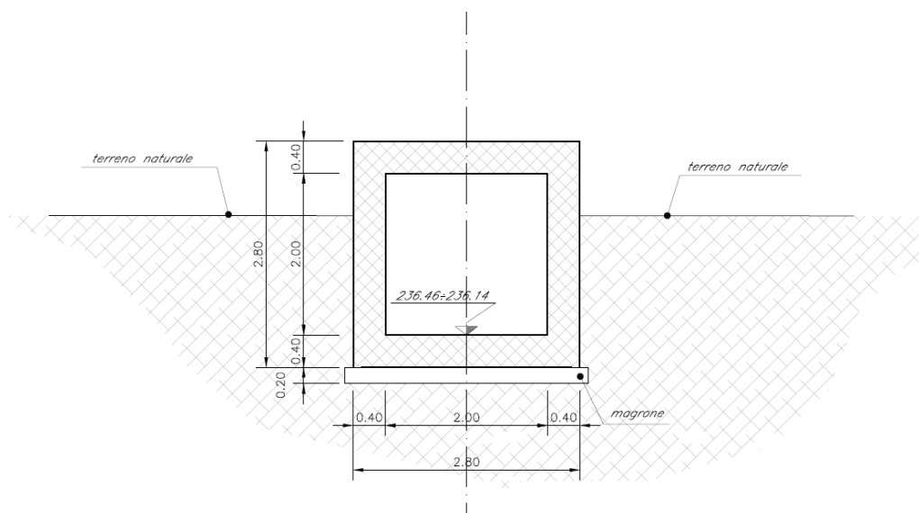
Figura 1-1 – Sezione tombino scatolare stradale IN02 B
