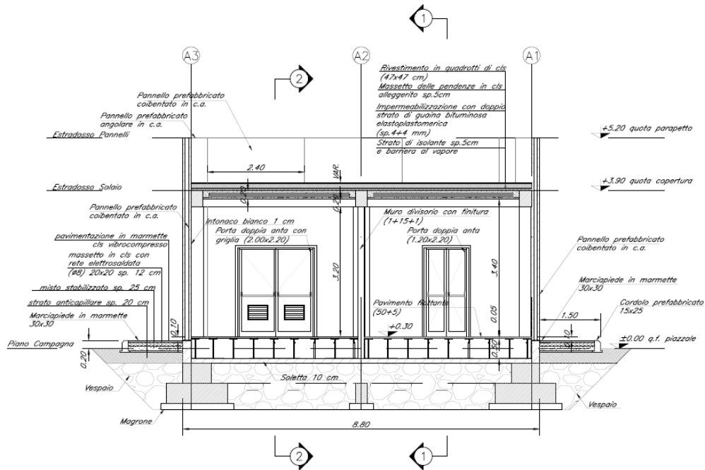
Figura 2 Sezione longitudinale
