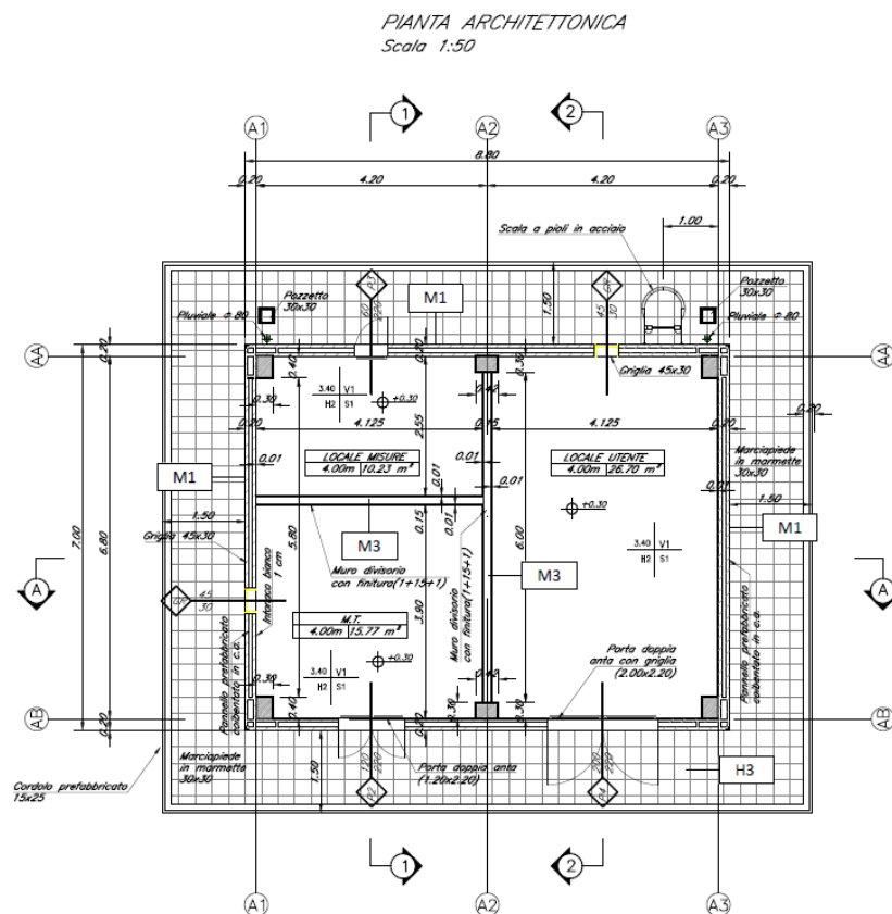
Figura 1 Pianta architettonica
