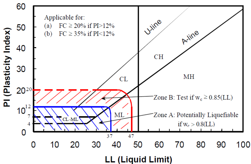
Fig. 6: Criterio di esclusione dei terreni coesivi (NCEER, Seed et al., 2003)
