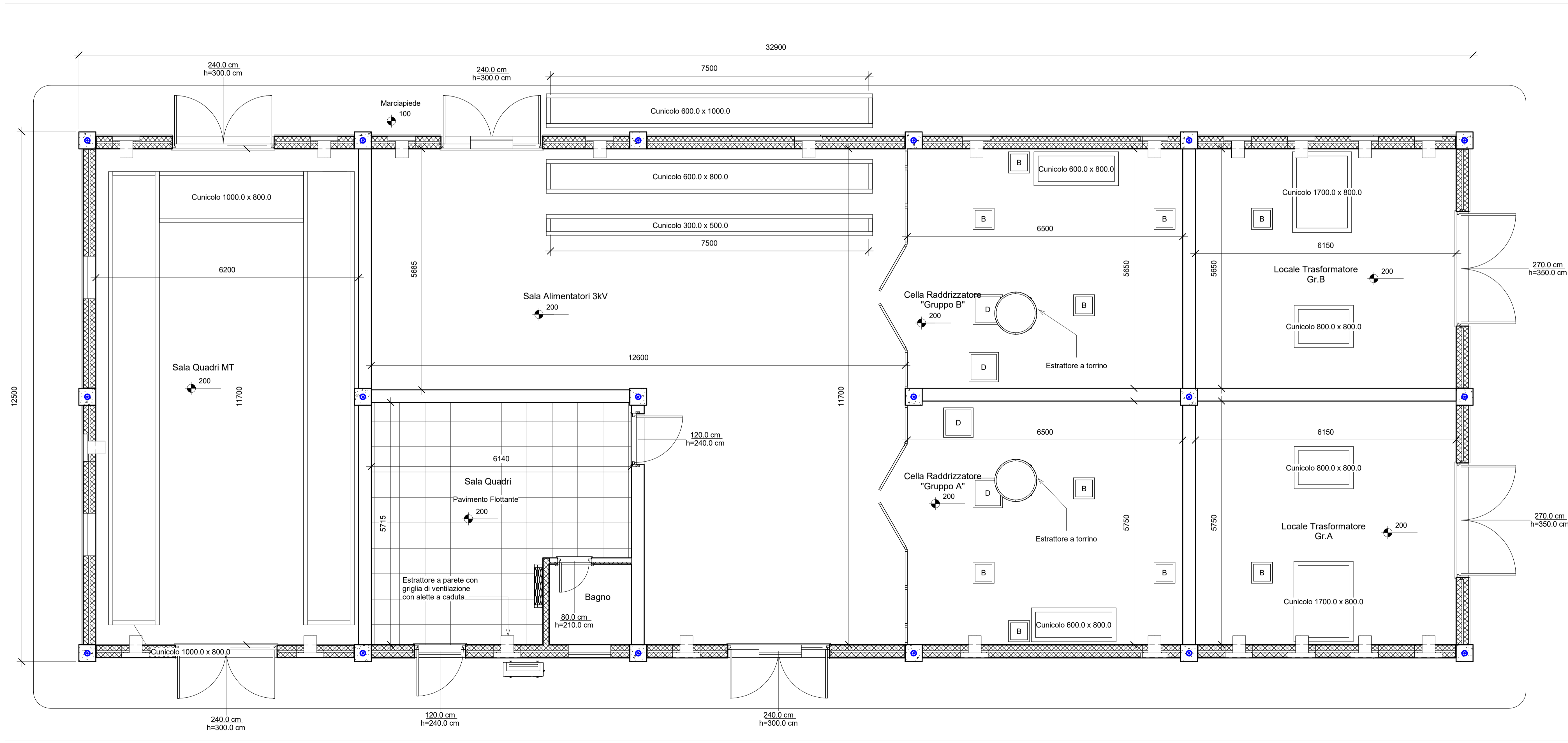
1 Pianta piano Terra 1 : 50
