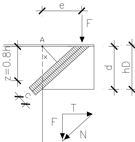
F7. modello di calcolo tirante - puntone
