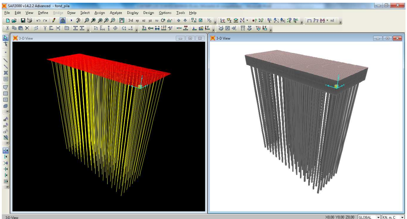
F15. Modello agli EF del sistema terreno-struttura
