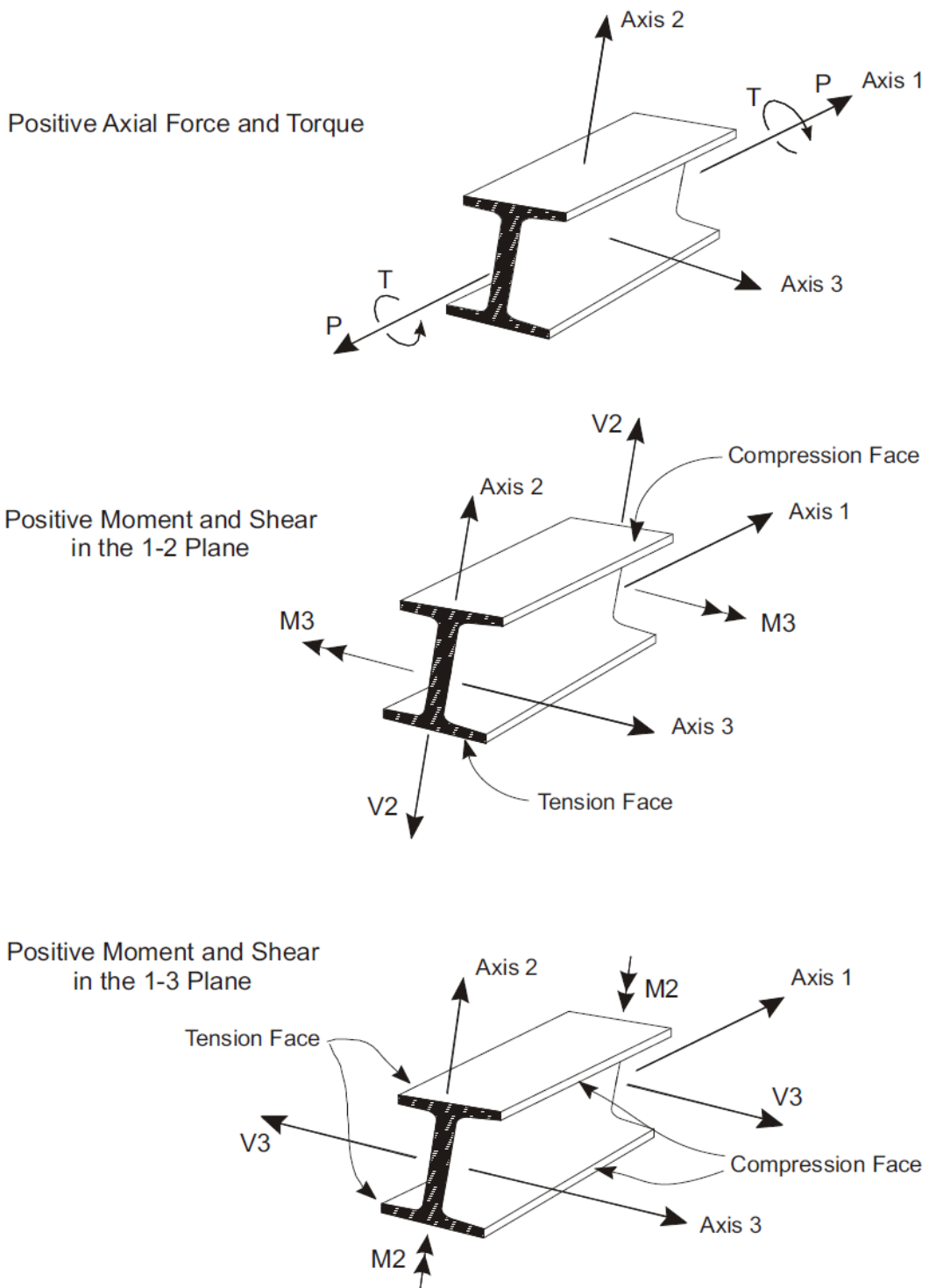
F3. Azioni e Sollecitazioni positive negli elementi tipo "line"
