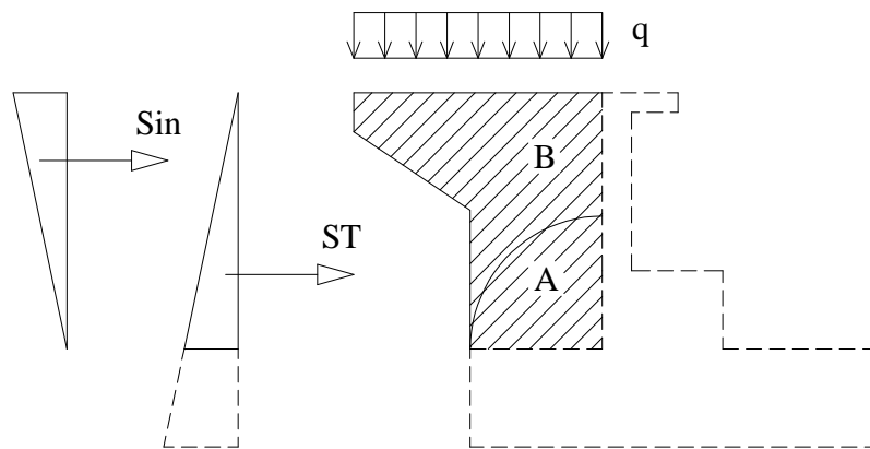
F9. sezione longitudinale dei muri di risvolto e schema delle azioni
