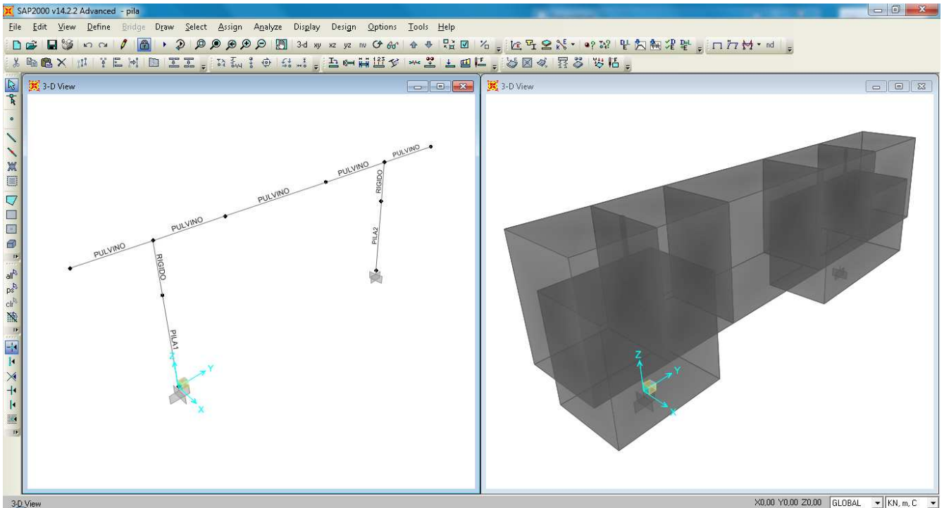
F11. Modello della pila agli EF
