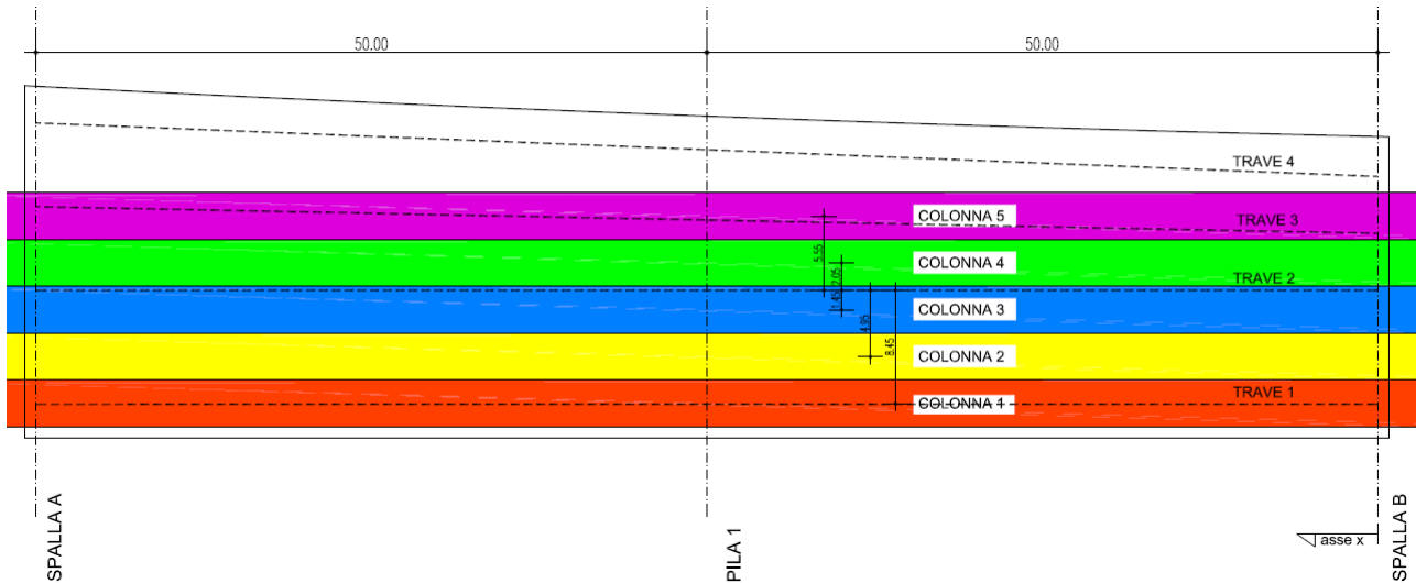
F2. Disposizione delle colonne di carico – vista planimetrica
