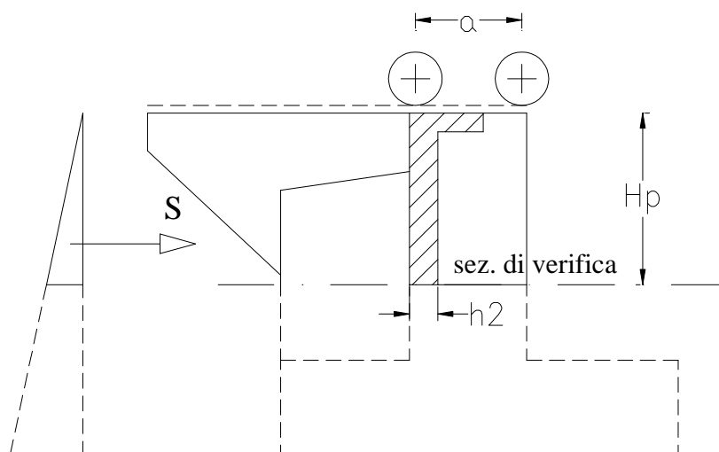
F8. schema azioni
