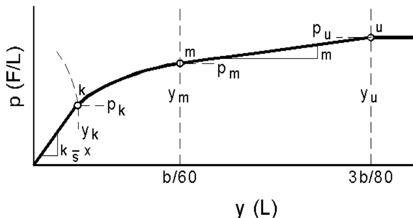
F14. Digramma p-y secondo Reese, Cox e Koop
