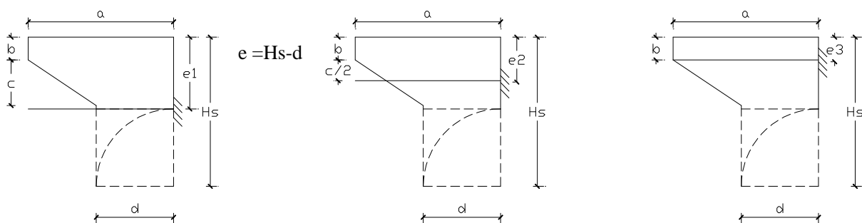
F10. modelli a mensola
