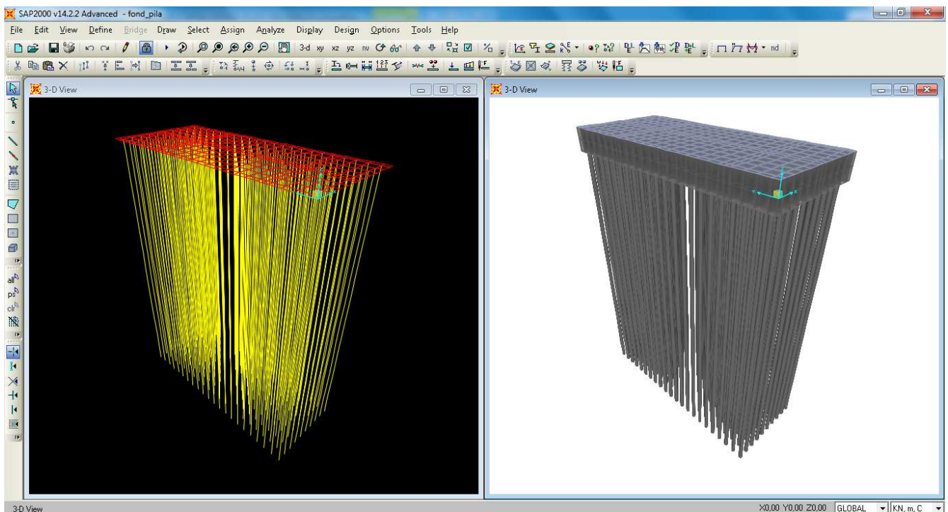
F5. Modello agli EF del sistema terreno-struttura
