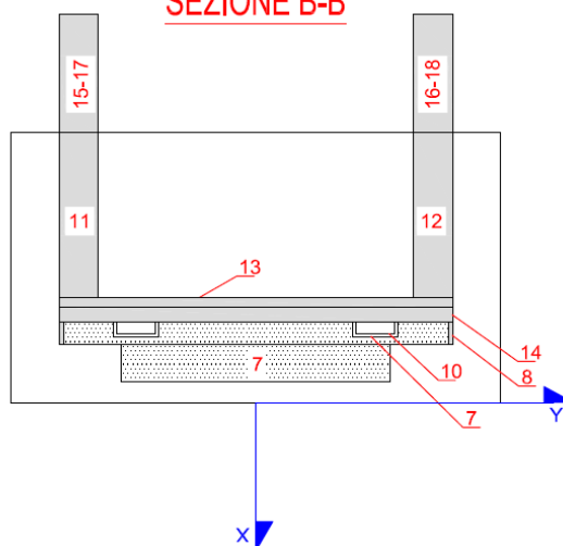
SEZIONE B-B
