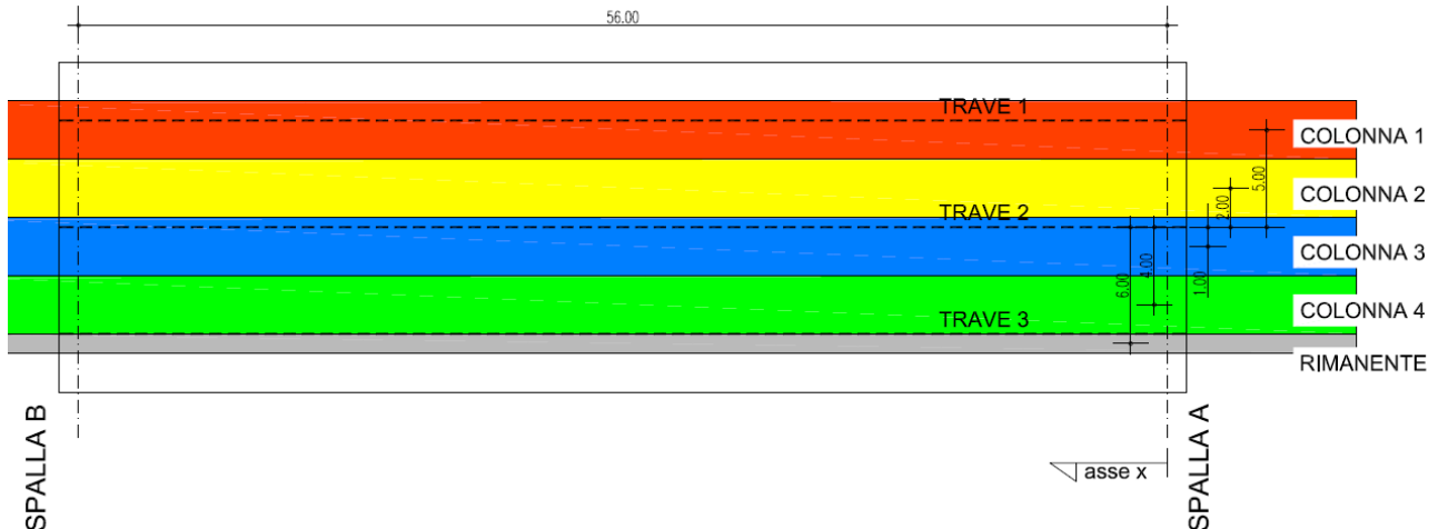
F3. Disposizione delle colonne di carico – vista planimetrica
