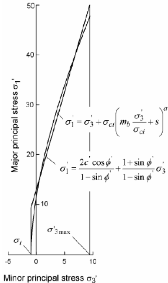
Fig. 21: Relazione fra gli sforzi principali massimi e minimi per il criterio di Hoek-Brown e per quello equivalente di Mohr-Coulomb.
