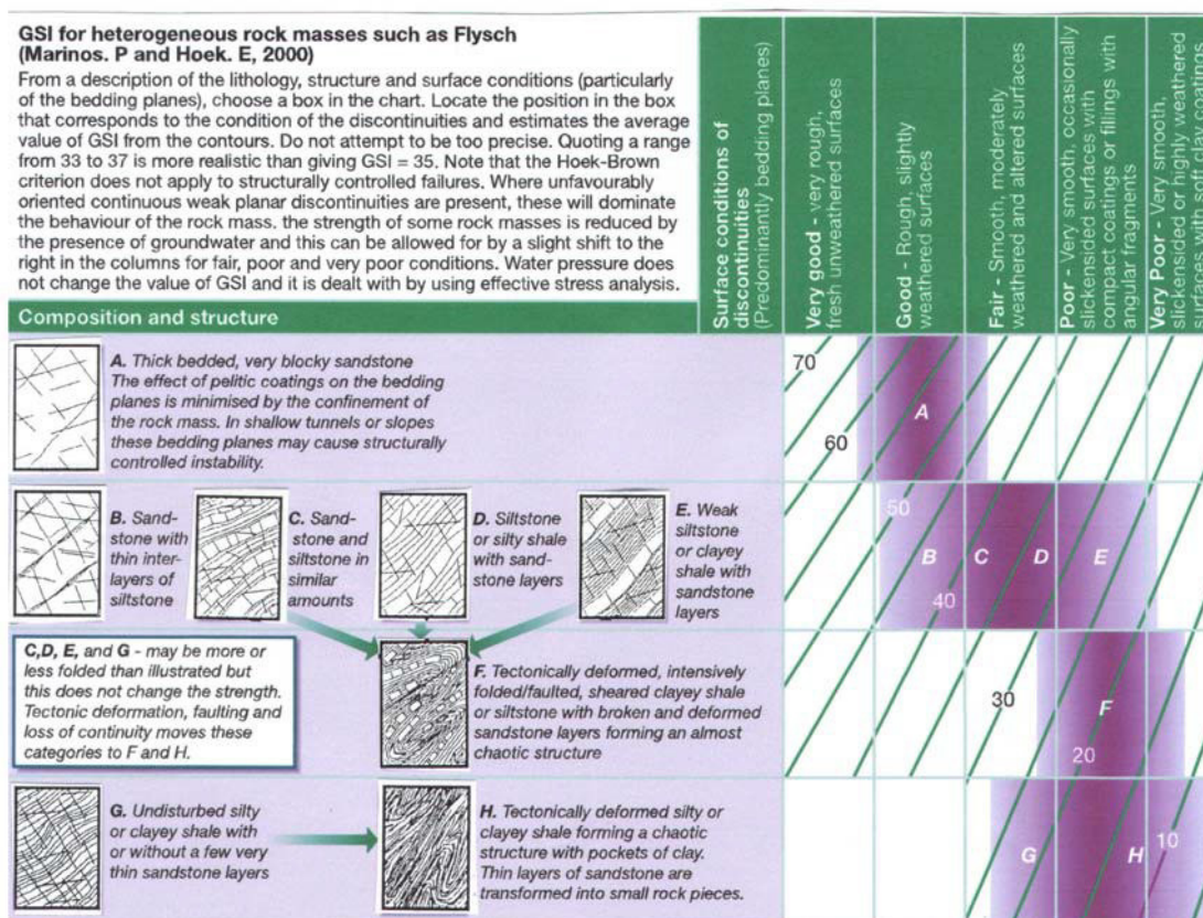
Fig. 27: Stima del valore di GSI (Geological Strength Index) per ammassi rocciosi eterogenei come i Flysch
