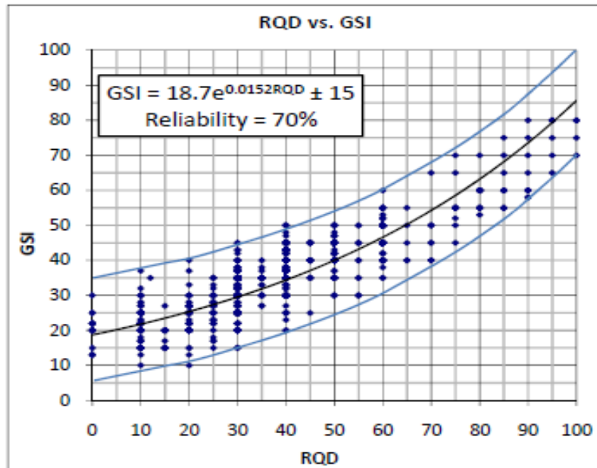
Fig. 19: Correlazione tra RQD e GSI (secondo Truzman et al., 2011)
