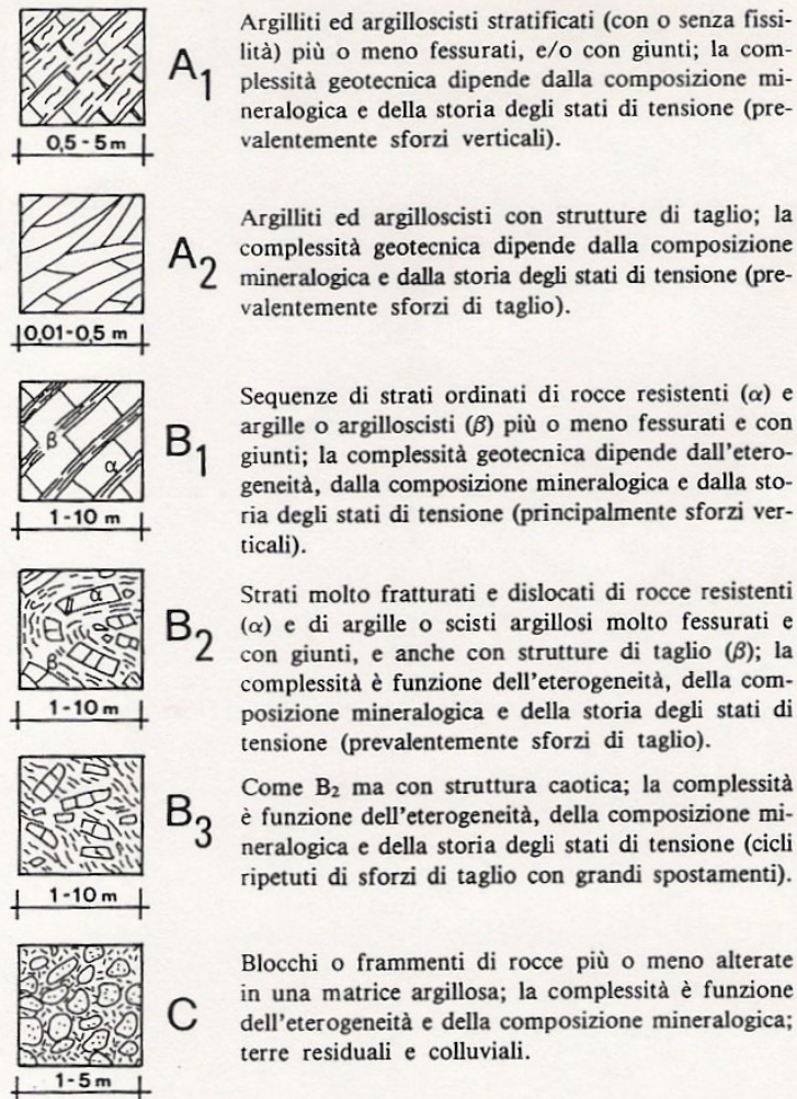
Fig. 26: Tipi di complessità elementari (da A.G.I., 1979)
