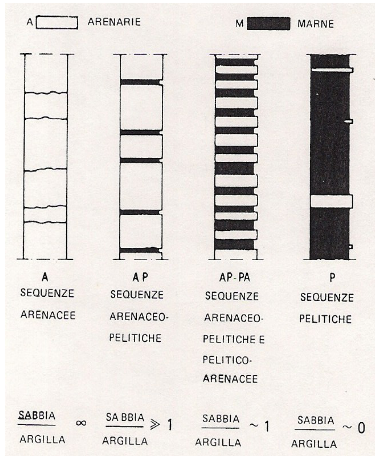
Fig. 23: Classificazione e sequenze arenaceo – pelitiche (da A.G.I., 1979)
