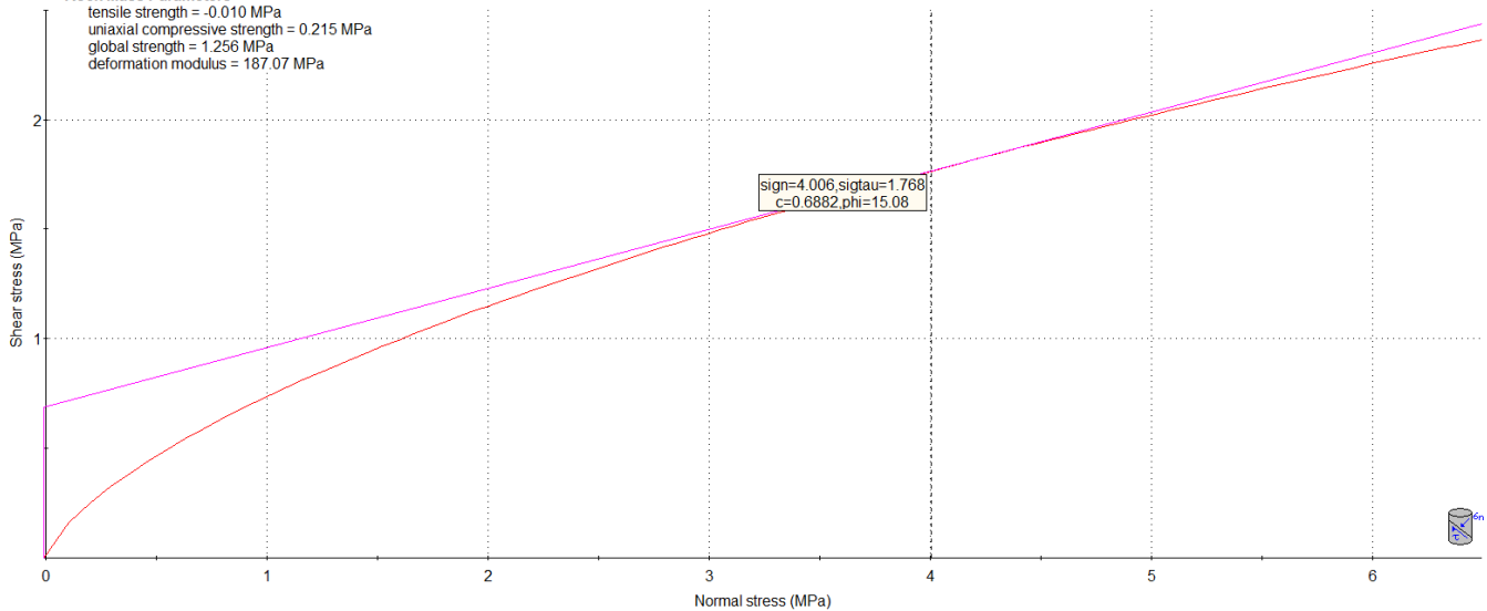
Fig. 22: Esempio di determinazione dei parametri di resistenza al taglio.
