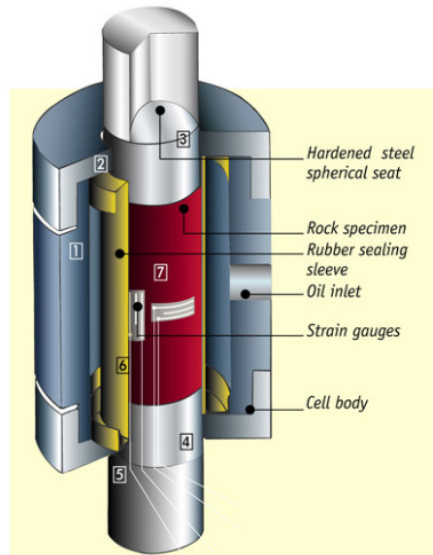
Fig. 20: Cella di Hoek.
