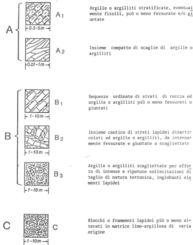
Fig. 25: Classificazione dei terreni strutturalmente complessi (Esu, 1977)
