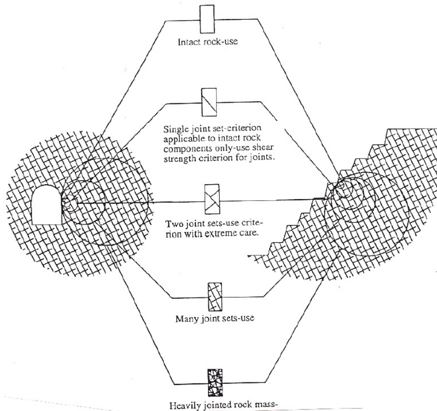
Fig. 15: Condizioni dell'ammasso roccioso ed effetto scala
