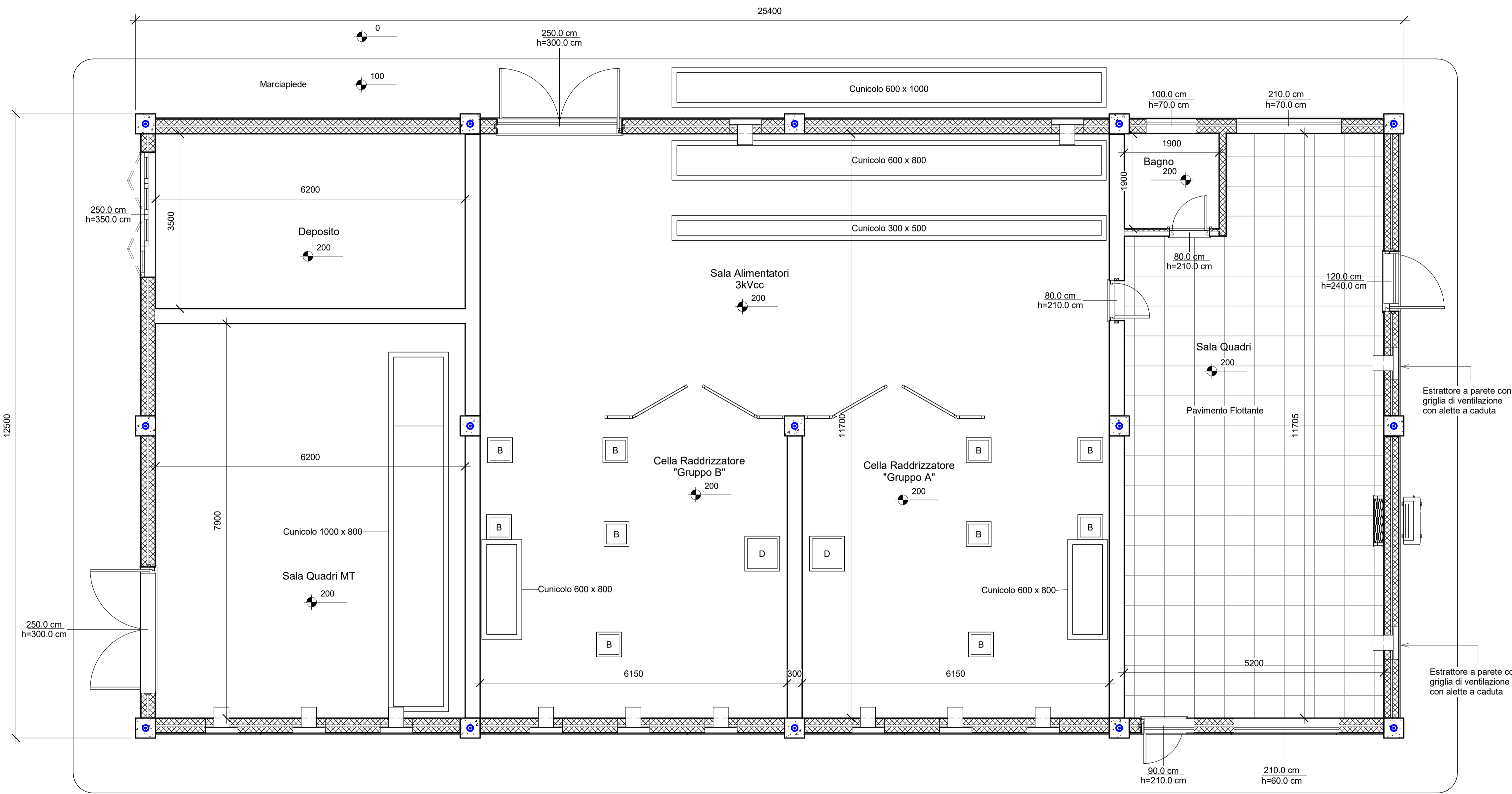
1 Pianta piano Terra 1 : 50
