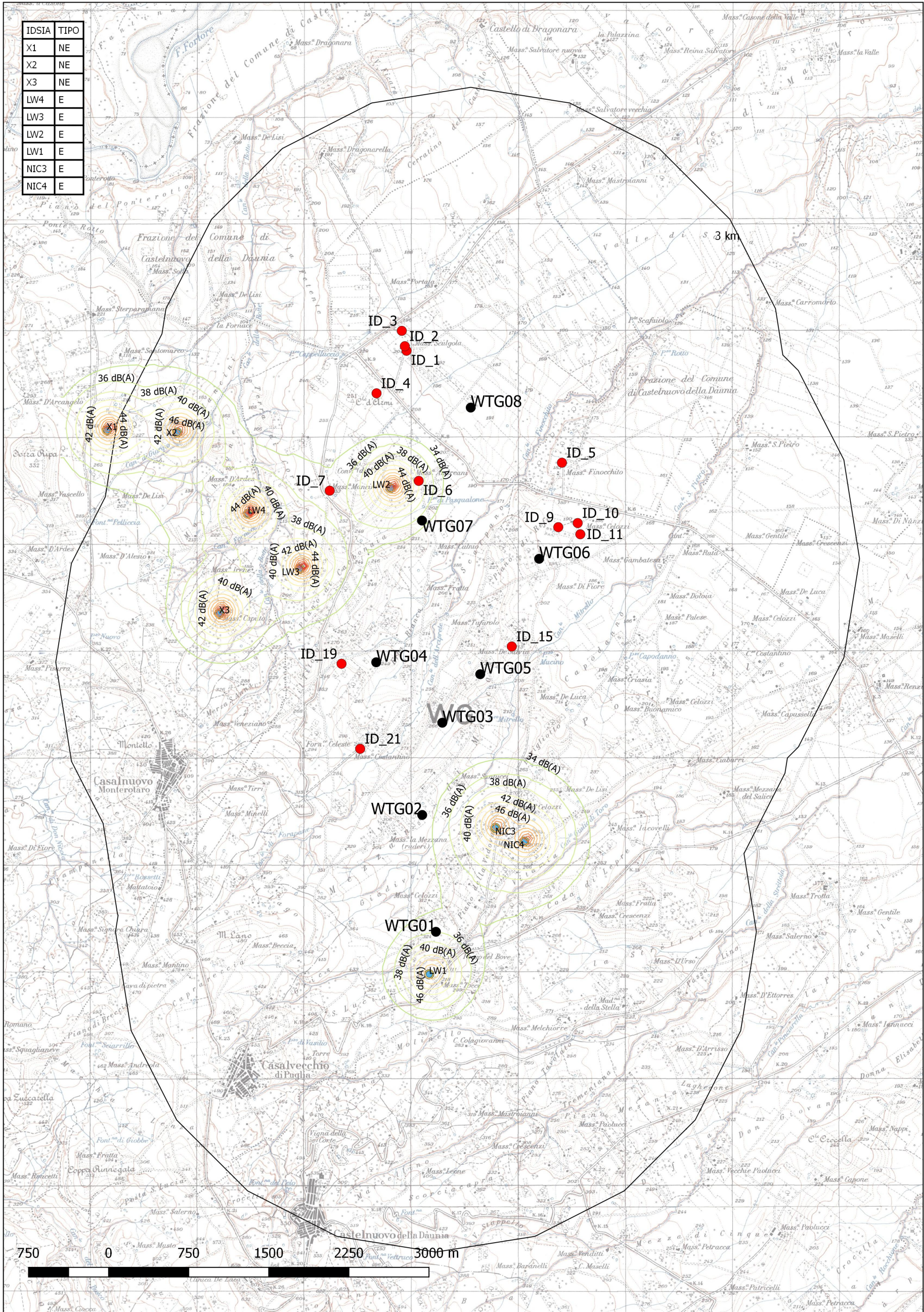
Isofonia del livello acustico prodotto dagli impianti esistenti ed in fase di autorizzazione in un buffer di 3 km dalle WTG in progetto
