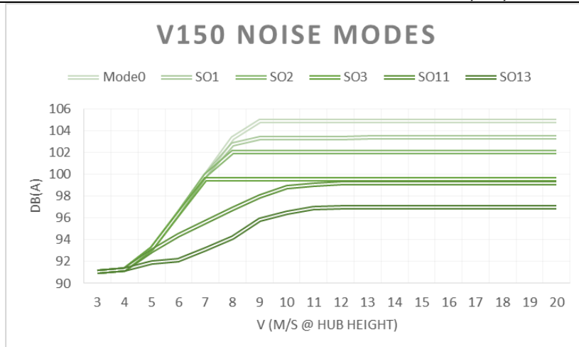
VESTAS V150 – Noise modes – Grafico ricavato dai dati nel documento VESTAS Document no.: 0067-7067 V08 – Rev. 21/12/2017
