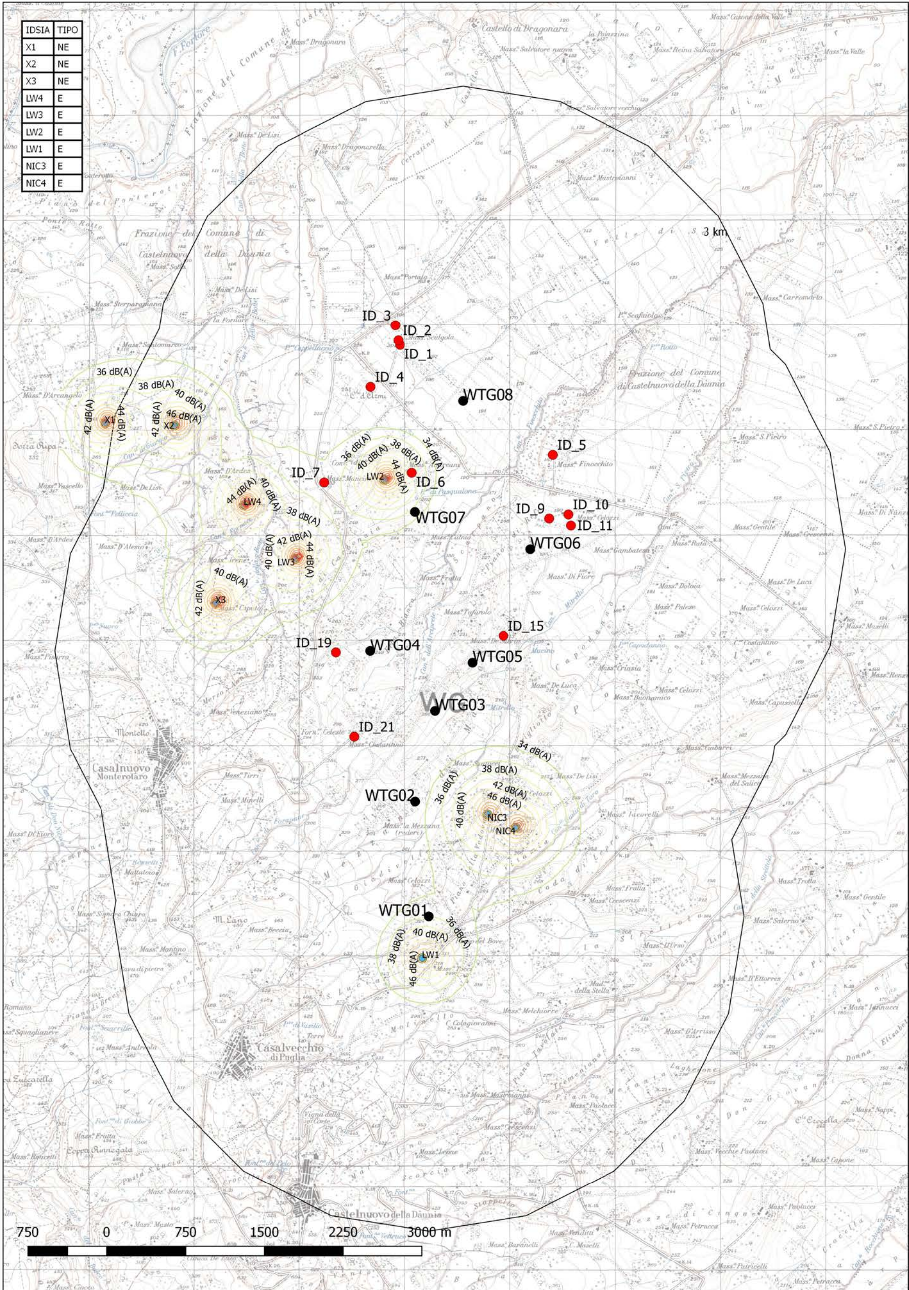
Isofoni del livello acustico prodotto dagli impianti esistenti ed in fase di autorizzazione in un buffer di 3 km dalle WTG in progetto
