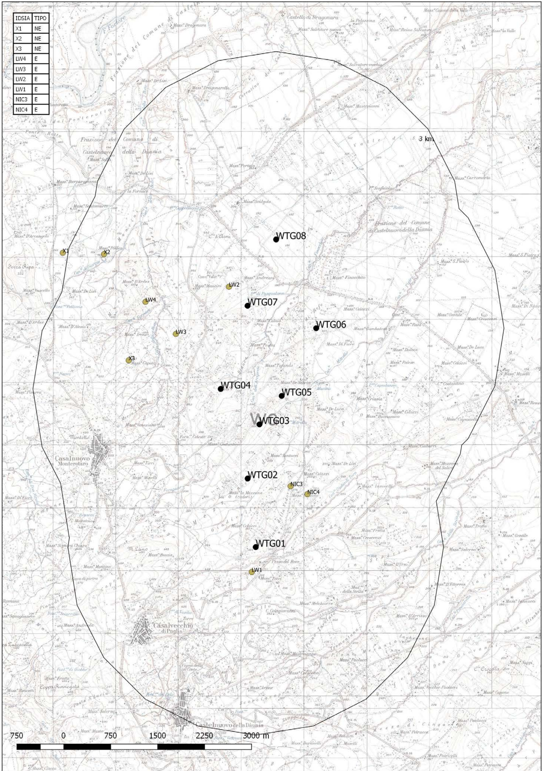
Impianti esistenti ed in fase di autorizzazione in un buffer di 3 km dalle WTG in progetto
