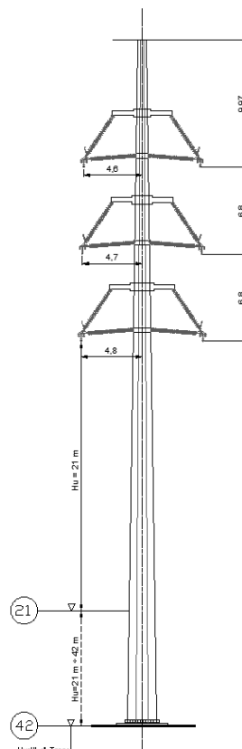
Schematico sostegno tubolare monostelo per linea doppia terna - sostegno di sospensione con armamento a mensola isolanti
