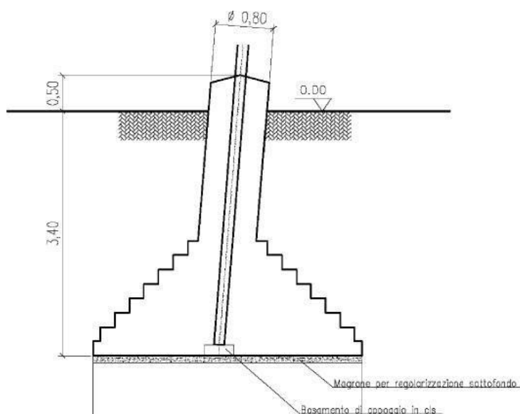
Figura 11 - Esempio di realizzazione di una fondazione a plinto con riseghe. Nell'immagine di sinistra di può osservare un disegno di progetto mentre nell'immagine di destra la fase di cassetatura della fondazione
