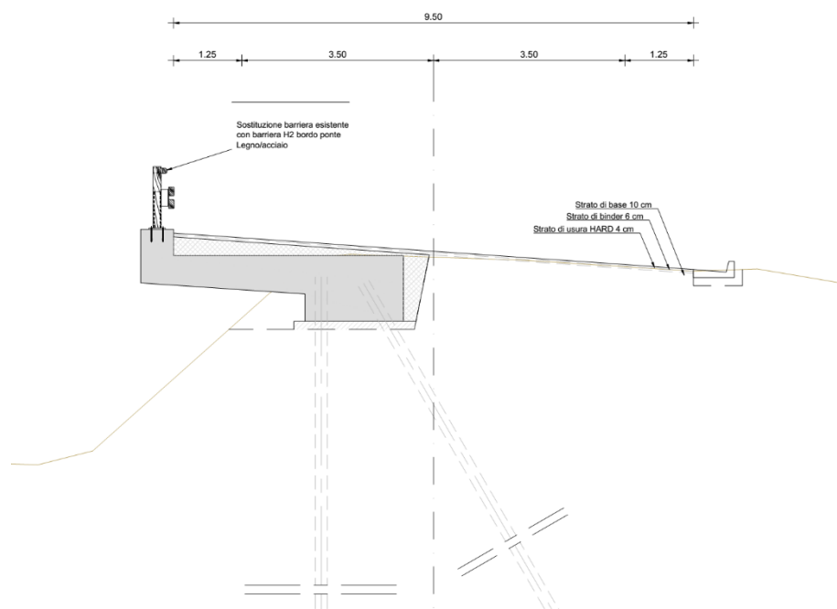
Sezione tipo con banchettone
