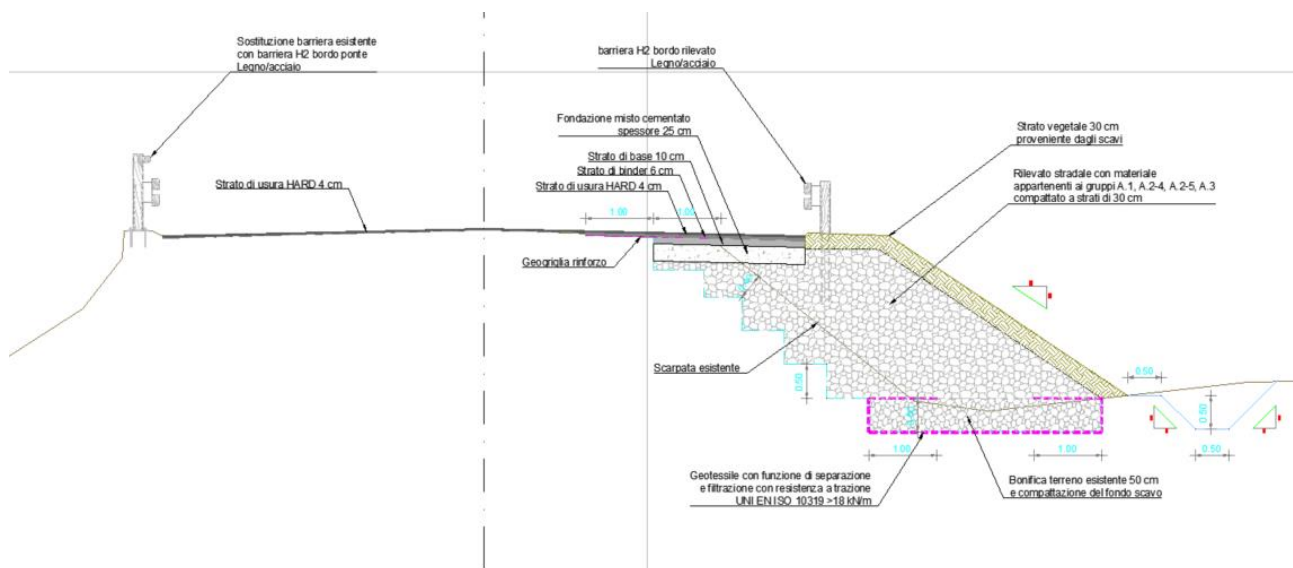
Sezione tipo con allargamento in rilevato.
