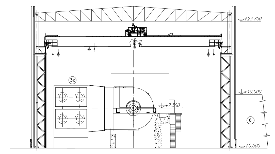
SEZIONE C-C
