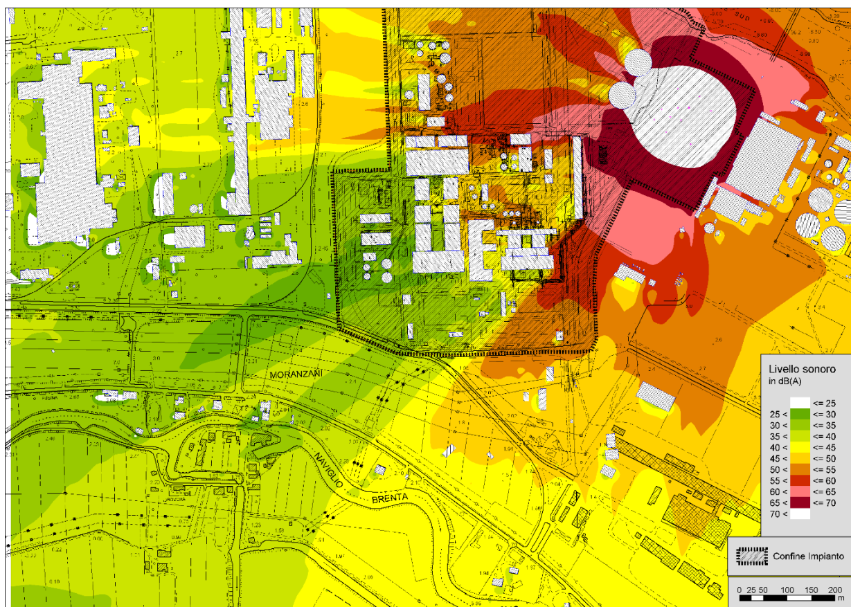
Figura 8 – C.le di Fusina - Cantiere per la realizzazione della nuova unità FS7 - Curve isofoniche di immissione specifica nell'area circostante all'altezza di 4 m dal suolo per la fase di preparazione del sito e scavi.
