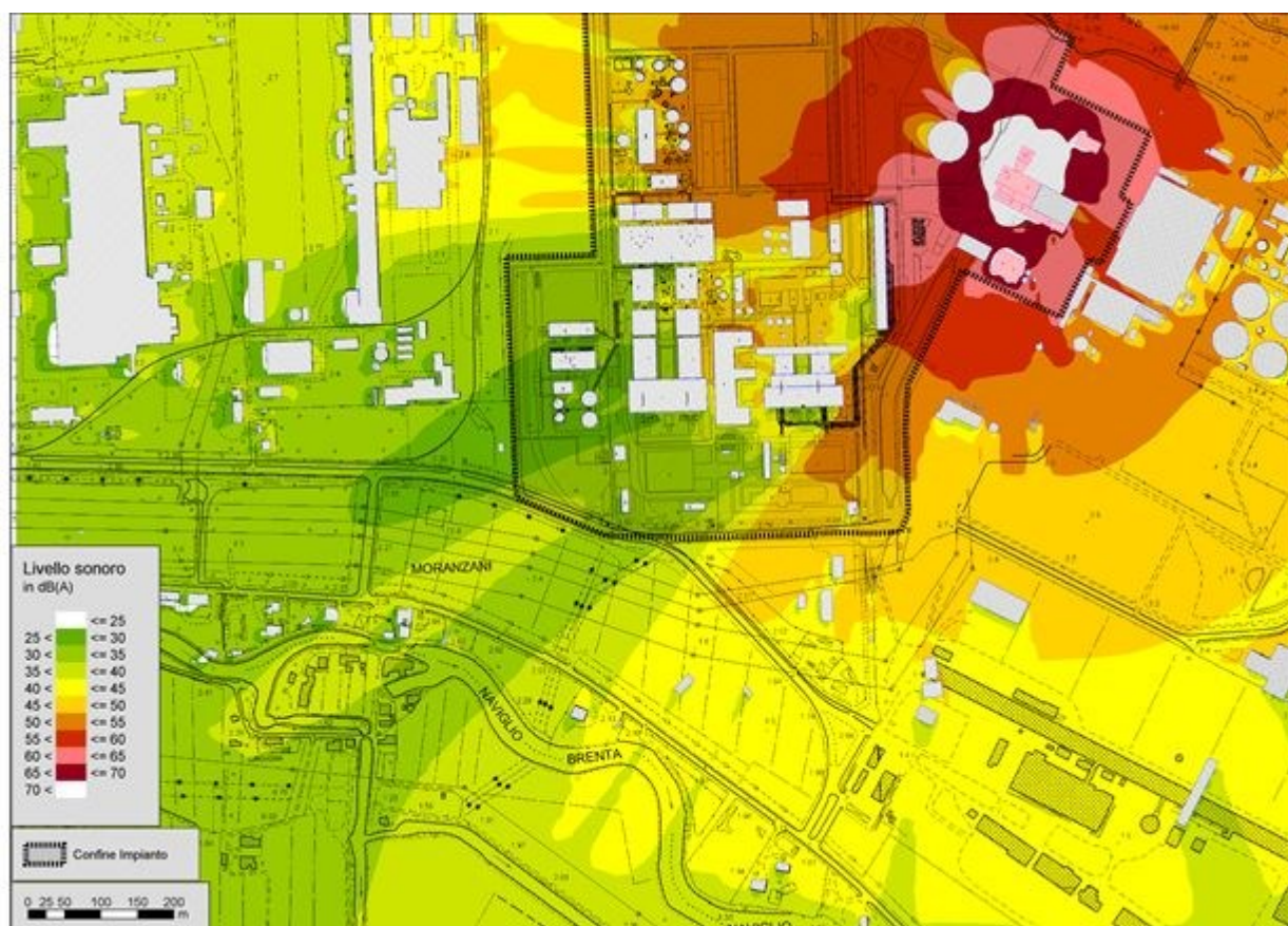
Figura 6-10 – livello sonoro senario futuro (fase 1)
