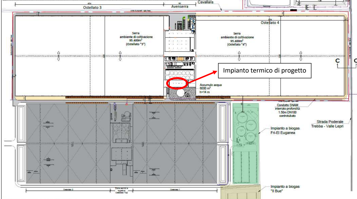
PLANIMETRIA GENERALE STATO DI PROGETTO Scala 1:1500
