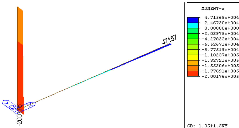
DIAGRAMMA MOMENTO FLETTENTE Mz (kgcm) - COMBINAZIONE 3 SLU 1.3*G+1.5*VY
