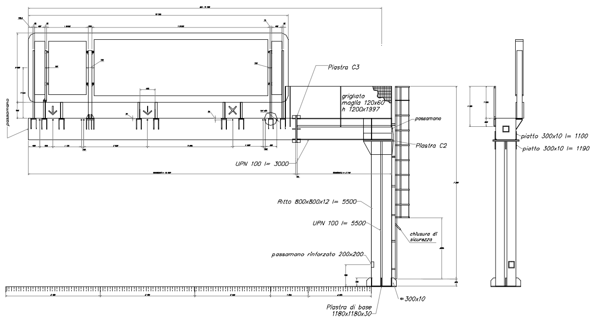
Schema portale
