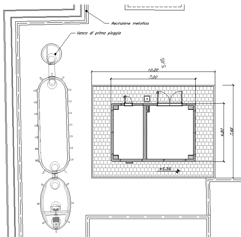
Figura 12 Stralcio planimetrico fabbricato tecnologico
