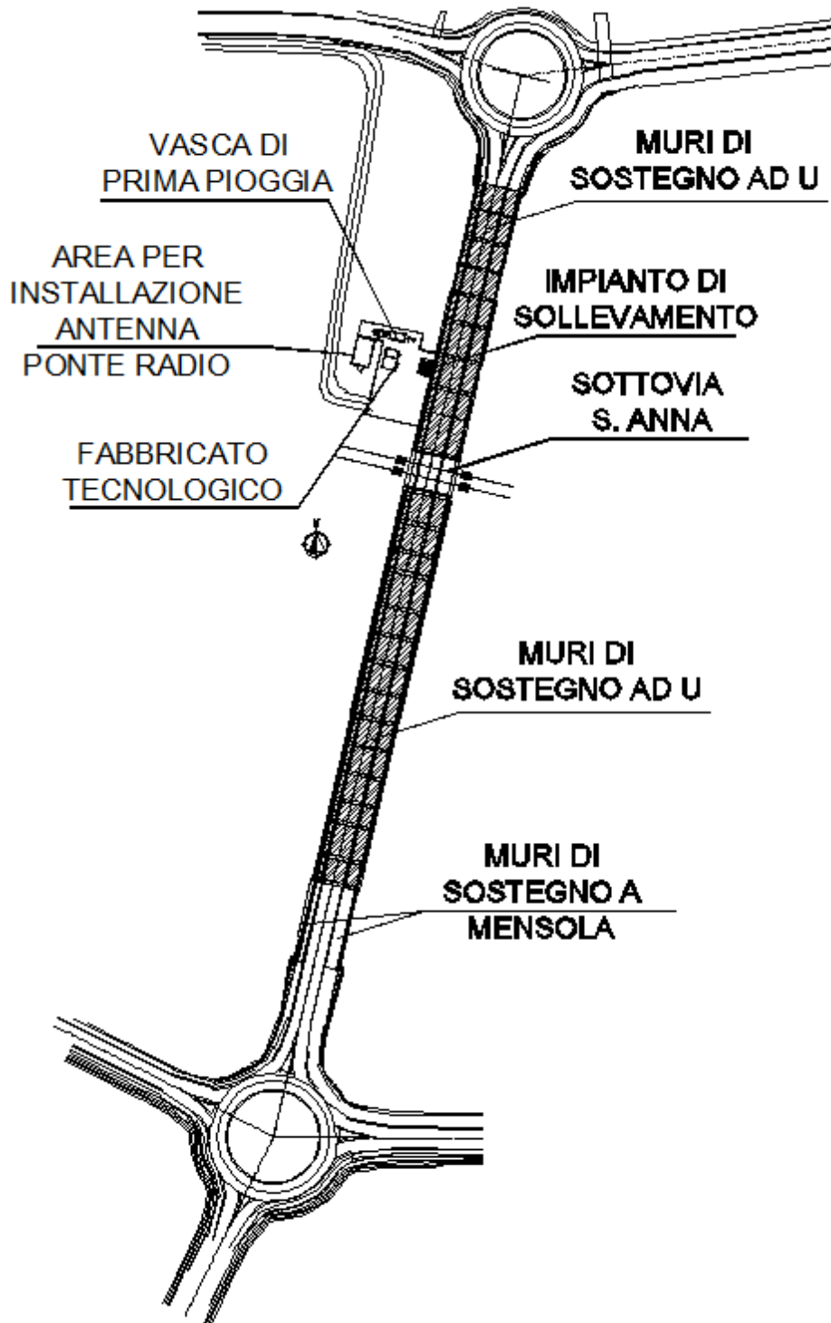
Figura 1 Inquadramento planimetrico
