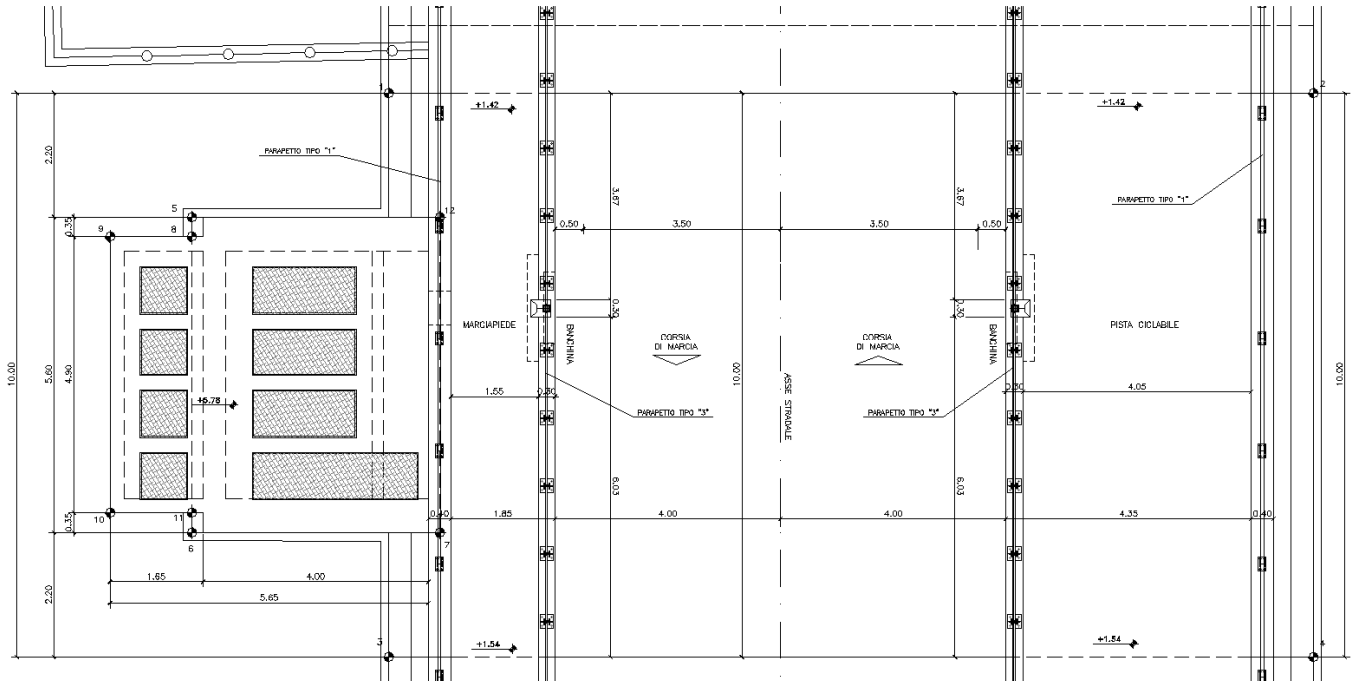
Figura 11 Vista dall'alto impianto di sollevamento
