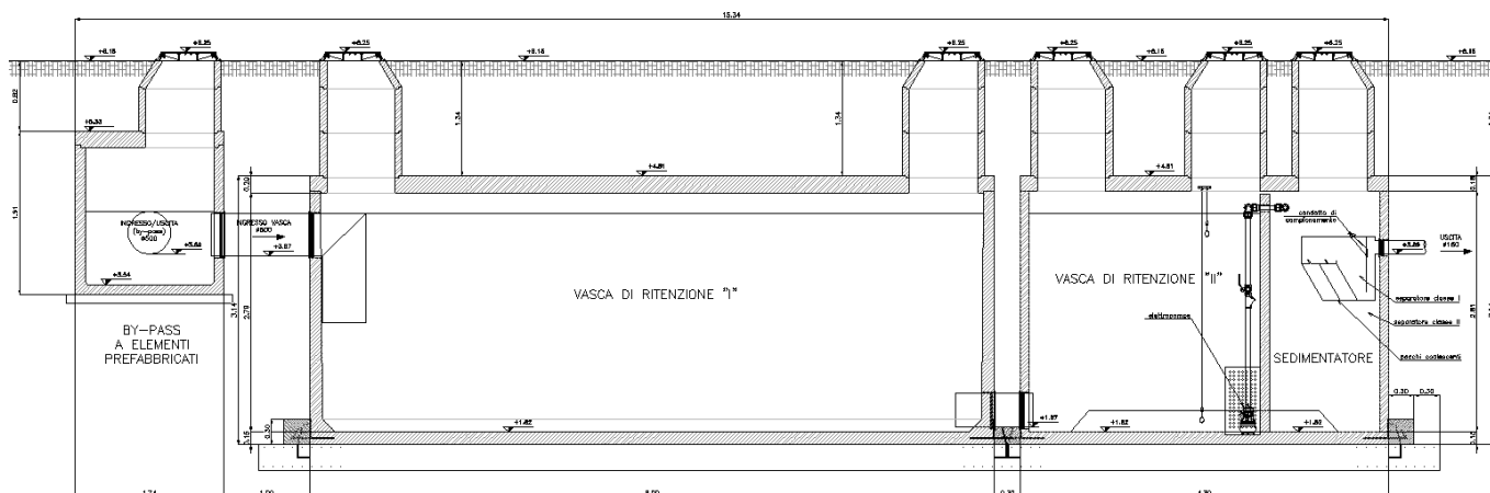
Figura 14 Sezione longitudinale fabbricato tecnologico
