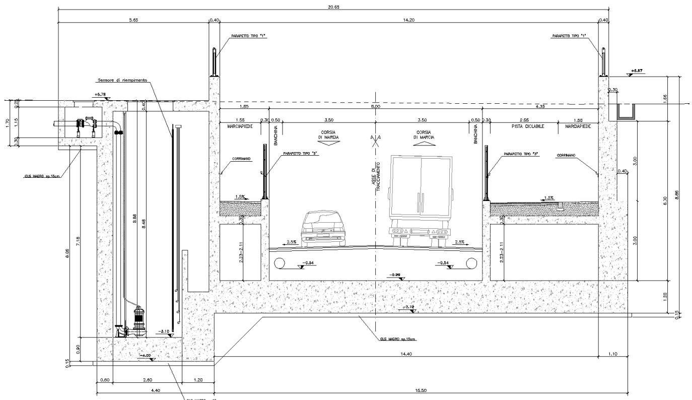
Figura 10 Sezione trasversale impianto di sollevamento
