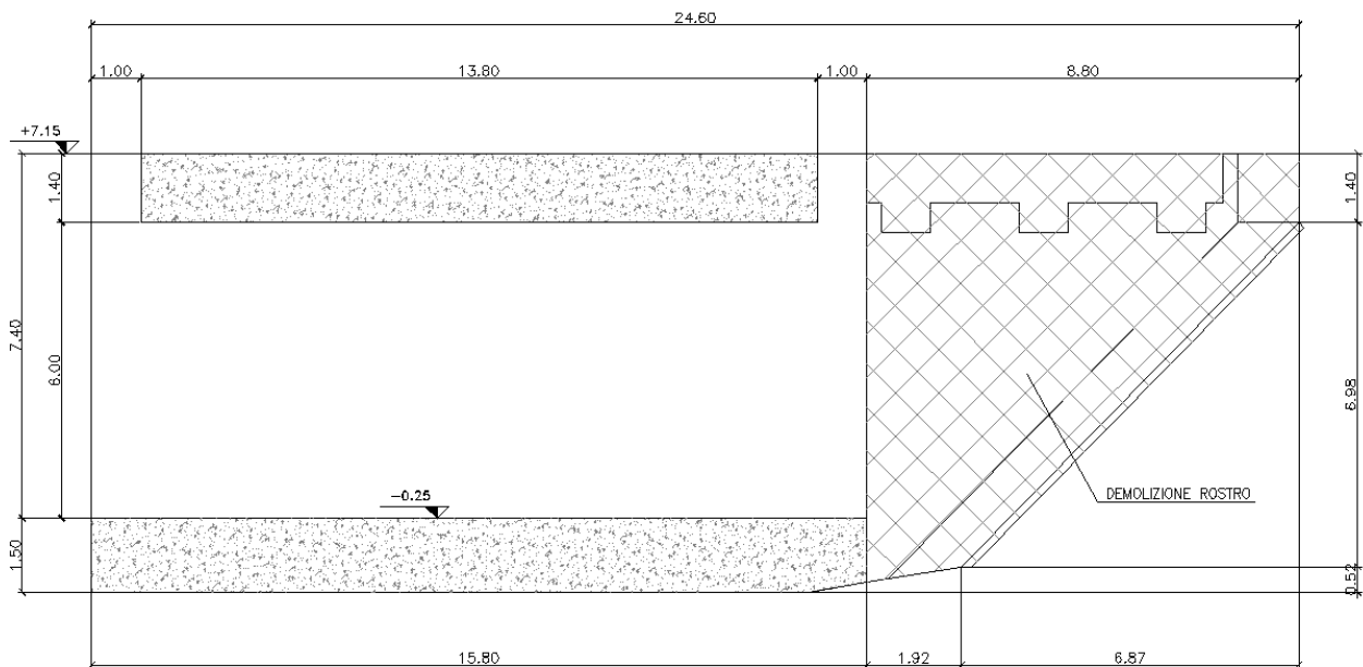
Figura 7 Sezione longitudinale monolite di spinta
