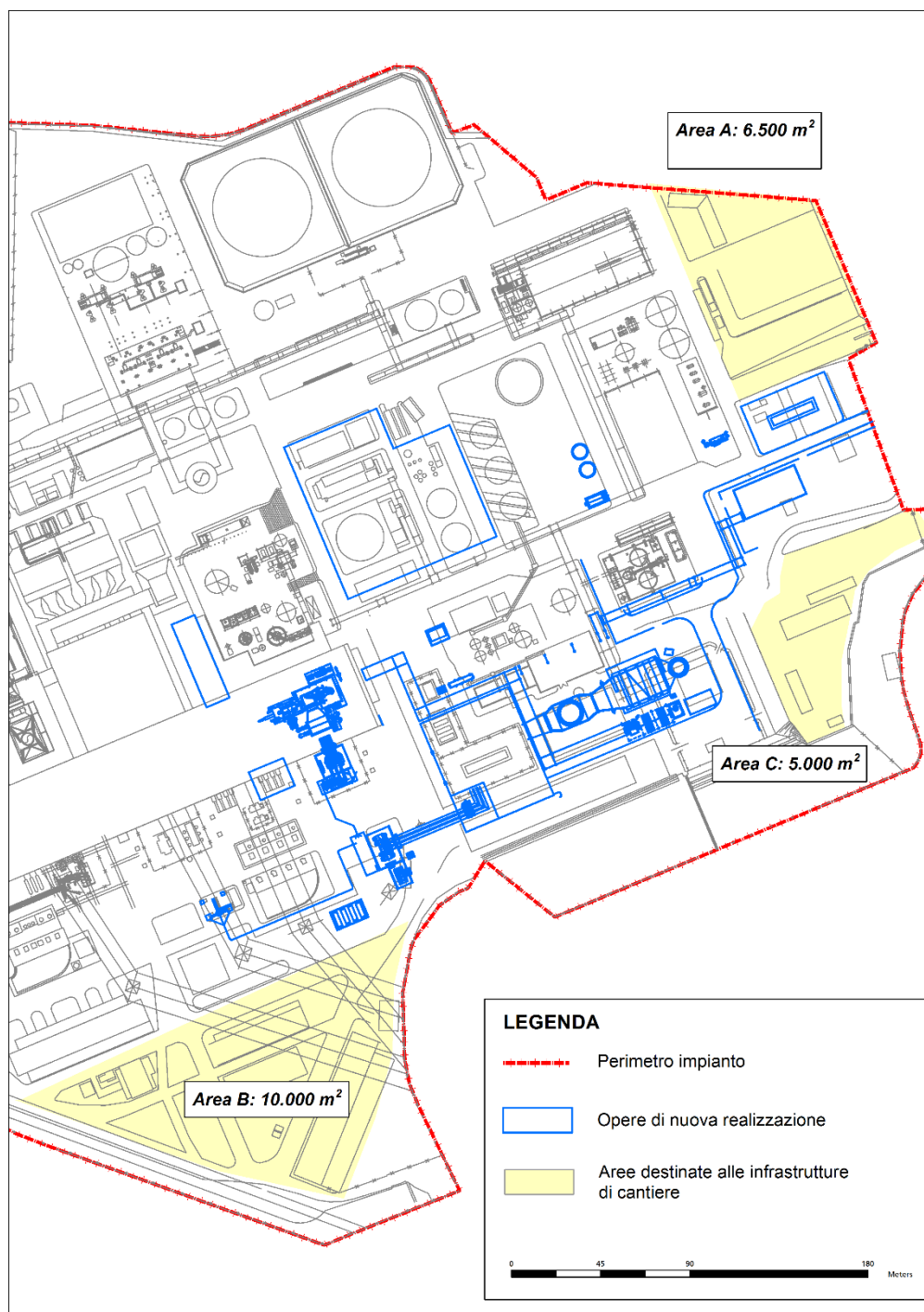
Figura 4.3 – Ubicazione delle aree destinate alle infrastrutture di cantiere
