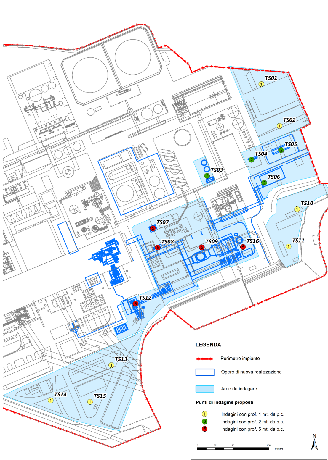
Figura 6.1 – Ubicazione dei punti di indagine proposti
