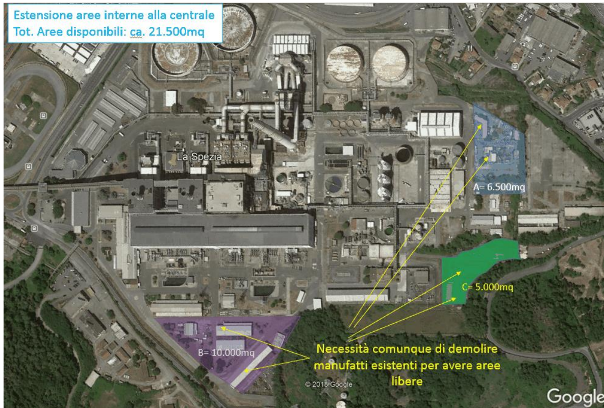
Figura 4.1 - Aree di cantiere interne al perimetro della Centrale
