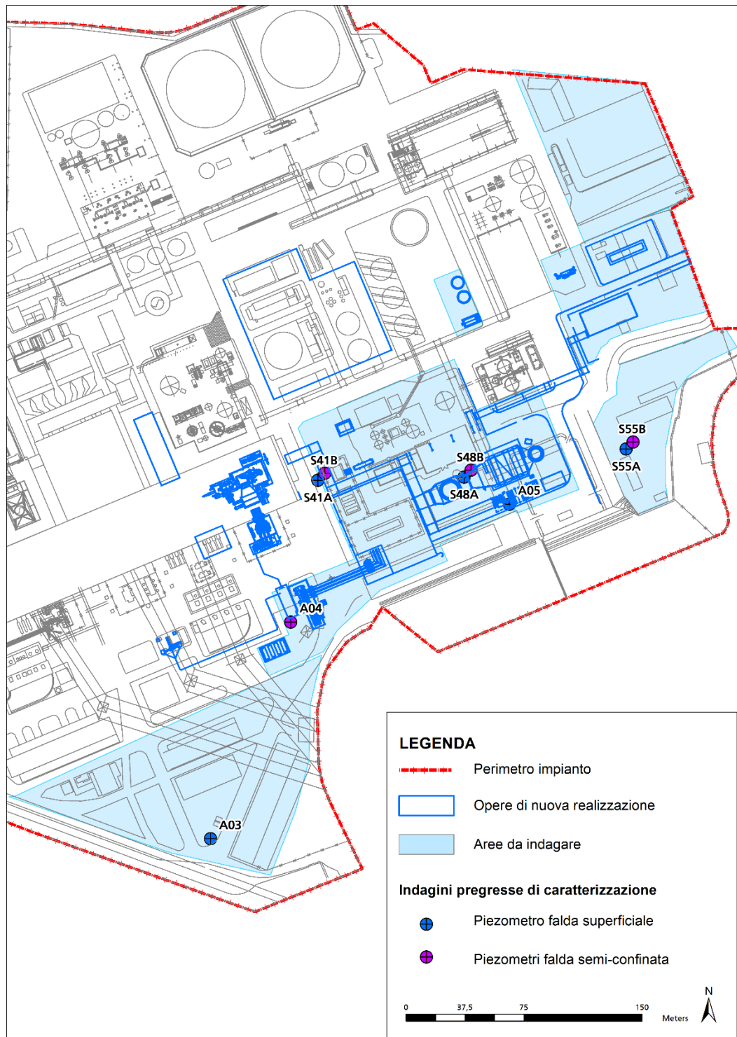
Figura 5.4 – Ubicazione dei piezometri nell’area di interesse
