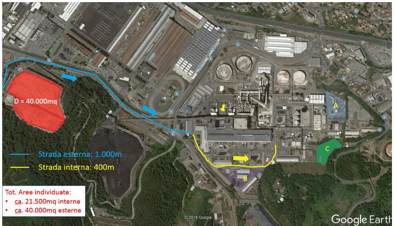
Figura 4.2 - Aree di cantiere
