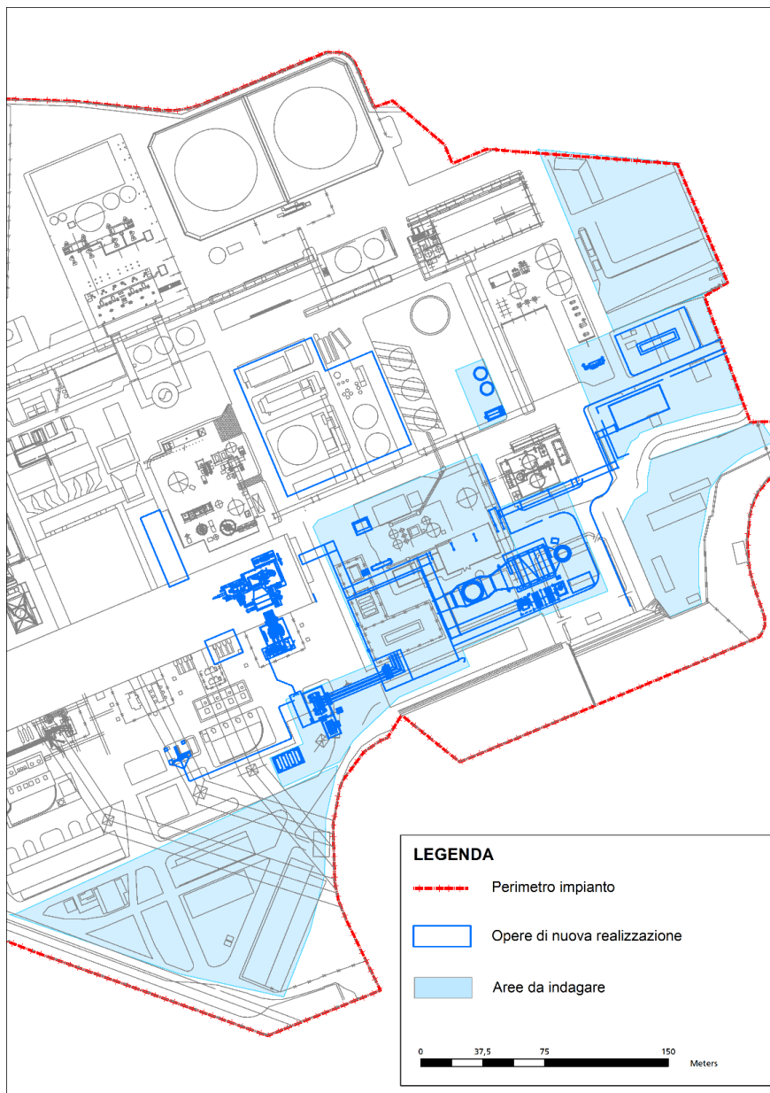
Figura 4.4 – Area da indagare
