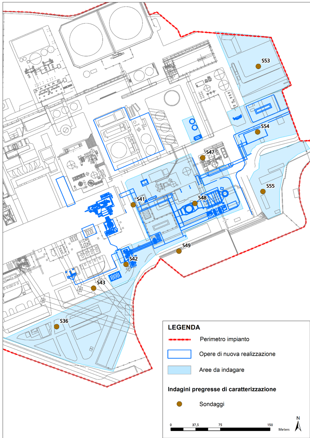
Figura 5.3 – Indagini pregresse: ubicazione dei sondaggi eseguiti per la caratterizzazione del sito
