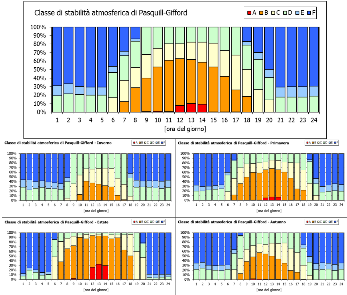
Figura 4.2.36 – Distribuzioni orarie della classe di stabilità atmosferica di Pasquill-Gifford calcolate su base annuale e stagionale. Periodo 2009-2013.
