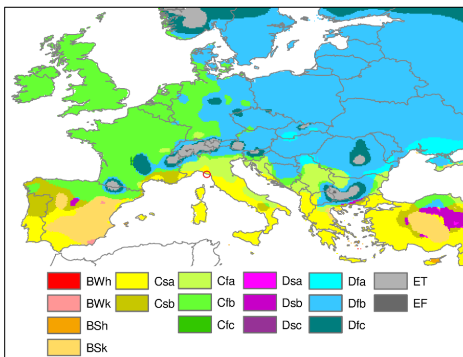
Figura 2.1.2 - Classificazione di Köppen Geiger
