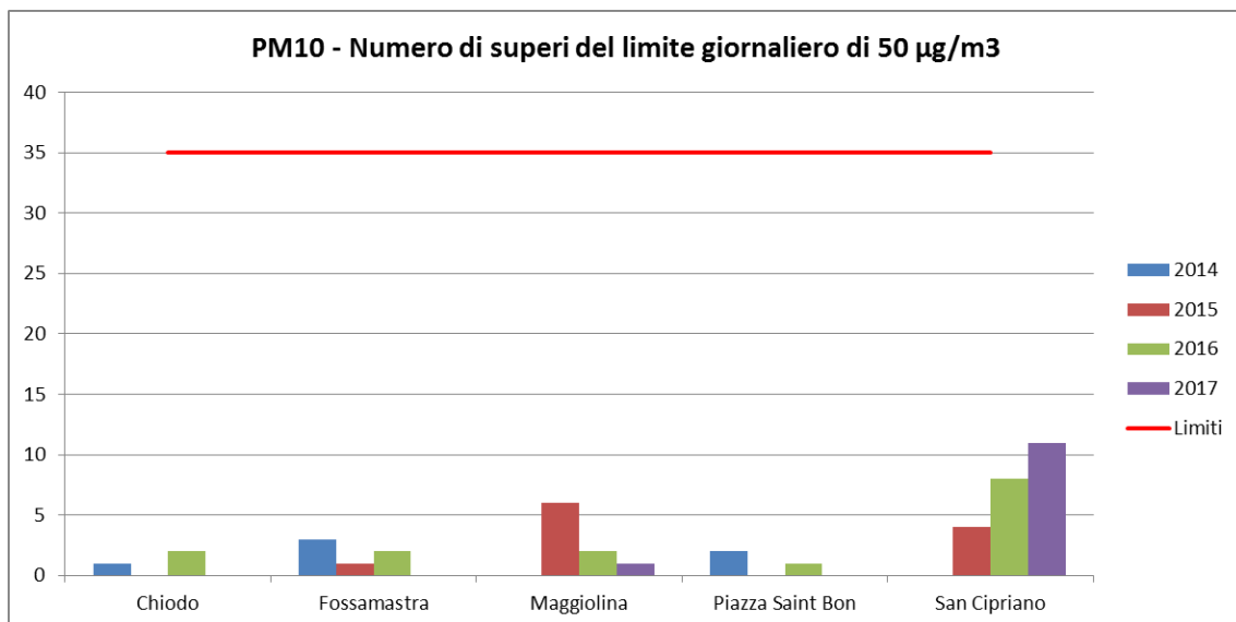
Figura 3.4.6 – Particolato PM 10 . Numero di superi del limite giornaliero di 50 µg/m³ nel quadriennio 2014-2017 nelle postazioni della rete di monitoraggio presenti nel Comune di La Spezia
