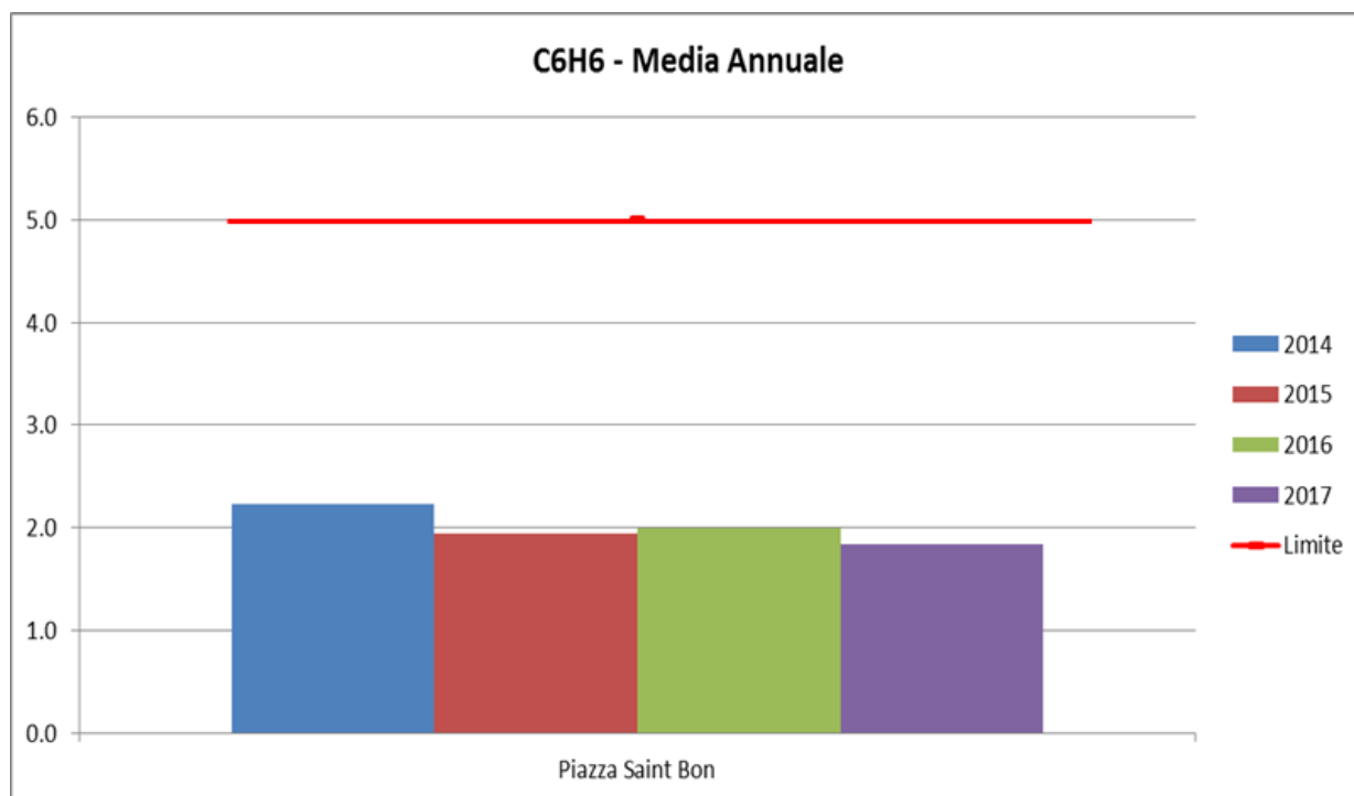
Figura 3.4.8 – Benzene. Medie annuali nel quadriennio 2014-2017 nella postazione della rete di monitoraggio presente nel Comune di La Spezia
