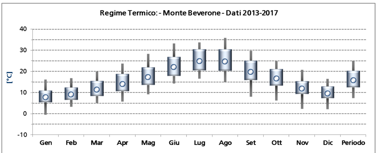
Figura 2.2.4 – Regime Termico nella stazione di Monte Beverone
