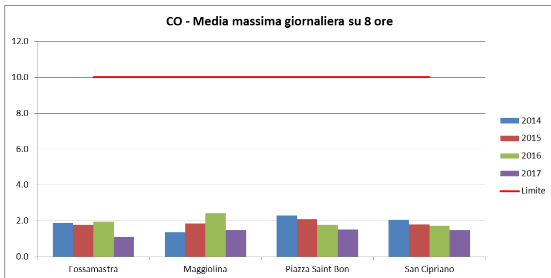
Figura 3.4.2 – Monossido di carbonio. Medie massime giornaliere su 8 ore nel quadriennio 2014-2017 nelle postazioni della rete di monitoraggio presenti nel Comune di La Spezia
