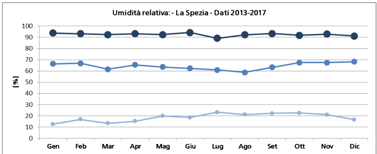
Figura 2.2.8 – Umidità relativa nella stazione di La Spezia
