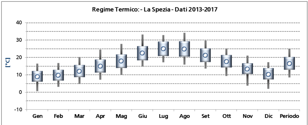
Figura 2.2.3 – Regime Termico nella stazione di La Spezia
