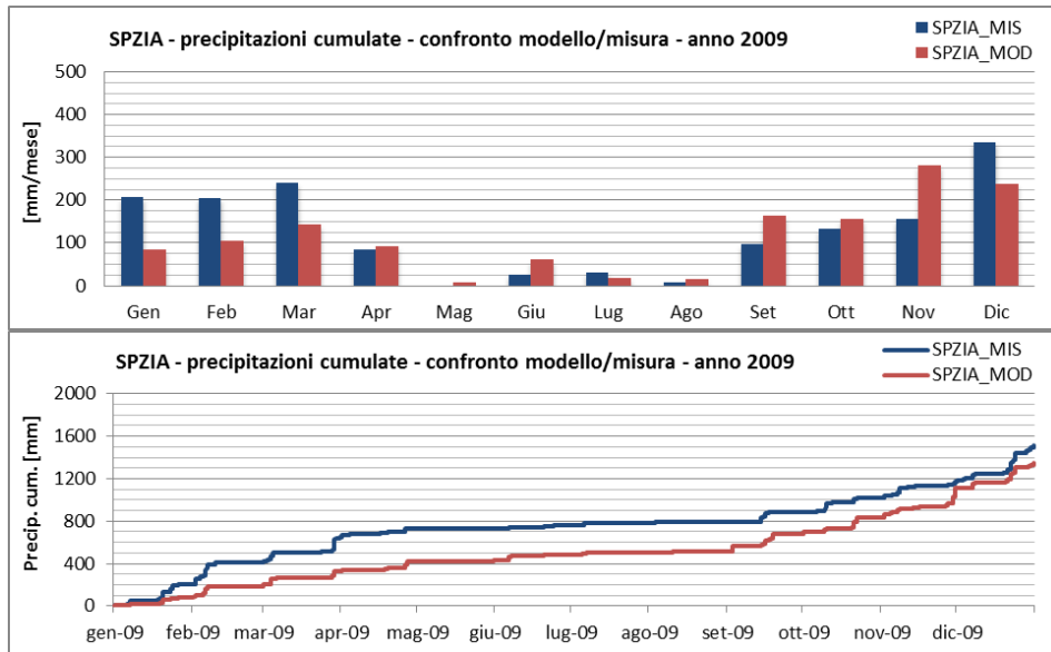
Figura 4.2.27 – Stazione meteo ARPAL La Spezia. Periodo 2009.
