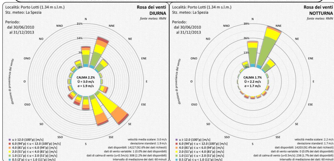
Figura 4.2.13 – Stazione meteo RMN La Spezia. Rose dei venti totale, diurna e notturna. Dati misurati nel periodo 30/06/2010-31/12/2013.
