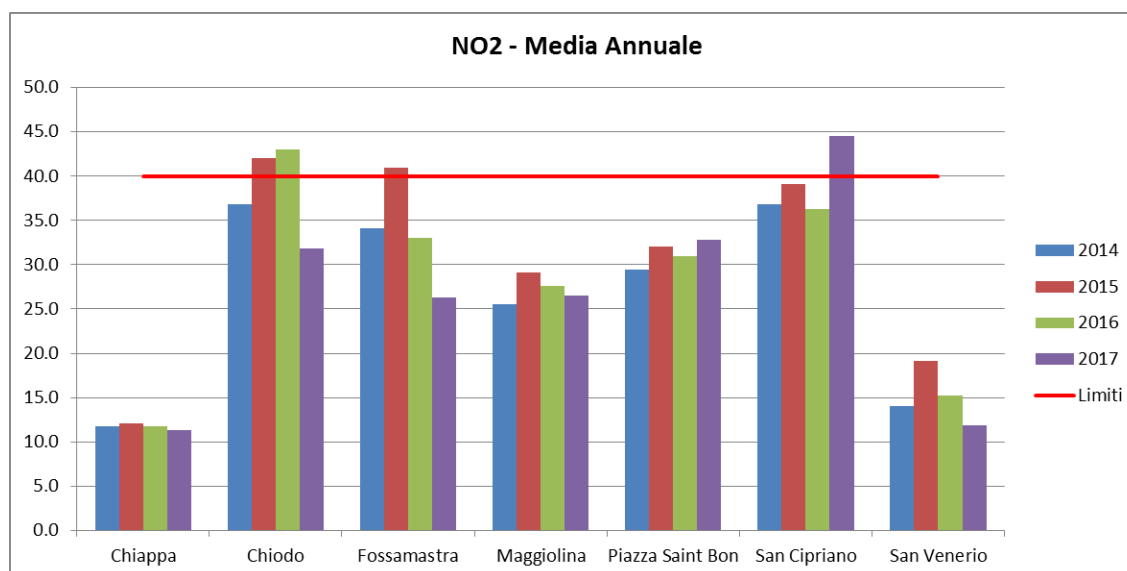
Figura 3.4.3 – Biossido di azoto. Medie annuali nel quadriennio 2014-2017 nelle postazioni della rete di monitoraggio presenti nel Comune di La Spezia
