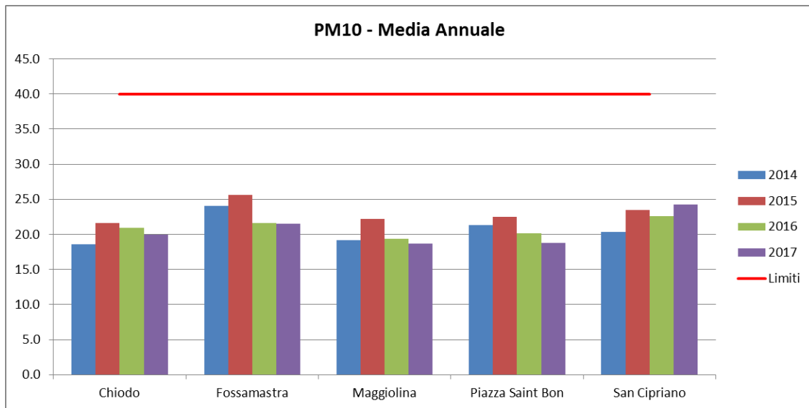
Figura 3.4.5 – Particolato PM 10 . Medie annuali nel quadriennio 2014-2017 nelle postazioni della rete di monitoraggio presenti nel Comune di La Spezia
