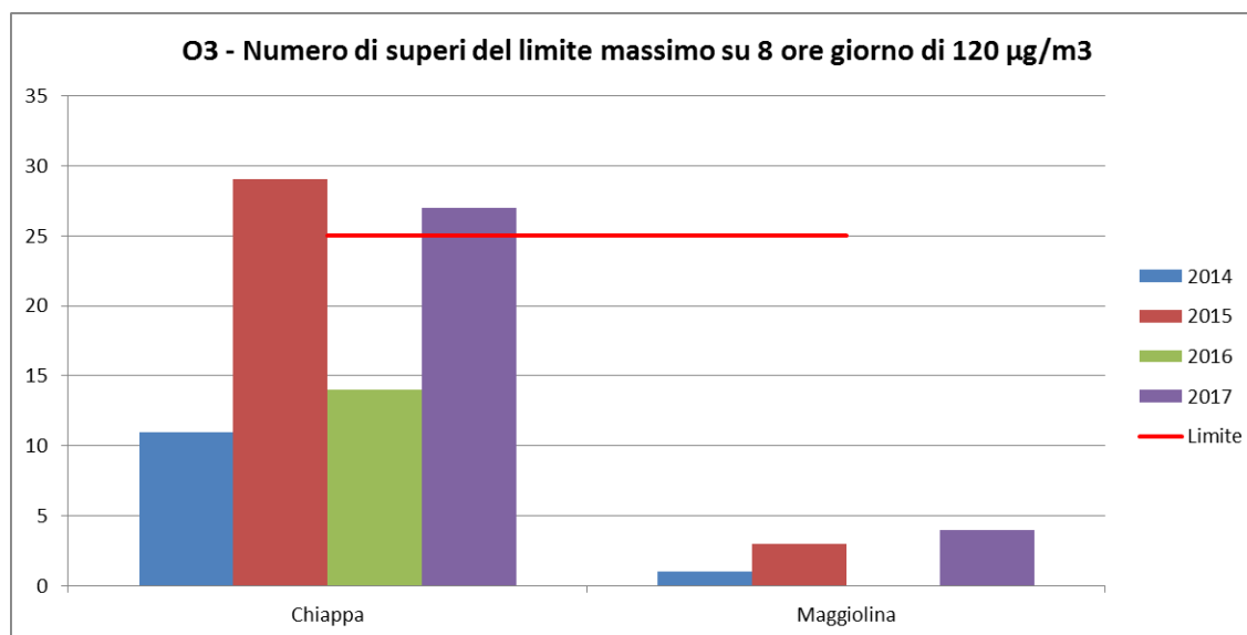
Figura 3.4.4 – Ozono. Numero di superi del limite massimo su 8 ore giorno di 120 µg/m 3 nel quadriennio 2014-2017 nelle postazioni della rete di monitoraggio presenti nel Comune di La Spezia
