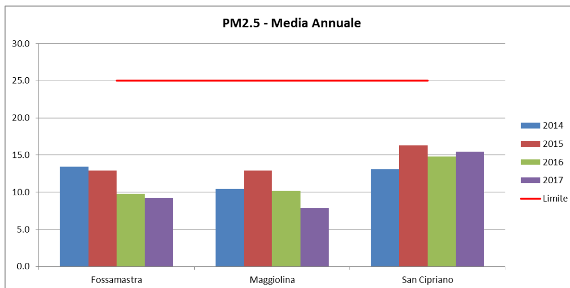
Figura 3.4.7 – Particolato PM 2.5 . Medie annuali nel quadriennio 2014-2017 nelle postazioni della rete di monitoraggio presenti nel Comune di La Spezia
