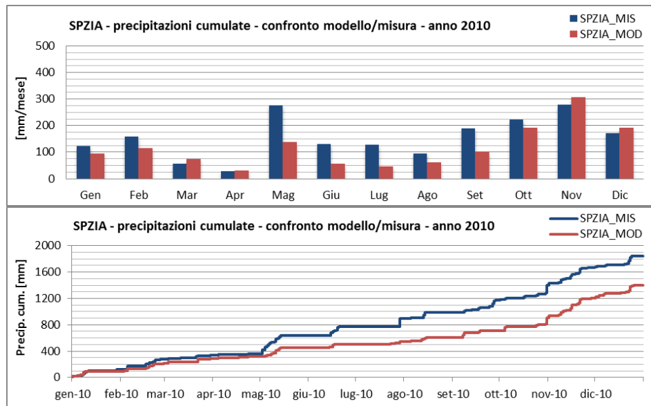
Figura 4.2.29 – Stazione meteo ARPAL La Spezia. Periodo 2010. Confronto tra misure e modello delle precipitazioni mensili e cumulate nell'anno.
