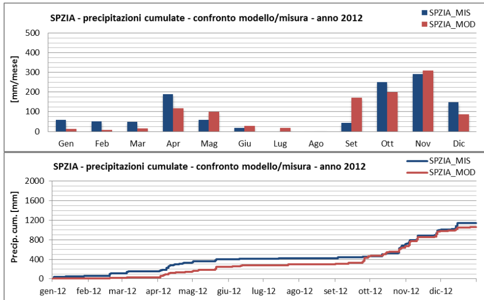
Figura 4.2.33 – Stazione meteo ARPAL La Spezia. Periodo 2012. Confronto tra misure e modello delle precipitazioni mensili e cumulate nell'anno.
