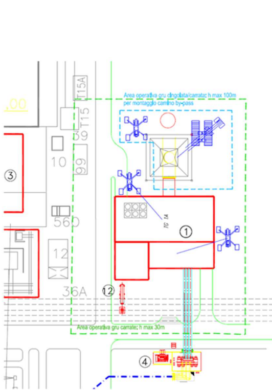
Fase 1 (OCGT)
