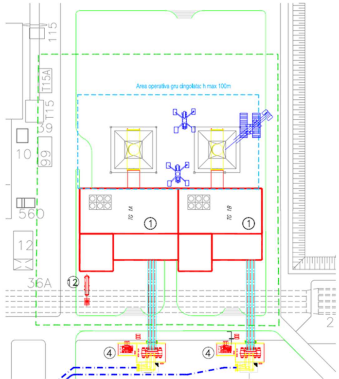
Fase 2 (OCGT)
