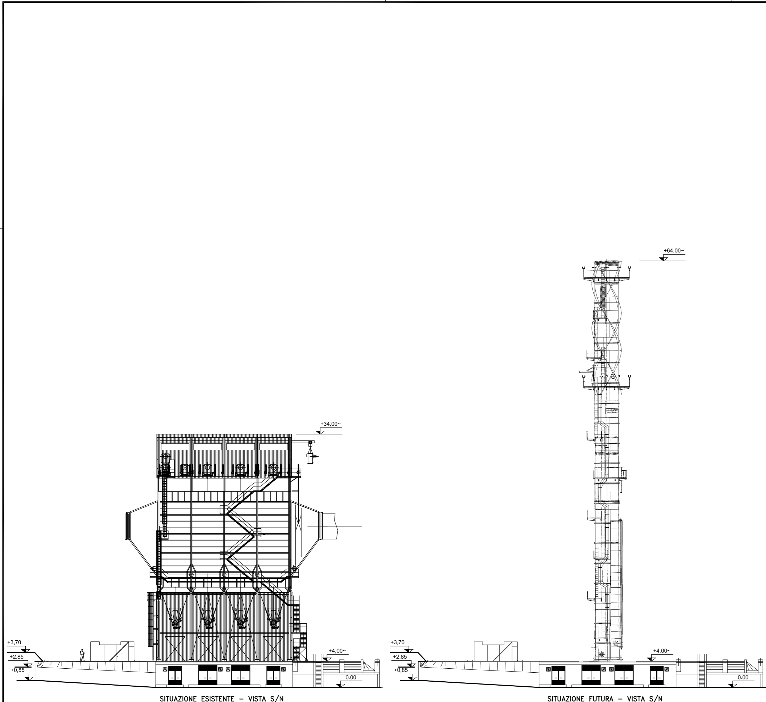
SITUAZIONE ESISTENTE - VISTA S/N
