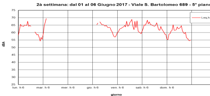
Grafico 2: Andamento temporale del LA_{eq,h} , presso abitazione Fam. Arduini dal 01 al 06 Giugno 2017
