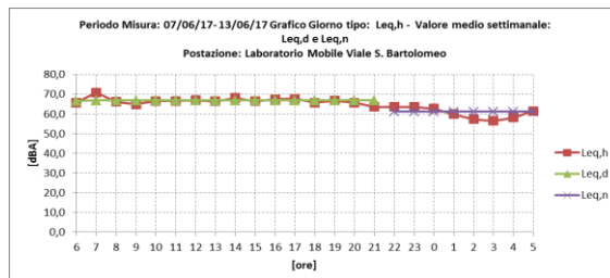
Grafico 10: Andamento temporale del L_{Aeq,h} della “giornata tipo” e valori medi L_{Aeq,TR} presso Lab. mobile dal 07 giugno al 13 Giugno 2017
