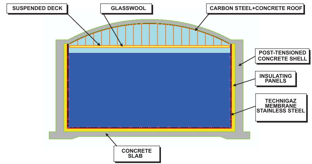
SERBATOIO A MEMBRANA
