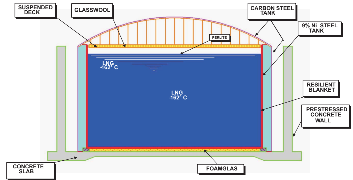
SERBATOIO A DOPPIO CONTENIMENTO
