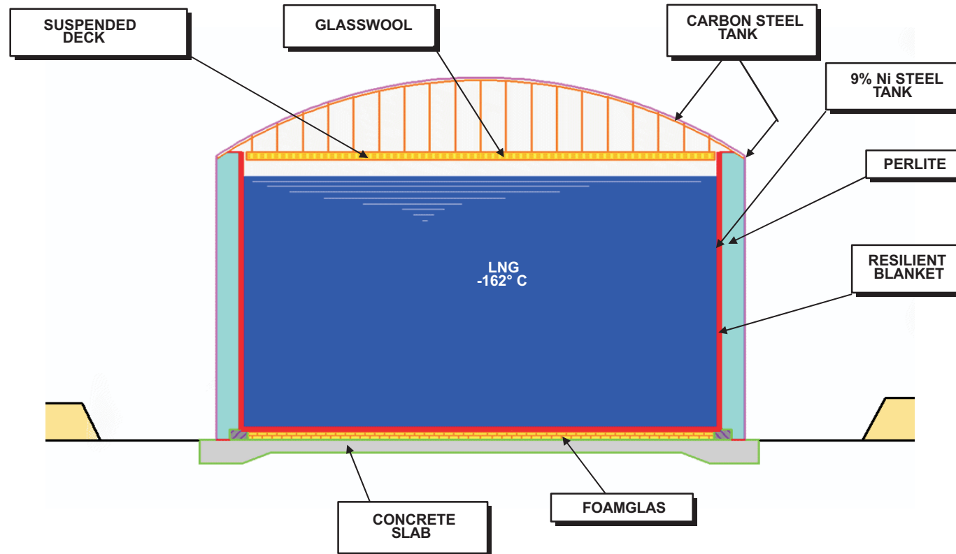
SERBATOIO A CONTENIMENTO SINGOLO
