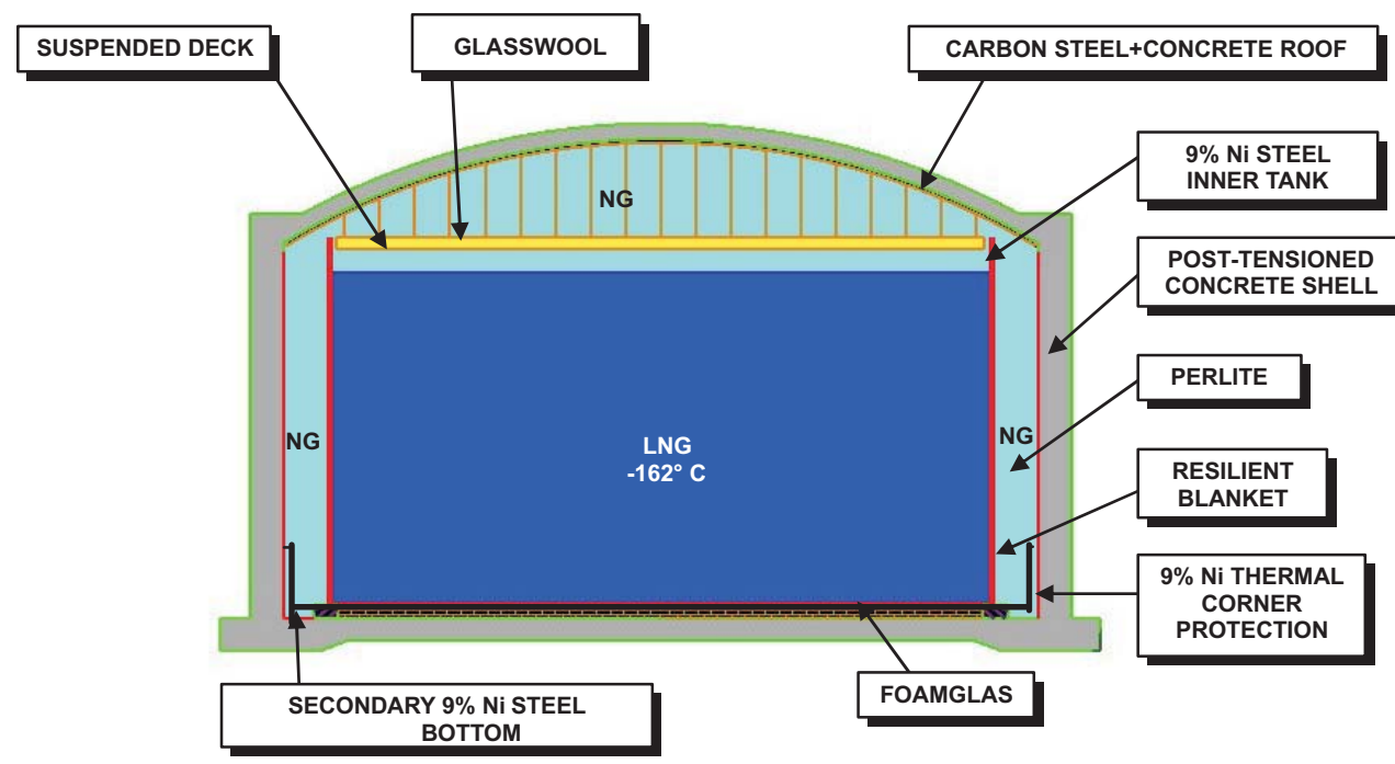
SERBATOIO A PIENO CONTENIMENTO (FULL CONTAINEMENT)
