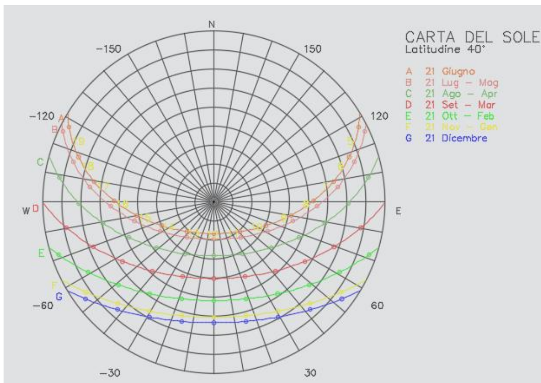
Fig. 2 - traiettorie solari - Carta del Sole Lat. 40
