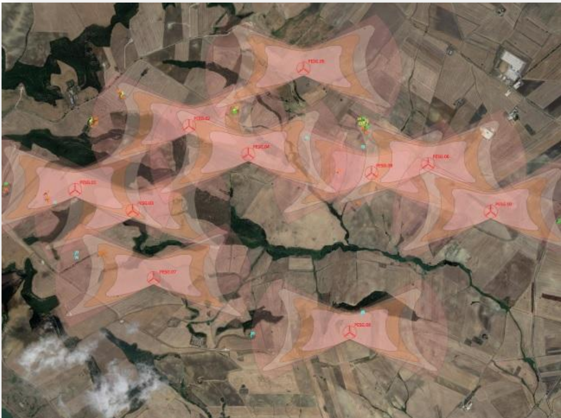
Figura 4. Analisi degli effetti dello shadow flickering su ortofoto
