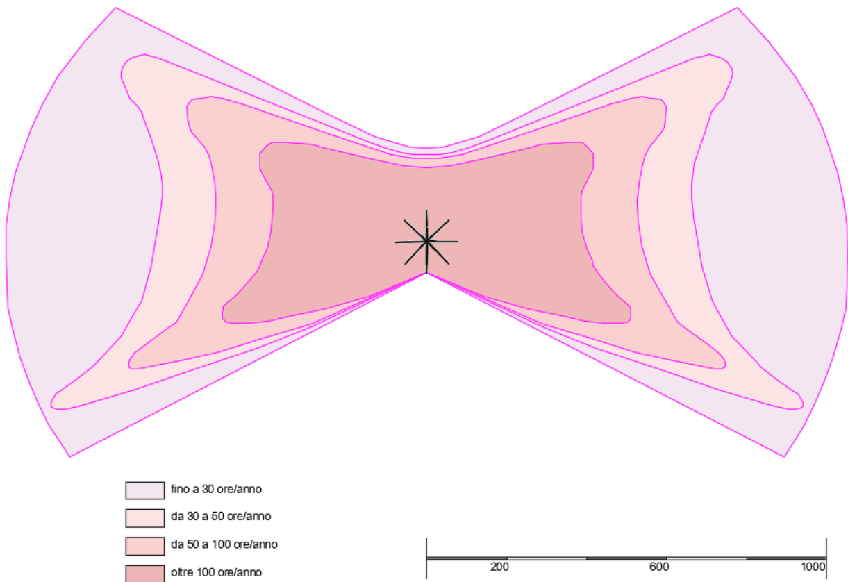
Fig. 3 - evoluzione effetto shadow flickering annuale - Carta del Sole Lat. 40 - turbina H = 112+75 = 187 m
