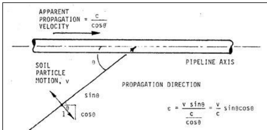
Figura 3.4.2 Effetto longitudinale delle onde di taglio sul tubo (ASCE, 1984 - Appendice B).
