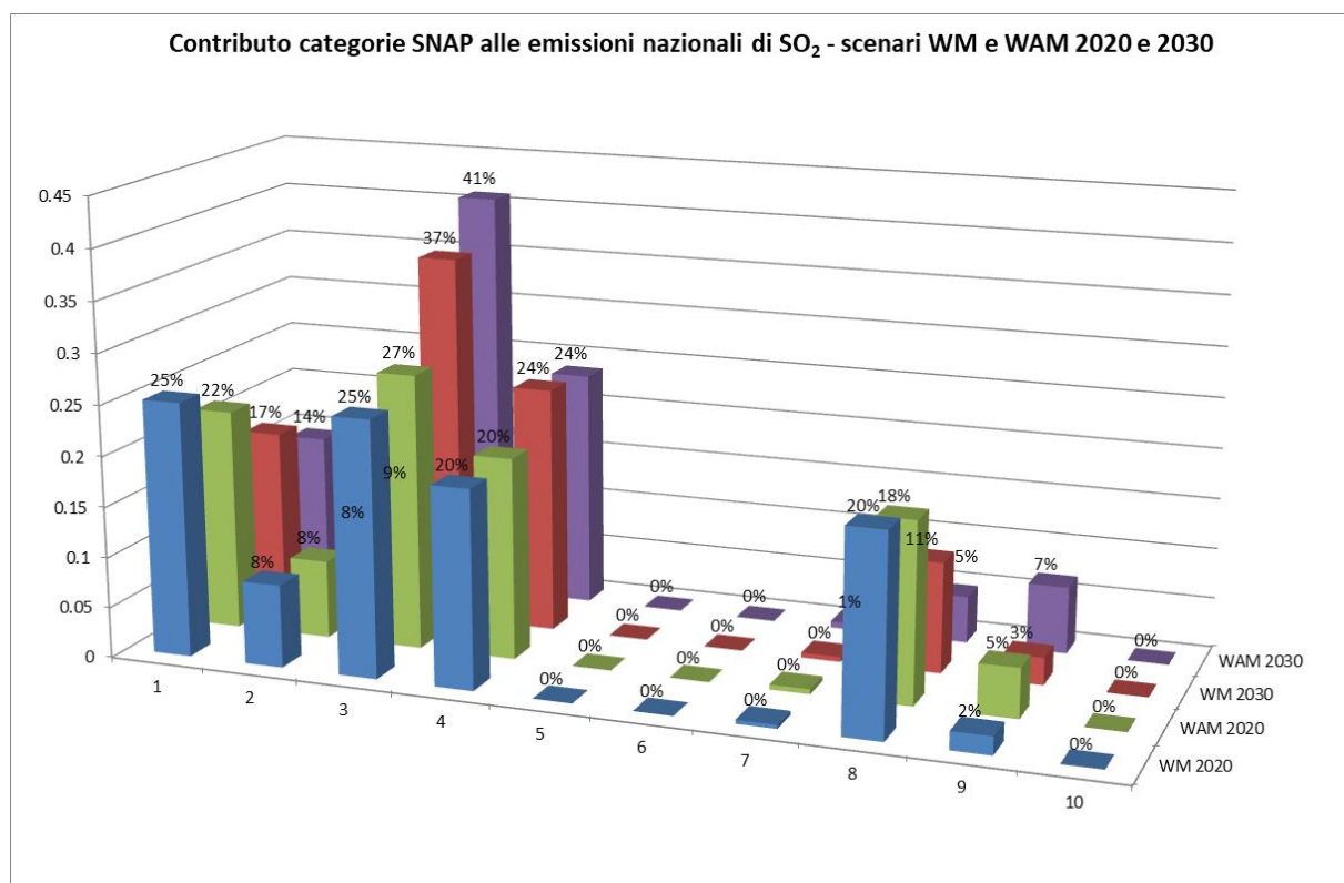
Figura A1 – Contributo (in %) delle macro categorie SNAP alle emissioni totali nazionali di SO 2 per gli scenari WM e WAM per gli anni 2020 e 2030.
