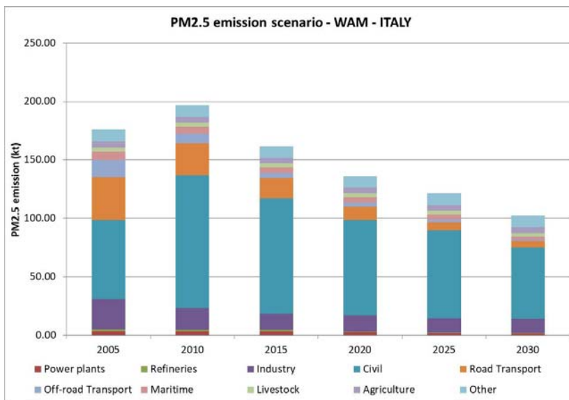
Figura 37 – Scenario nazionale WM (in alto) e WAM (in basso) per le emissioni PM_{2,5} per settore elaborato con il modello GAINS-Italia per gli anni 2005-2030.
