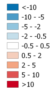
Figura 60 – 2020 WM, PM 10 , 36° valore più elevato sulla serie temporale dei valori giornalieri. Differenza rispetto all'anno base.
