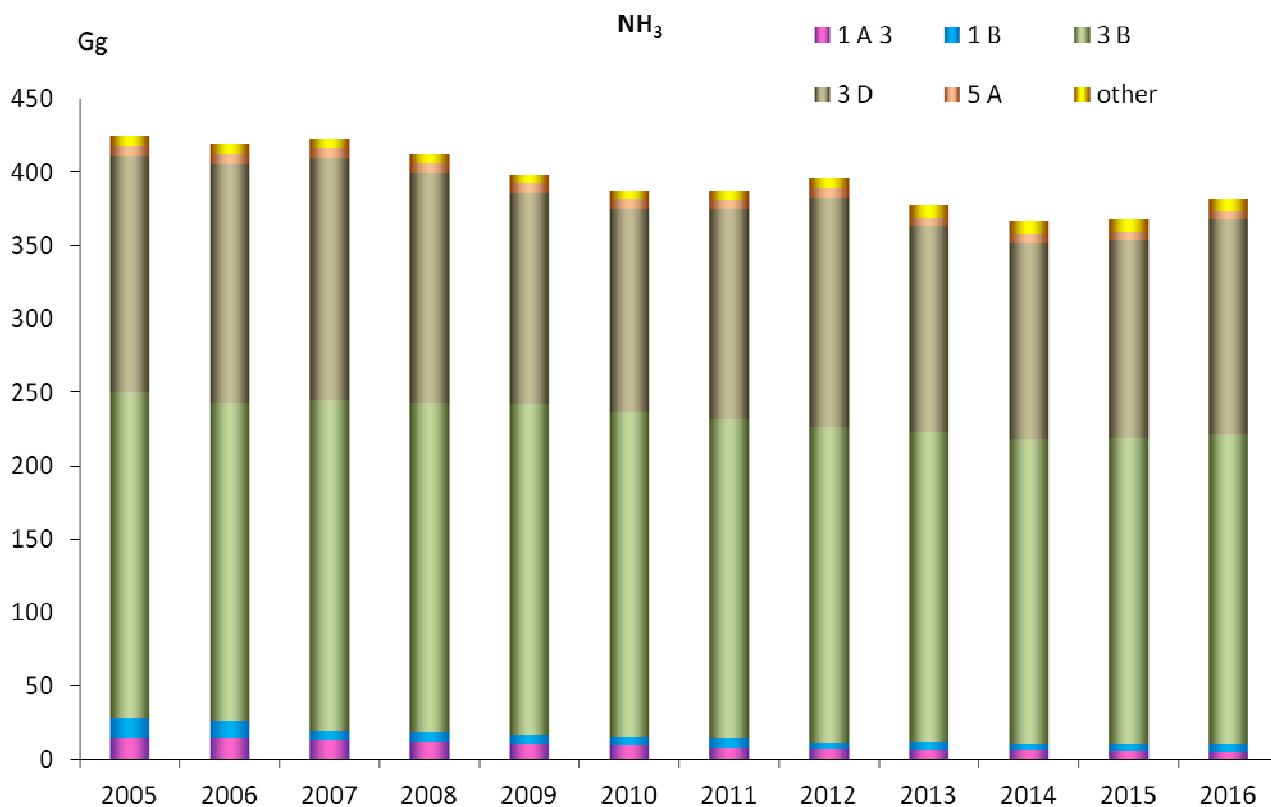
Figura 4 – Andamento delle emissioni di ammoniaca, categorie NFR
