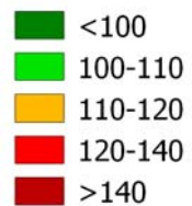
Figura 68 – 2020 WAM, O 3 , 26° valore più elevato sulla serie temporale dei massimi giornalieri delle medie mobili su 8 ore. Differenza rispetto all'anno base.
