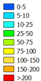
Figura 58 – 2020 WM, NO 2 , 19° valore più elevato sulla serie temporale dei valori orari. Differenza rispetto all'anno base.
