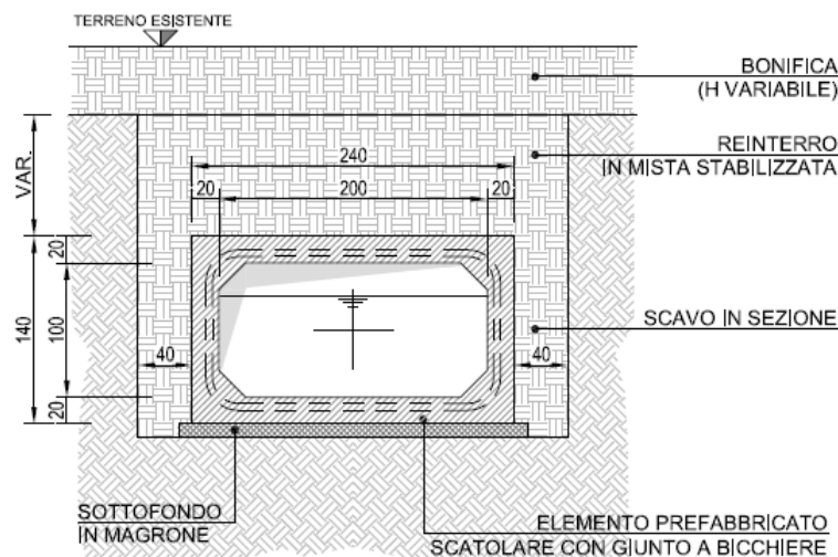
Sezione trasversale
