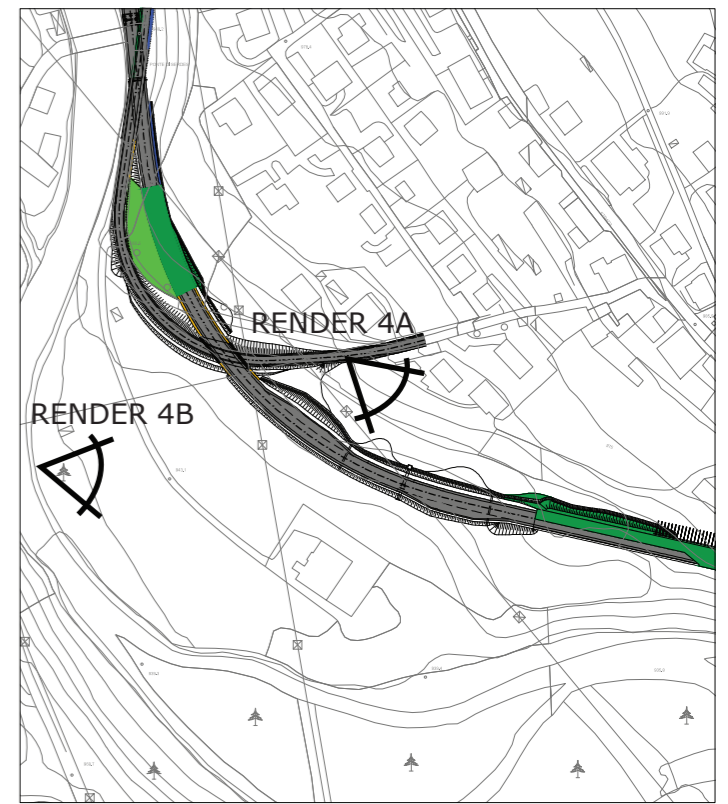
PLANIMETRIA D'INQUADRAMENTO
