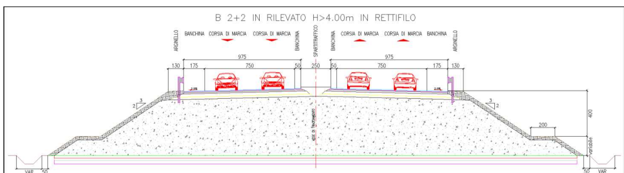
FIGURA 1-7 - SEZIONE TIPO CATEGORIA B
