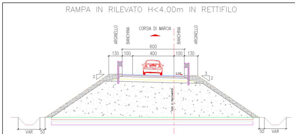
FIGURA 1-9 - SEZIONE TIPO RAMPA DI SVINCOLO
