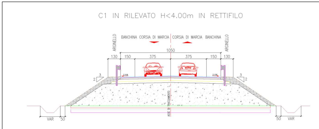
FIGURA 1-8 - SEZIONE TIPO CATEGORIA C1
