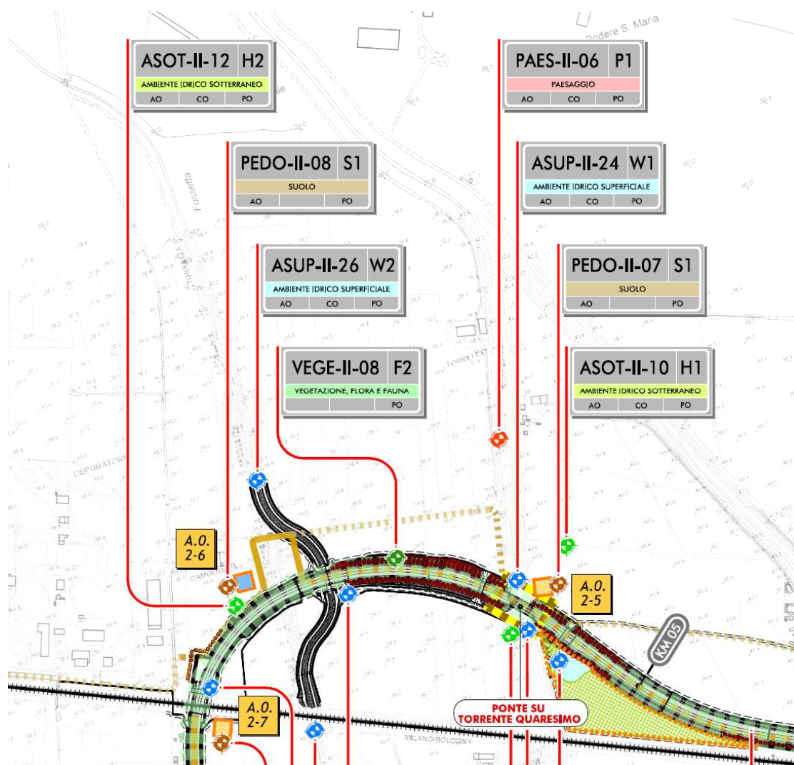
FIGURA 4-3– STRALCIO PLANIMETRICO CON LA LOCALIZZAZIONE DEI PUNTI DI MONITORAGGIO
