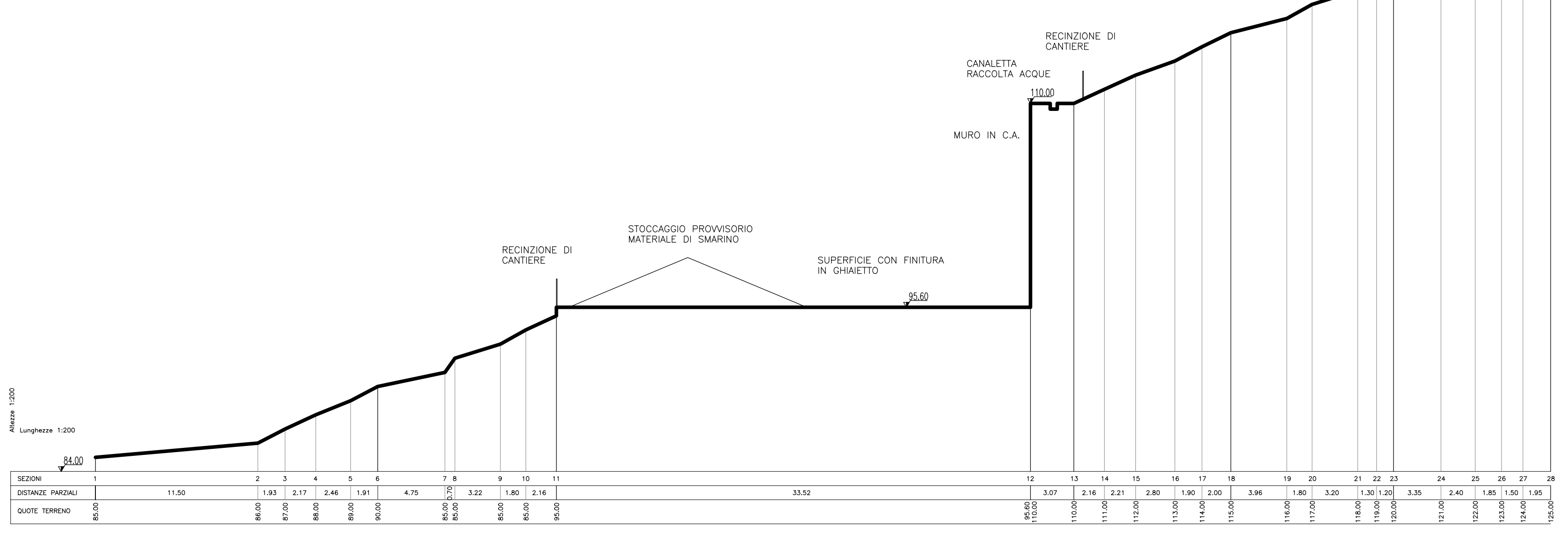
SEZIONE E-E SCALA 1:200
