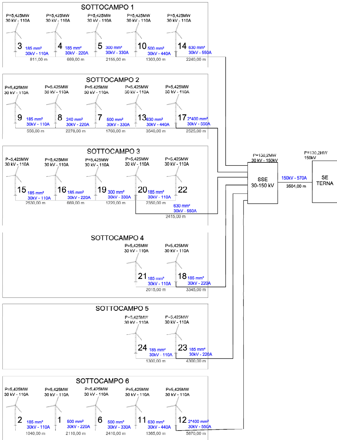
Schema a blocchi Parco Eolico
