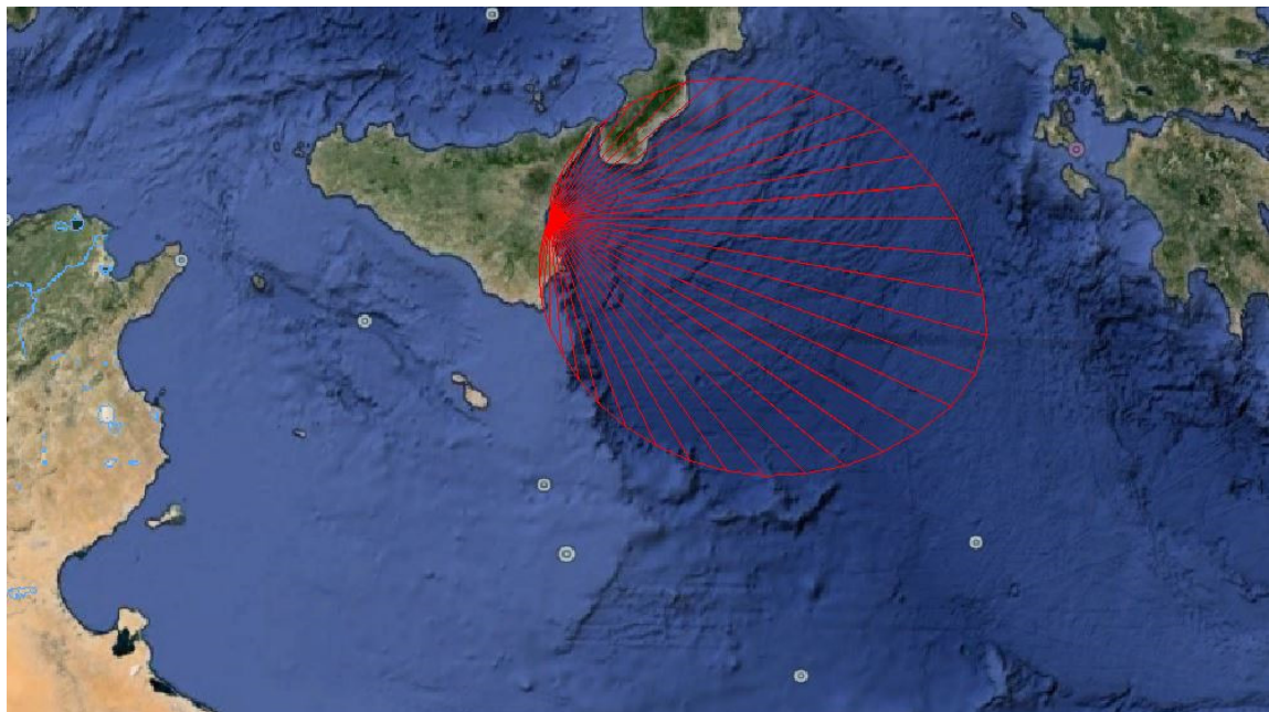
Figura 8: Tracciamento dei fetch efficaci per il paraggio di Catania
