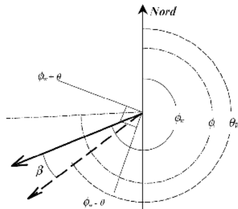
Figura 10: Schema di riferimento, convenzioni e simboli relativi alle direzioni del vento e del moto ondoso
