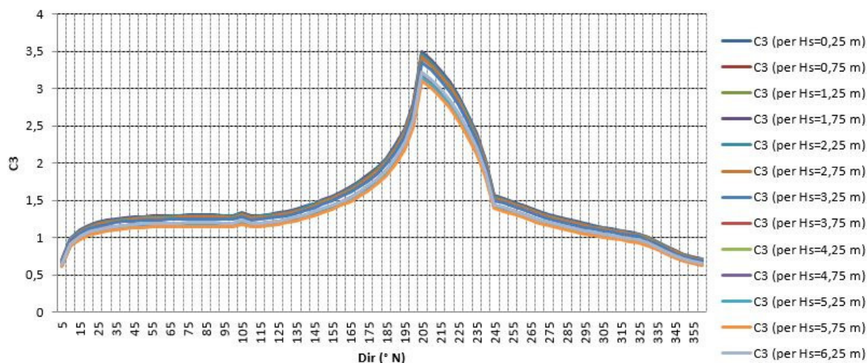
Figura 9bis: Coefficiente di trasposizione C3 in funzione della direzione di provenienza del moto ondoso (da Catania ad Avola). Nel calcolo del coefficiente C3, il rapporto T_p/T_m è stato determinato sulla base delle curve di regressione H_s-T_m e H_s-T_p per la boa reale di Catania (vedi capitolo relativo alle correlazioni periodo-altezza d'onda).
