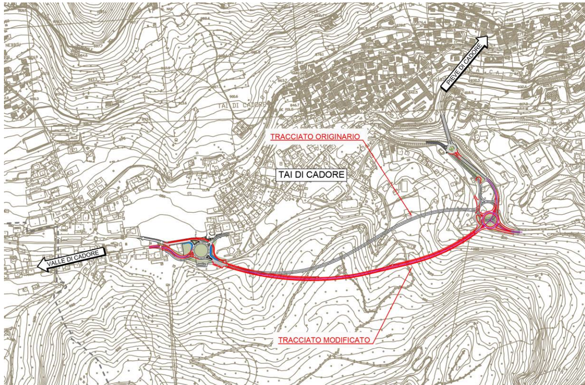
Figura 2- Confronto planimetrie tracciato
