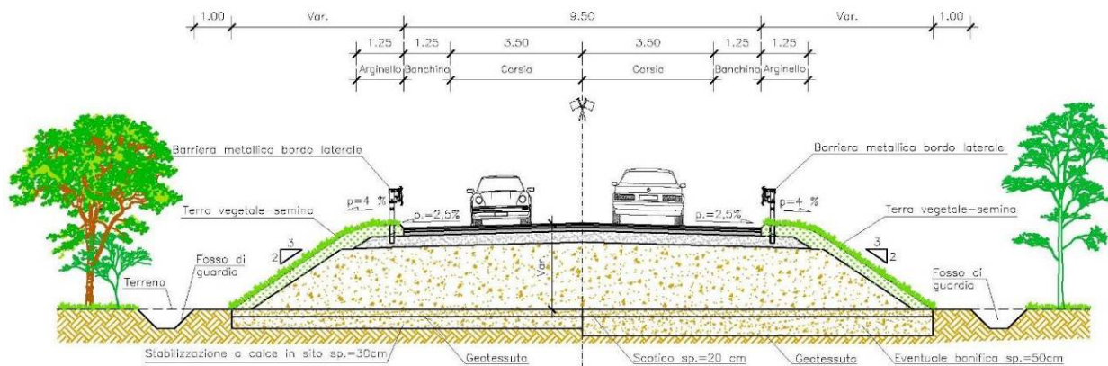
Figura 7 - Sezione tipo C2 in rettilineo attraversamento abitato di Tai di Cadore
