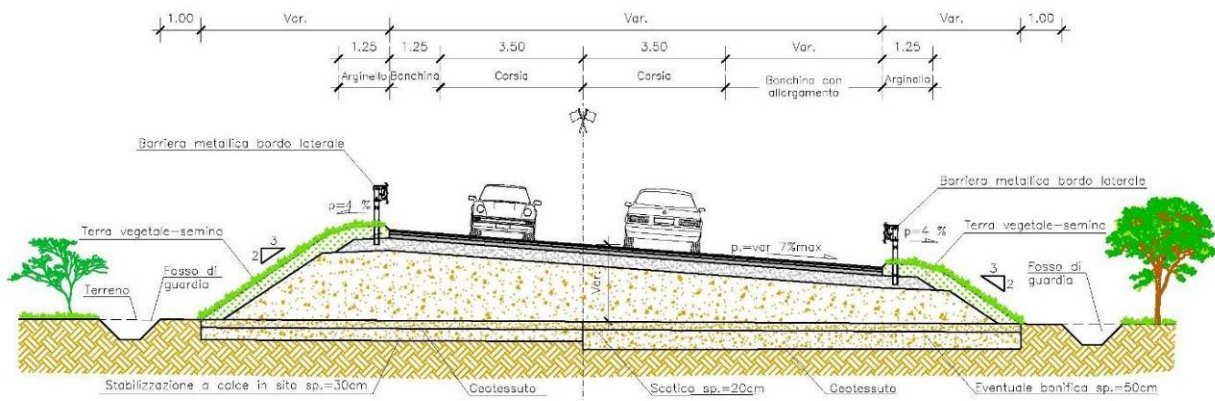
Figura 8 - Sezione tipo C2 in curva attraversamento abitato di Tai di Cadore
