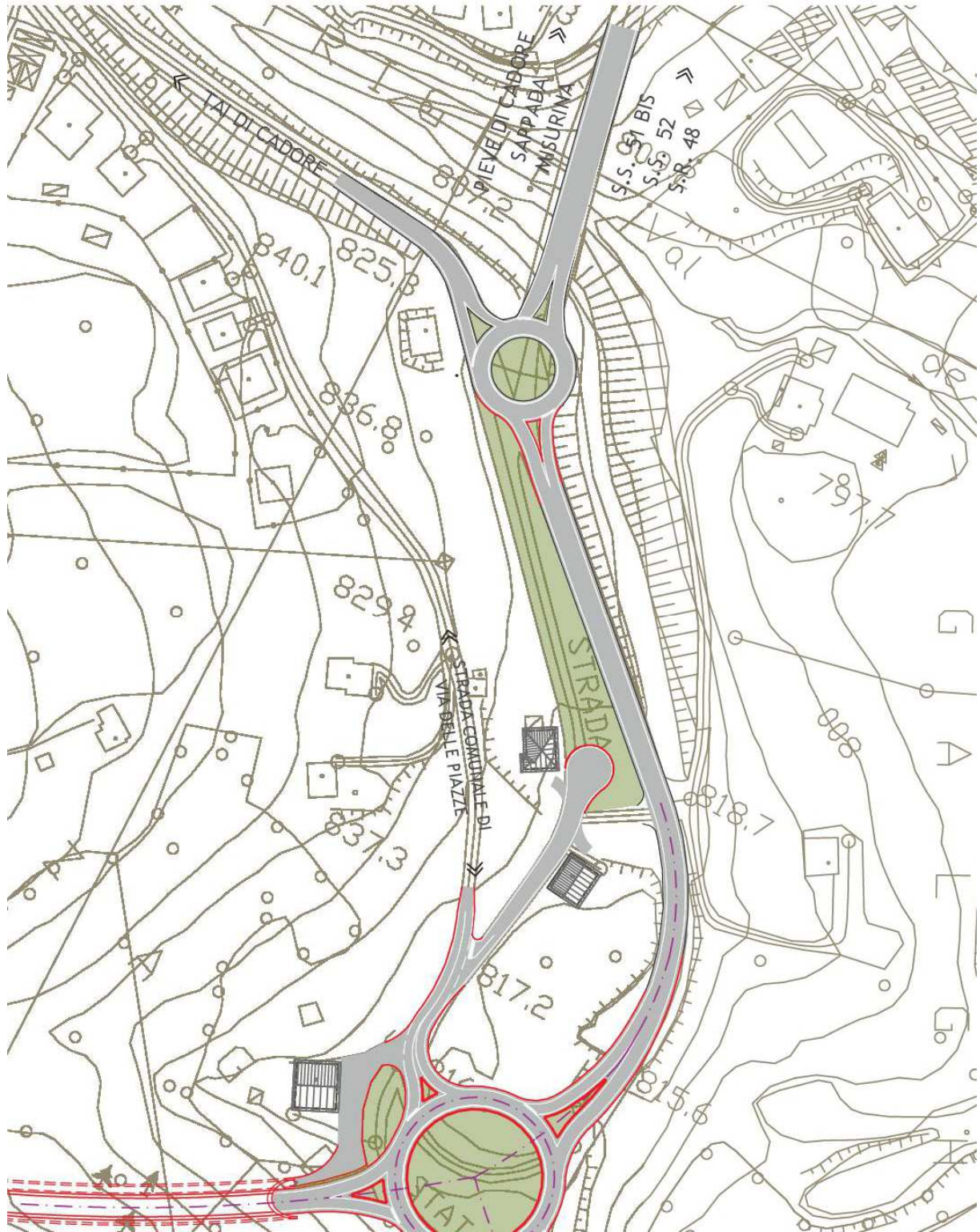
Figura 5 – Piccola rotatoria a nord dello svincolo Est
