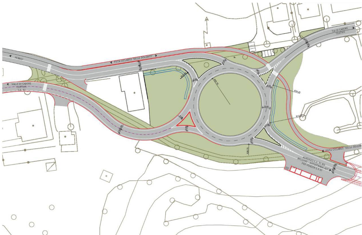
Figura 6 - Svincolo di Tai Ovest
