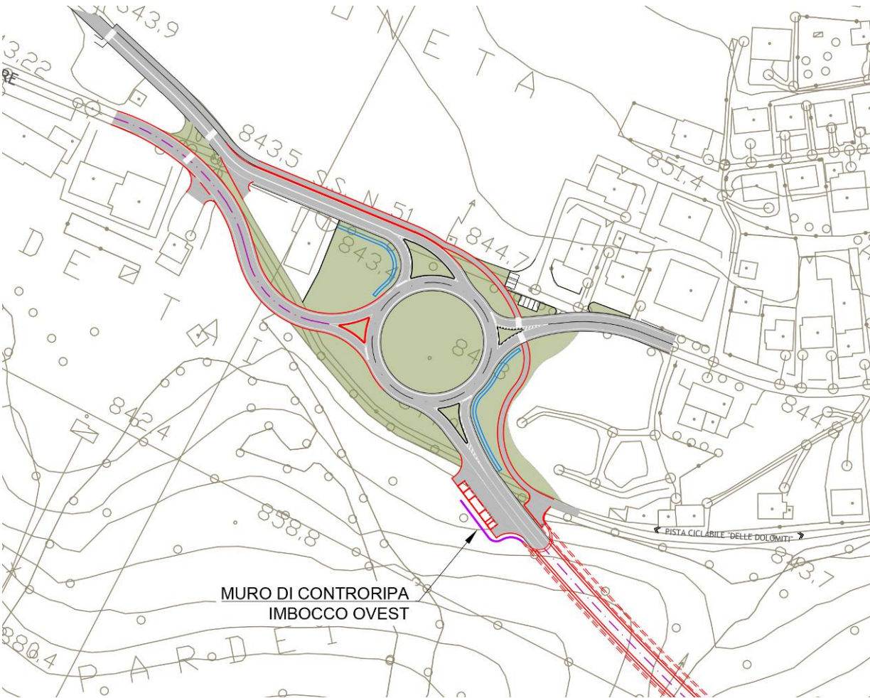
Figura 13 - Muro di controripa zona svincolo Ovest
