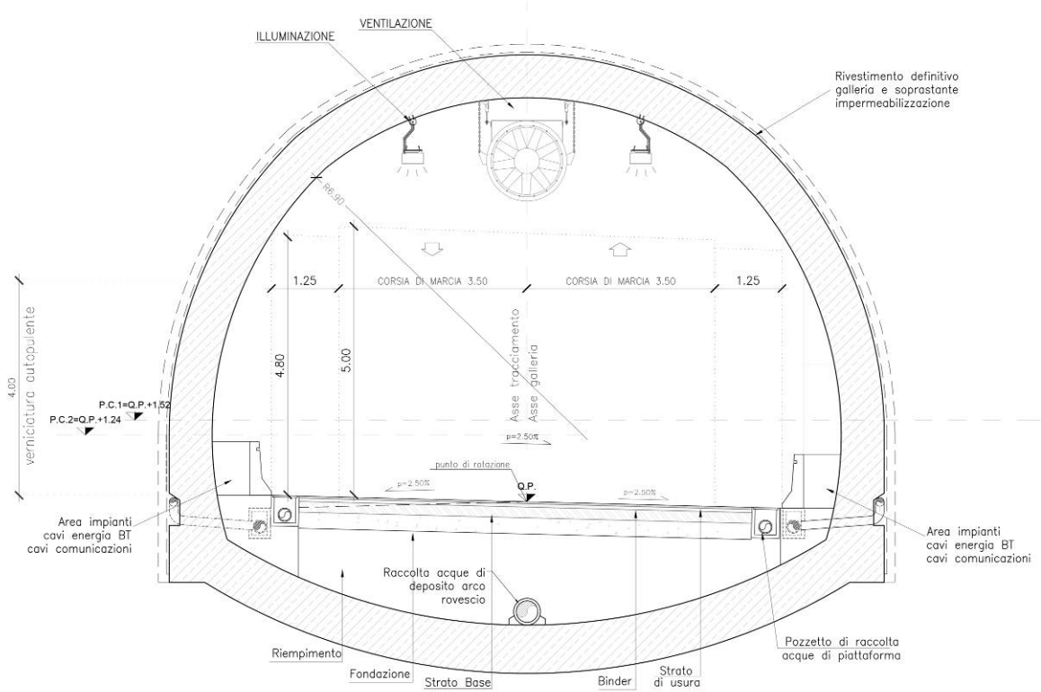
Figura 9 - Sezione corrente della galleria tipo C2 Anas (tratto intermedio senza cunicolo di sicurezza)
