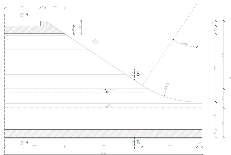
Figura 11 - Imbocco Est ed Ovest a becco di flauto
