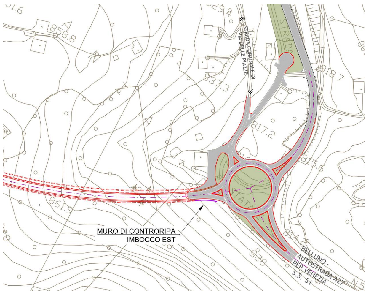
Figura 12 - Muro di controripa zona svincolo Est
