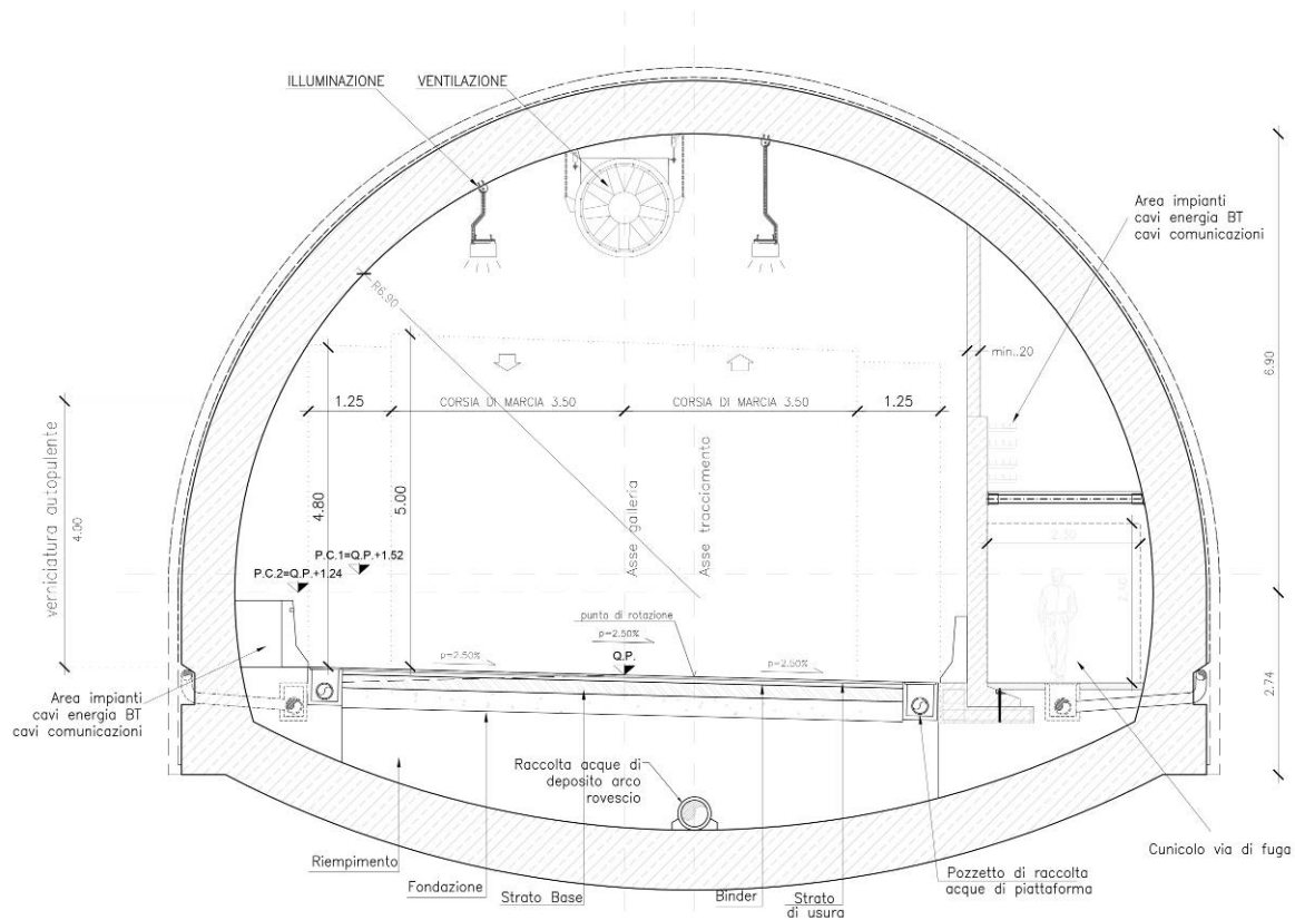
Figura 10 - Sezione corrente della galleria tipo C2 Anas con cunicolo di sicurezza
