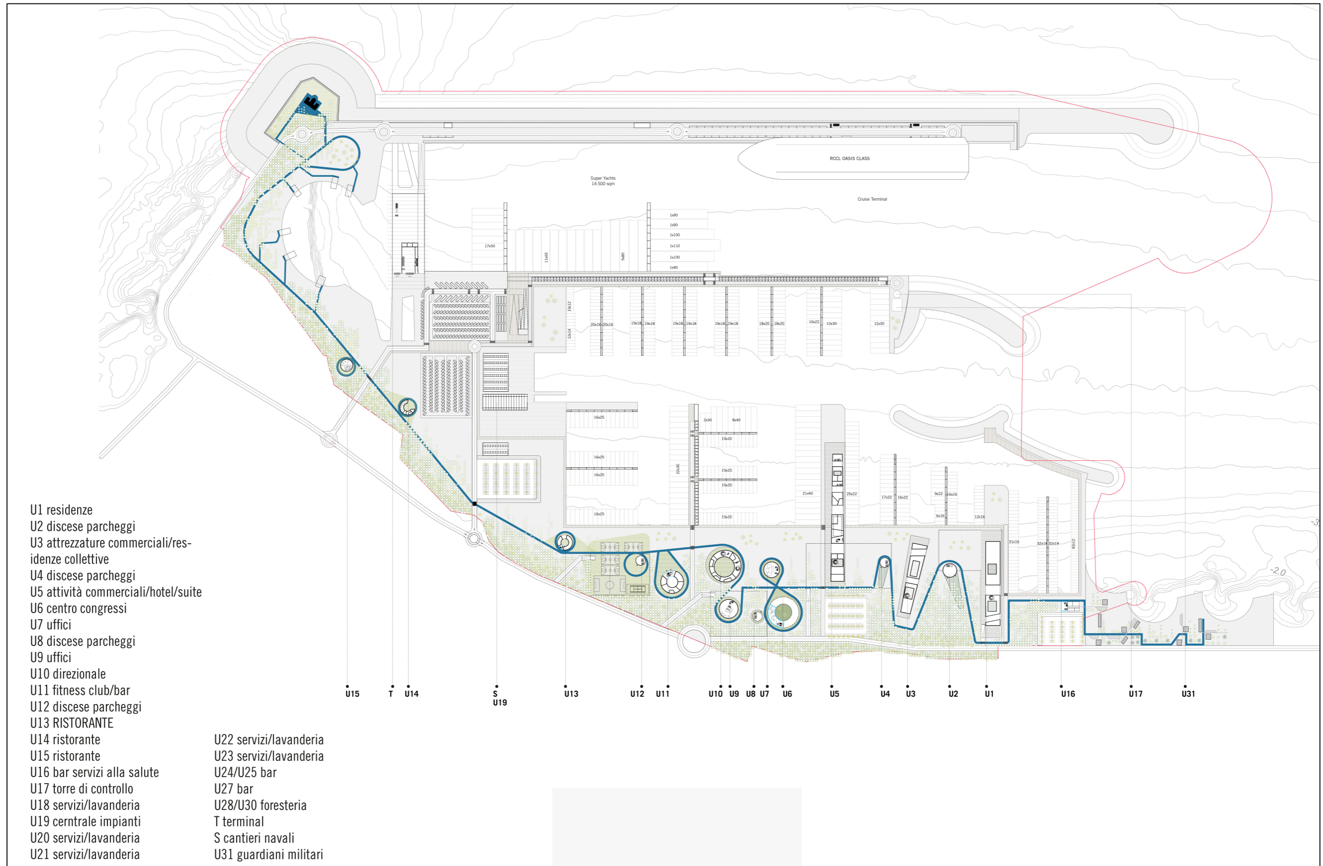
FIGURA 2.2 LAYOUT DI PROGETTO
