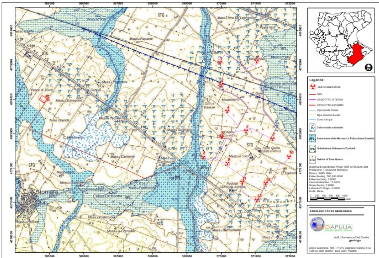
Stralcio tavola DW19045D-V13 – Carta geologica
